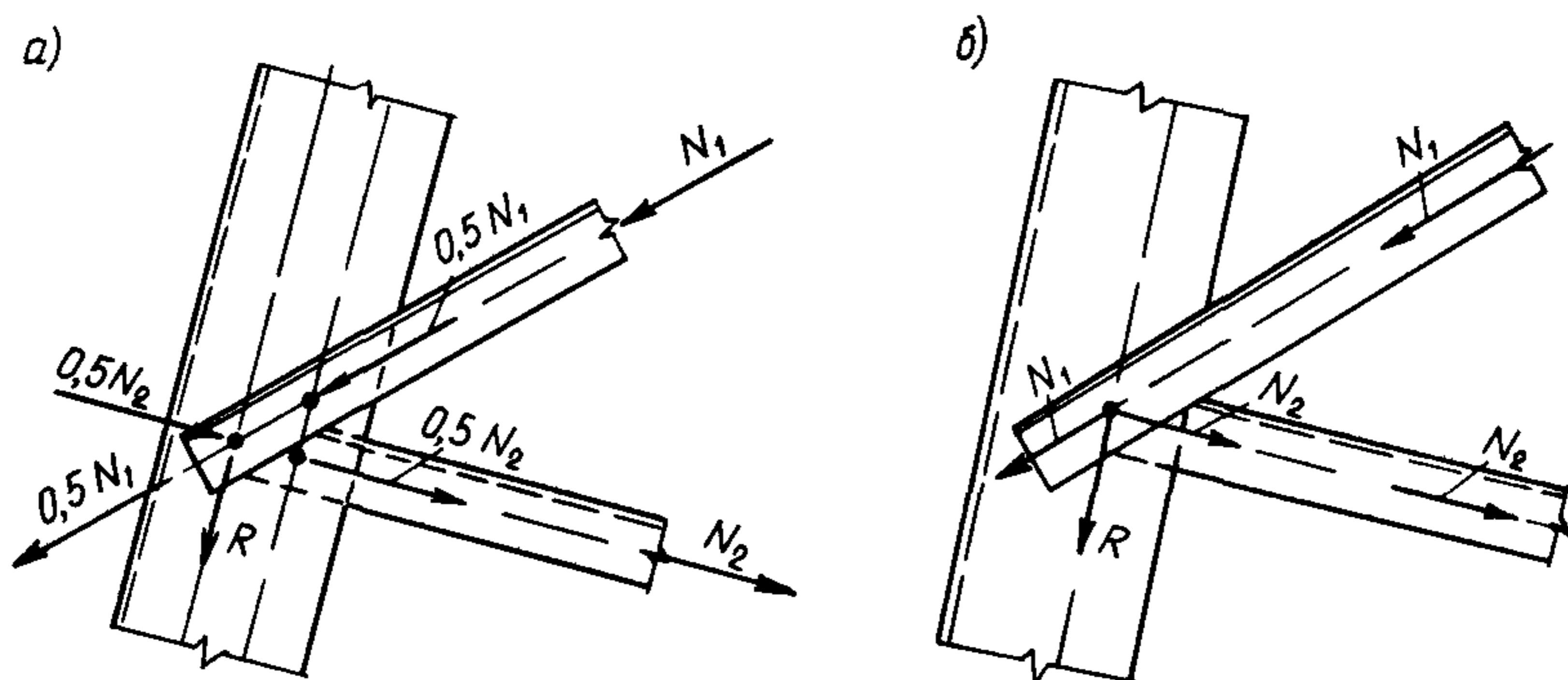
Черт. 17. Схема соединения раскосов с поясом
