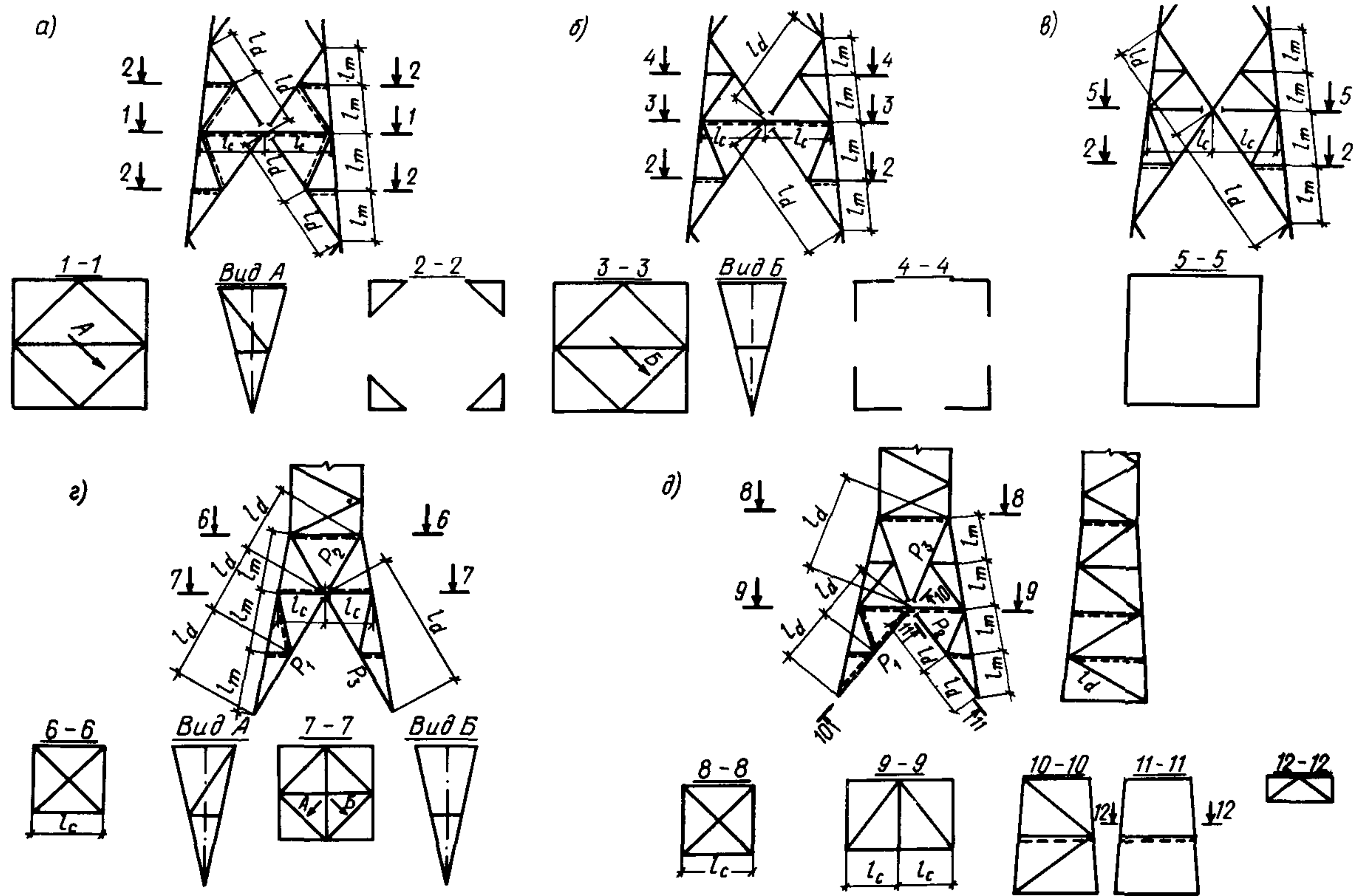
Черт. 2. Схемы шпренгельной решетки
