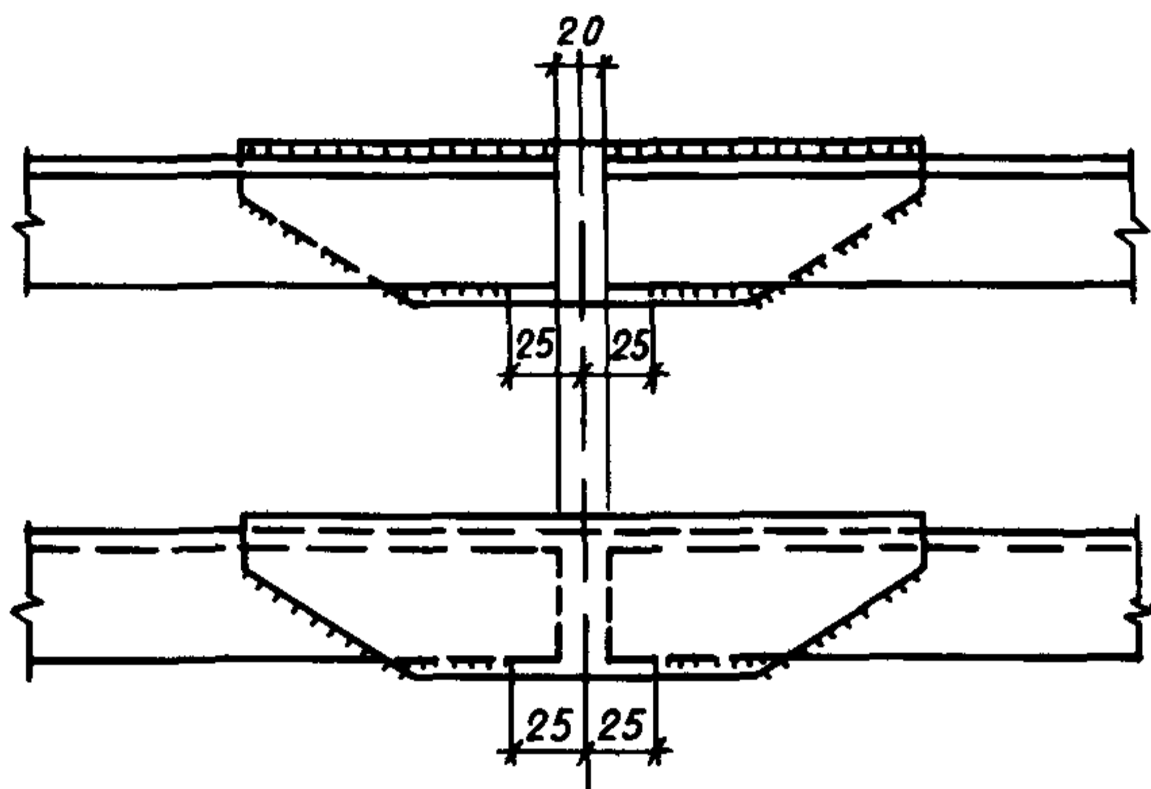
Черт. 19. Сварной стык пояса
