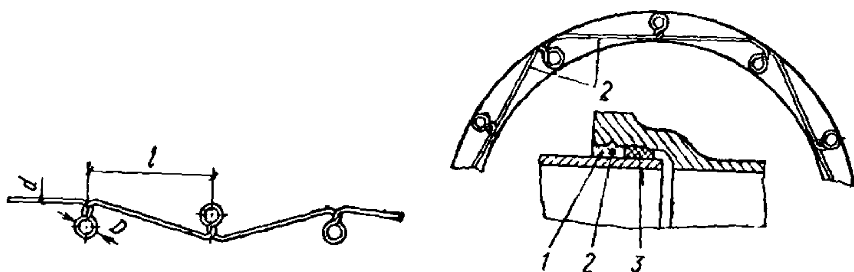
Рис. 38. Проволока для армирования асбестоцемента:
