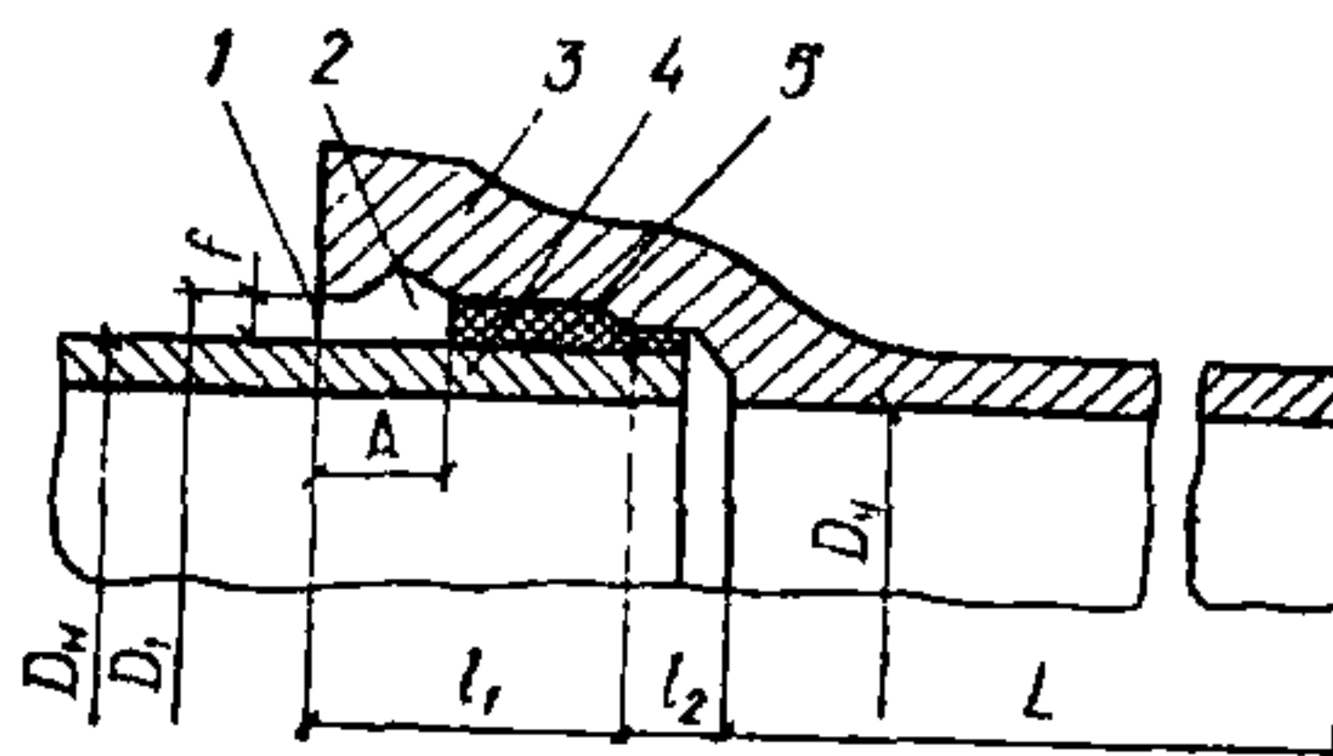
Рис. 29. Раструбное стыковое соединение чугунных напорных труб (ГОСТ 9583—75):
