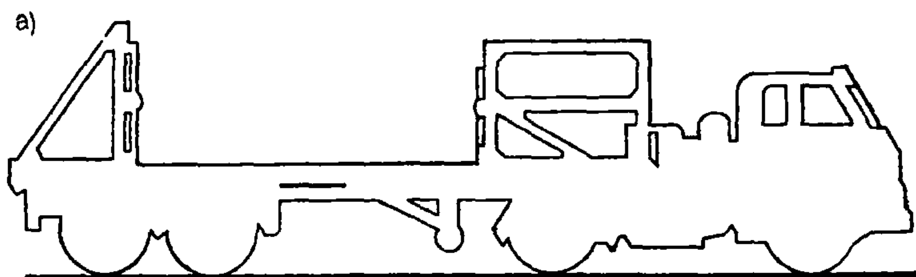
Рис. 6. Расположение полотенец строп-контейнера (а) и схема укладки труб в двух строп-контейнерах в кузов автомобиля (б): 1 — полотенце; 2 — замок; 3 — пластина с фиксатором; 4 — прокладка
