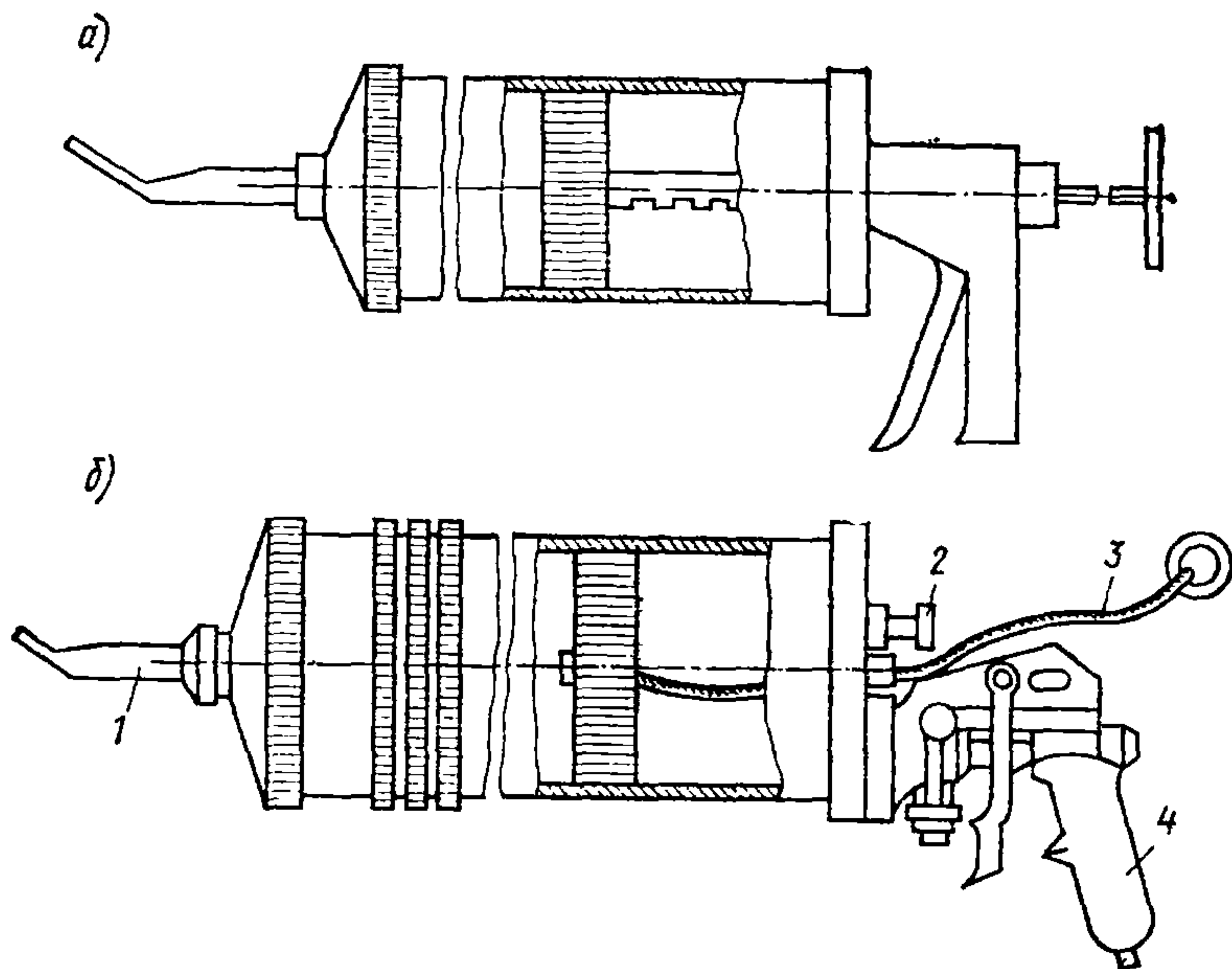
Рис. 40. Шприцы для герметизации стыковых соединений трубопроводов:
