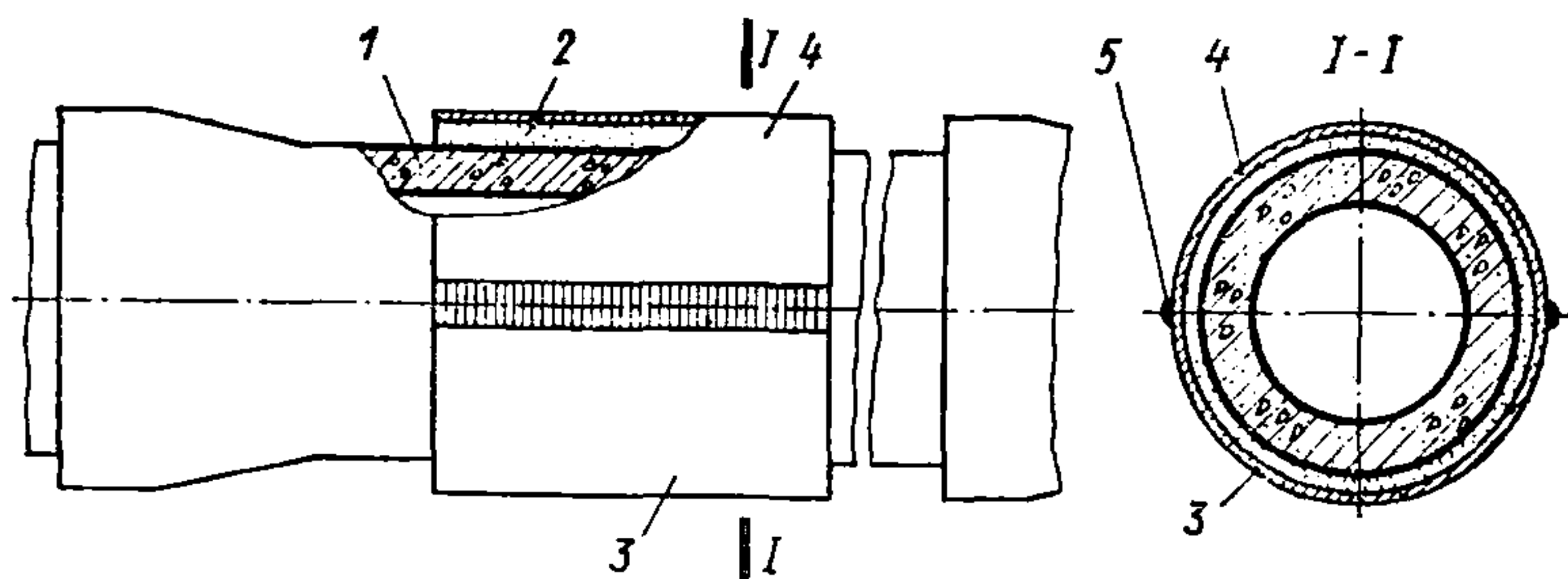
Рис. 62. Ремонт железобетонной трубы наложением стальной разрезной муфты:
