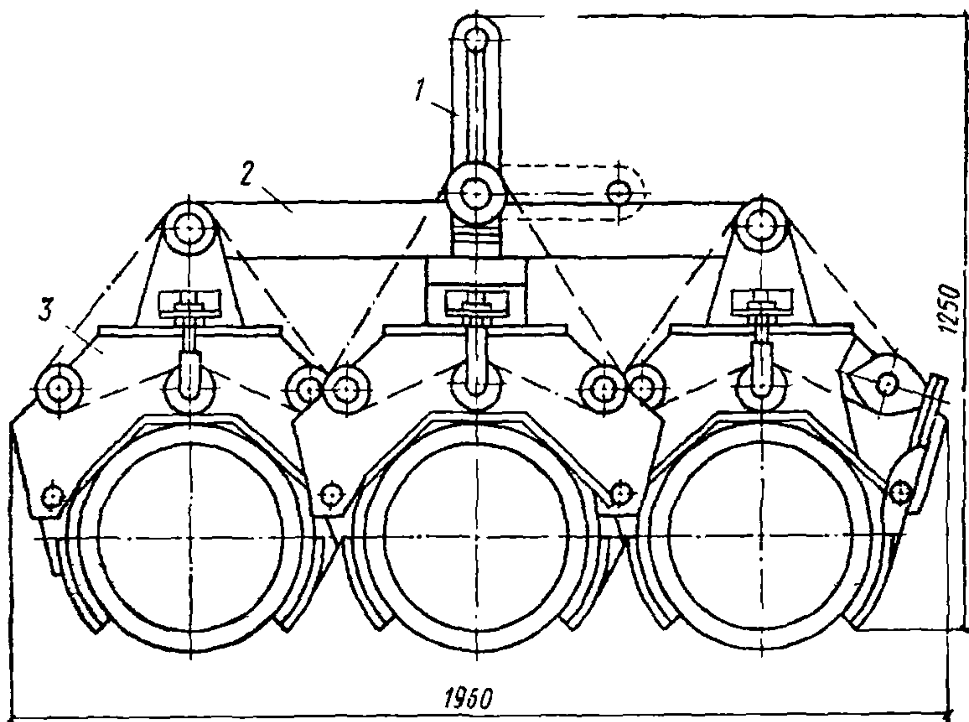
Рис. 4. Траверса ГТА-0510 для труб ТНСП:
