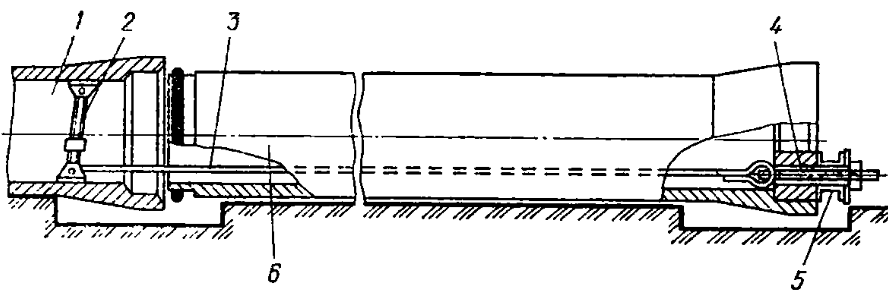
Рис. 17. Монтаж трубопровода с помощью натяжного приспособления, устанавливаемого внутри трубы:
