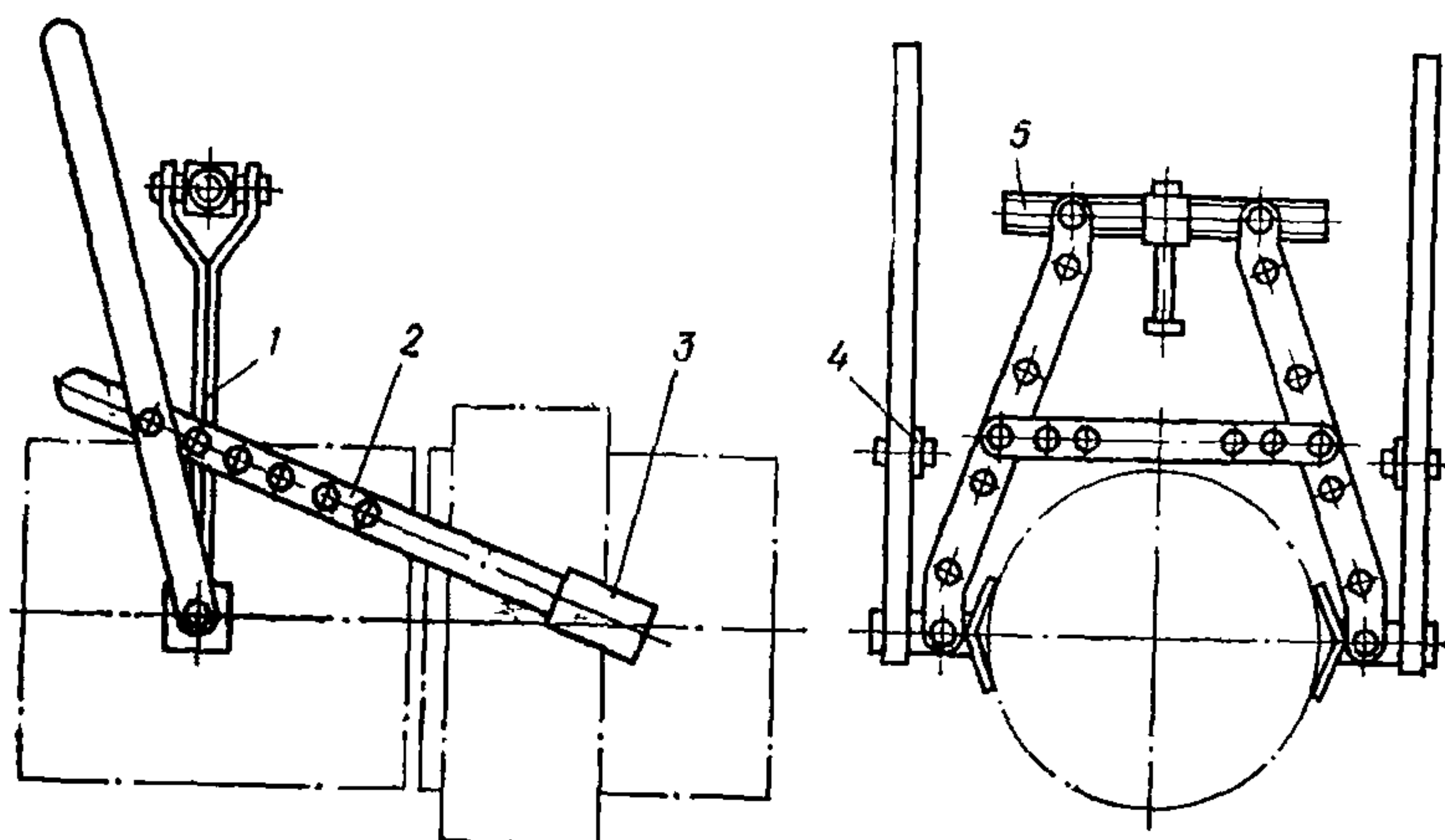
Рис. 50. Рычажный домкрат:
