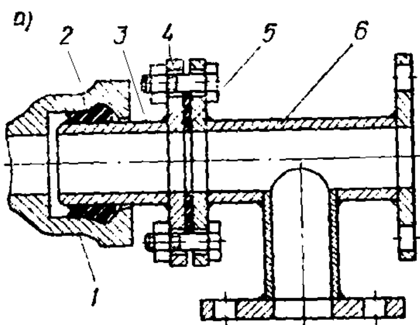
Рис. 42. Присоединение фланцевой части:
