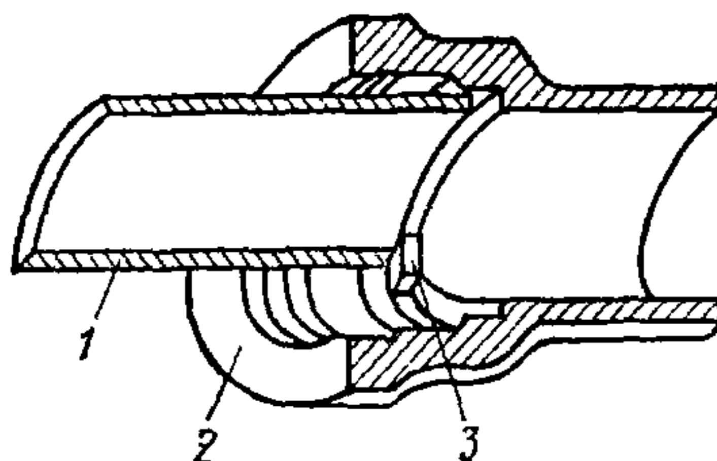
Рис. 34. Положение вкладыша-ограничителя в трубе:
