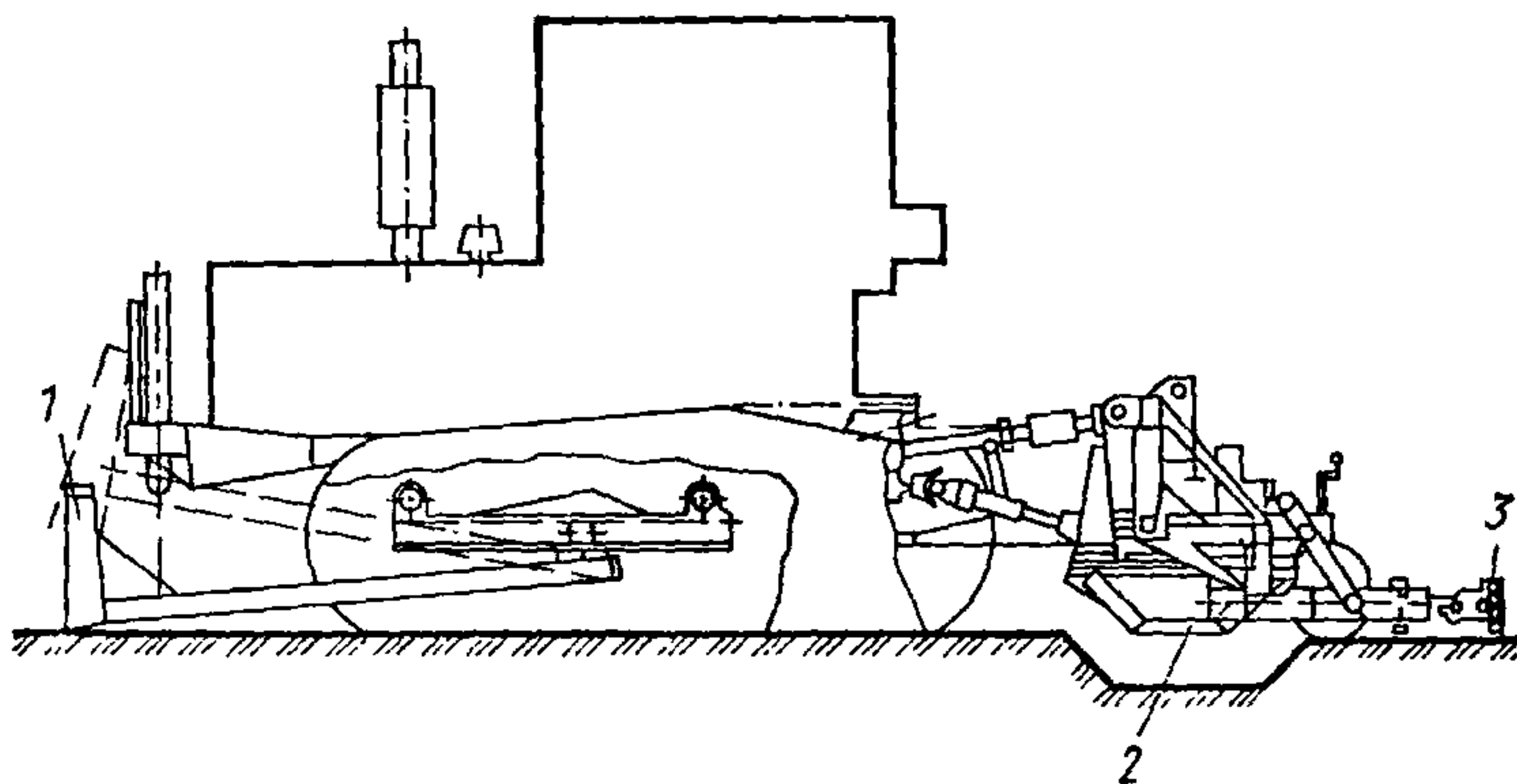
Рис. 10. Навесное сменное оборудование к трактору Т-54 В-С2 для планировки дна траншей, разработки профилированного грунтового основания под трубопроводы и стыковки труб ТНСП диаметром 500—1000 мм:
