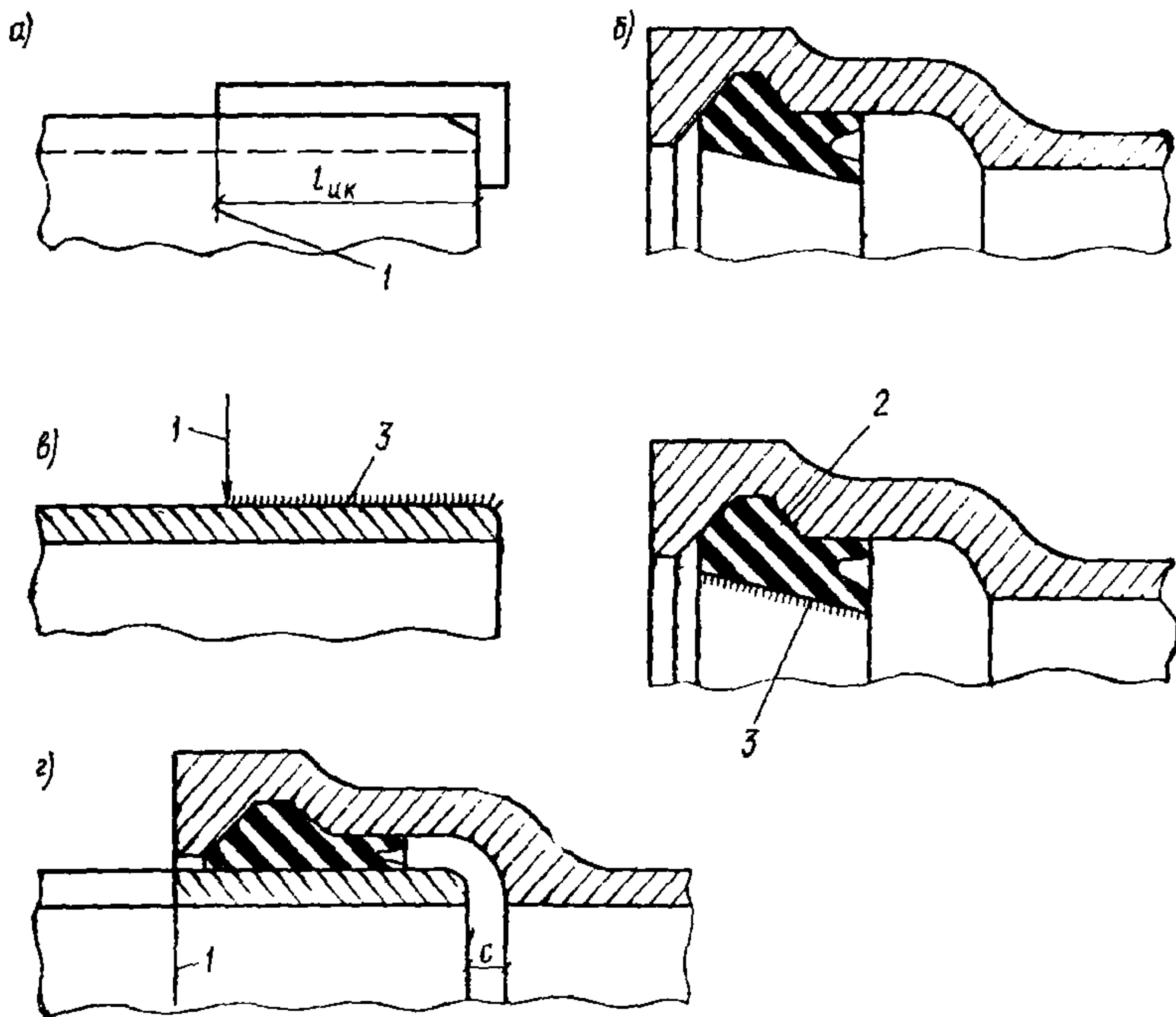
Рис. 31. Порядок монтажа трубопроводов из чугунных труб со стыковым соединением на резиновой манжете:
