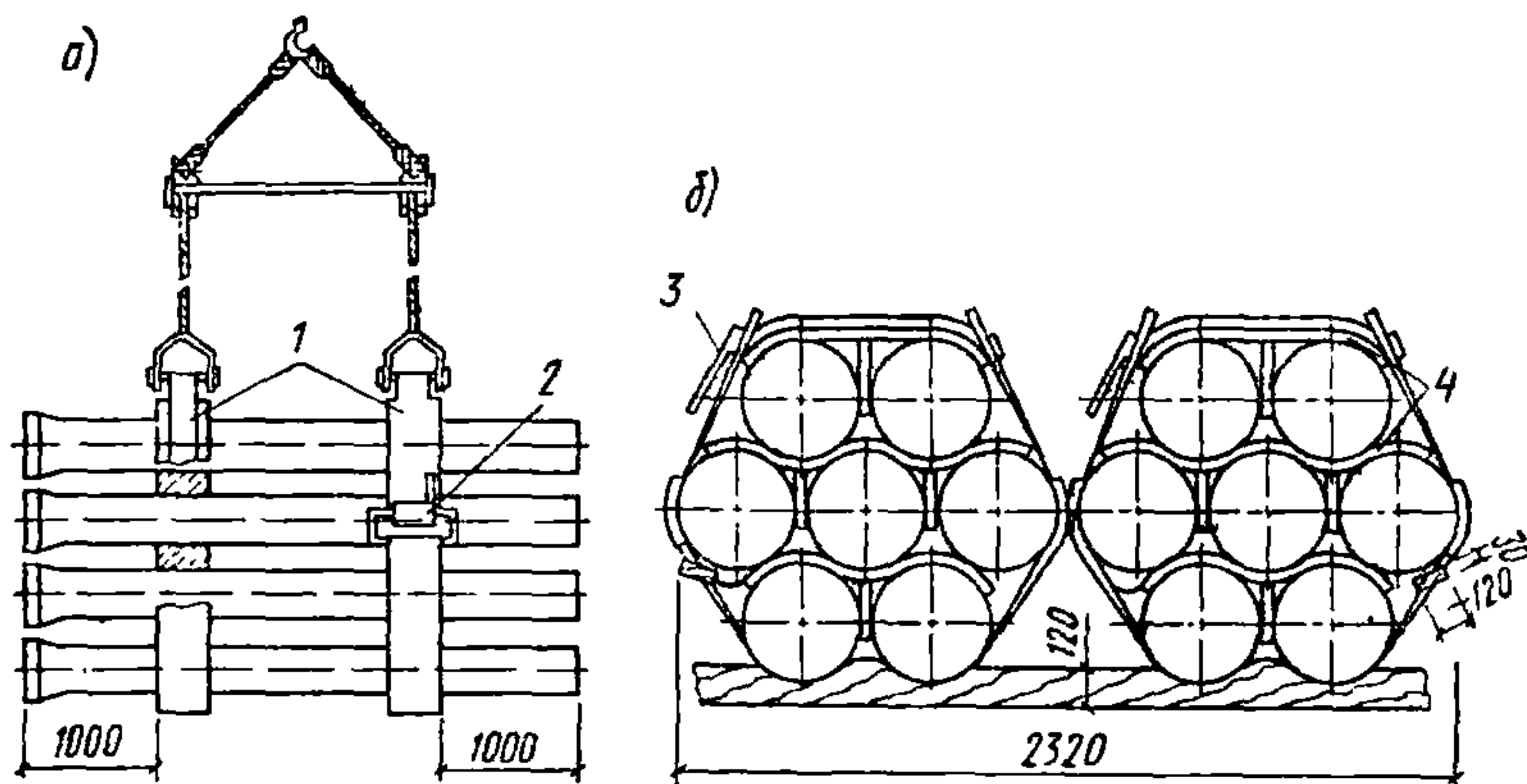
Рис. 6. Расположение полотенец строп-контейнера (а) и схема укладки труб в двух строп-контейнерах в кузов автомобиля (б): 1 — полотенце; 2 — замок; 3 — пластина с фиксатором; 4 — прокладка
