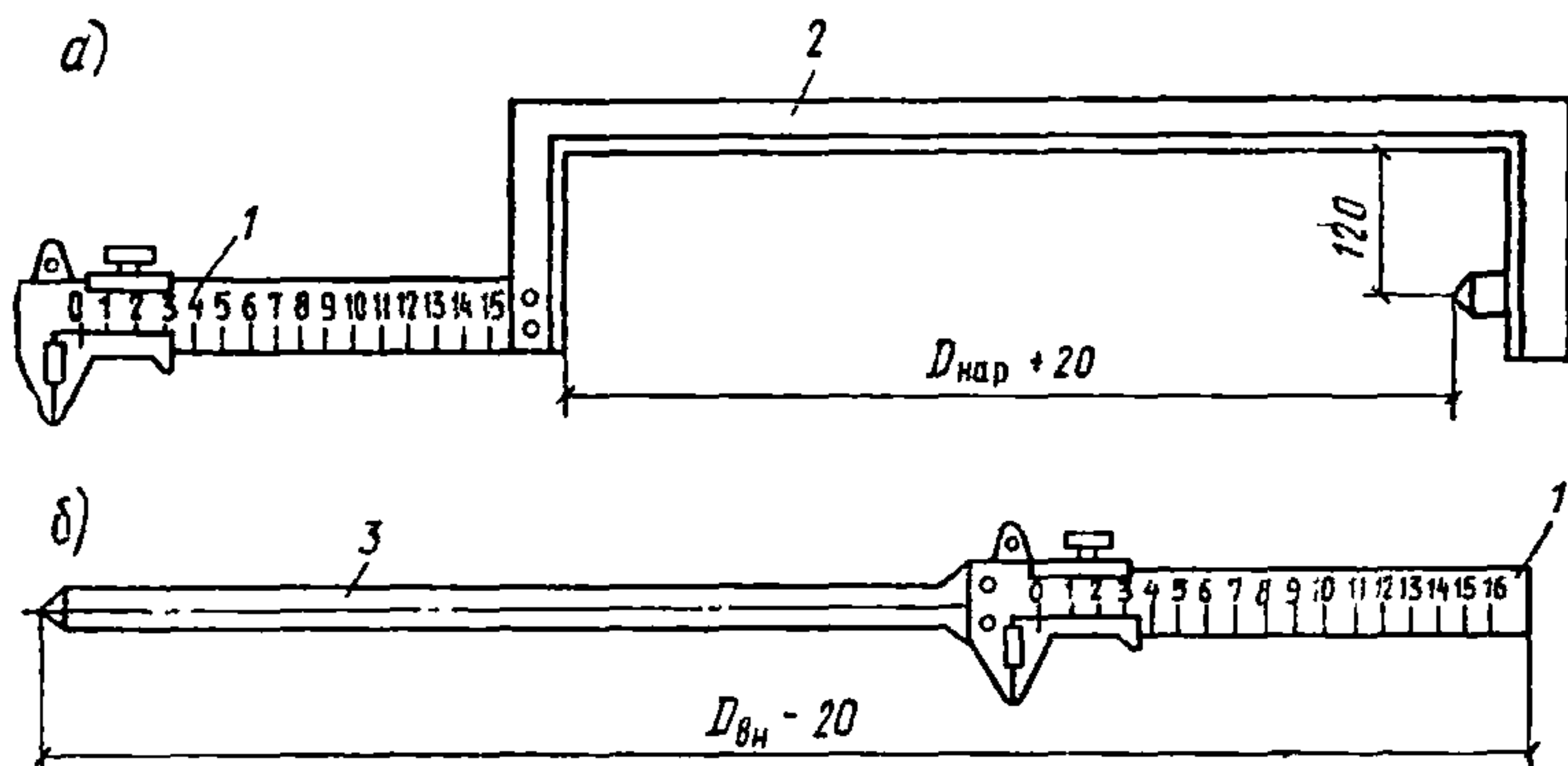
Рис. 1. Измерительные приспособления с использованием штангенциркулей: а — скоба для контроля наружных диаметров труб; б — внутромер; 1 — штангенциркуль; 2 — металлическая скоба; 3 — удлинитель
