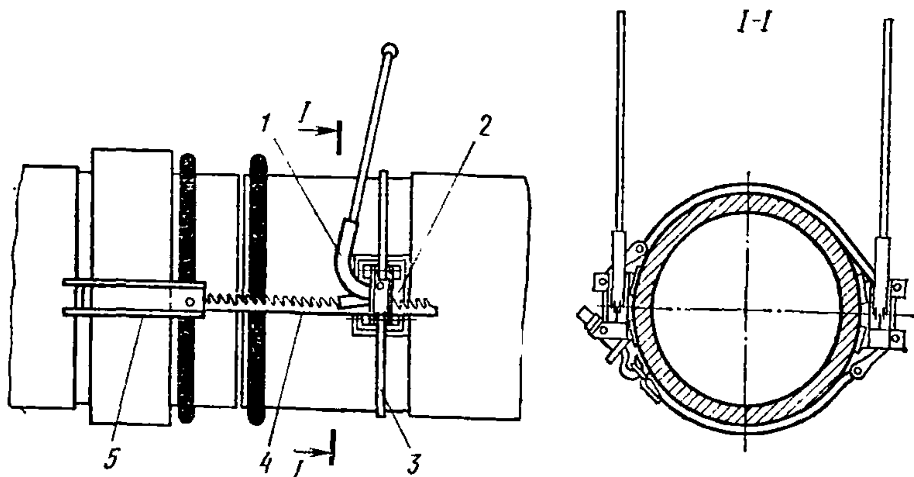
Рис. 51. Рычажно-реечное натяжное приспособление: 1 — рычаг; 2 — упорный башмак; 3 — комут; 4 — рейка; 5 — захват
