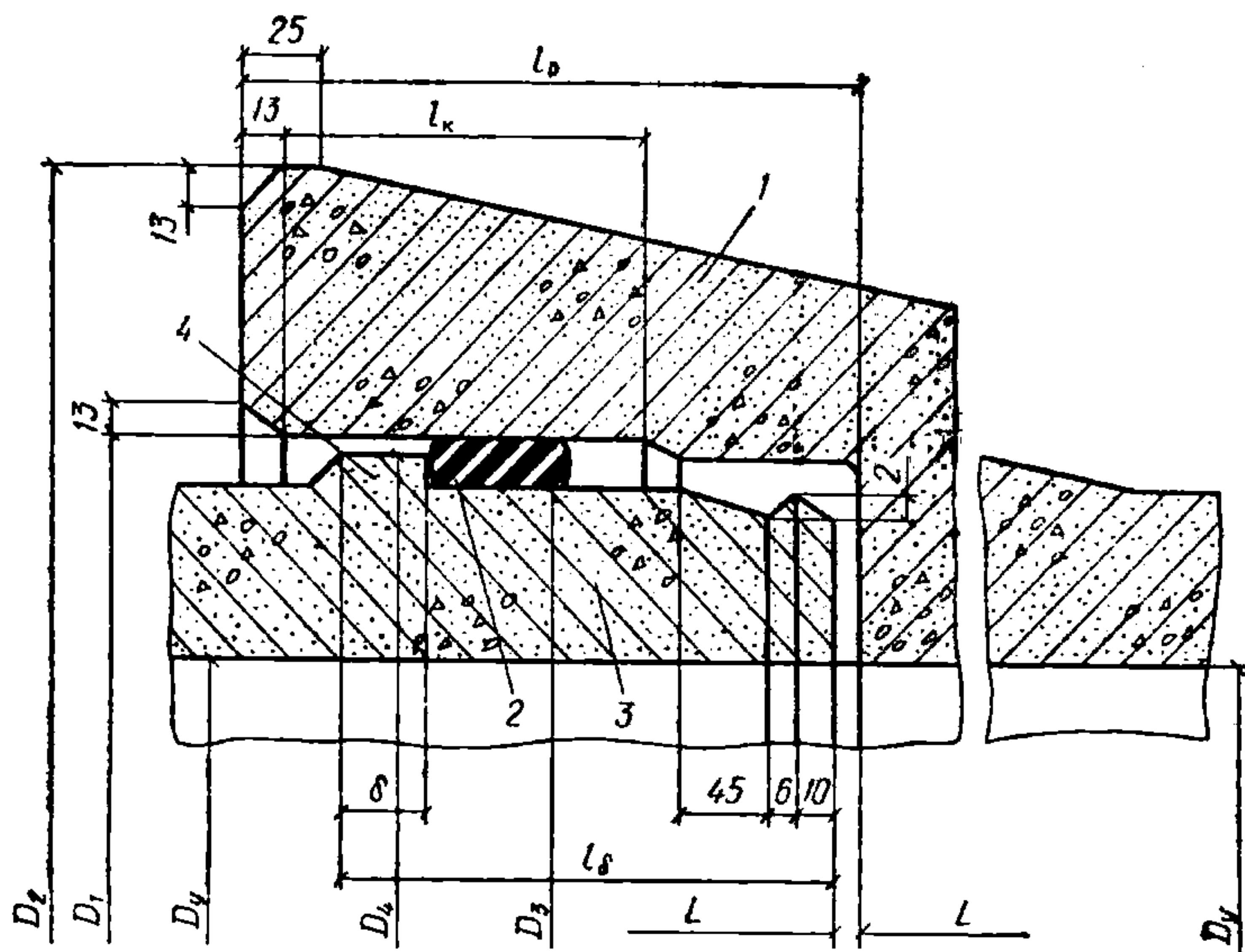
Рис. 11. Раструбное стыковое соединение железобетонных напорных виброгидропрессованных труб (ГОСТ 12586.0—83):
