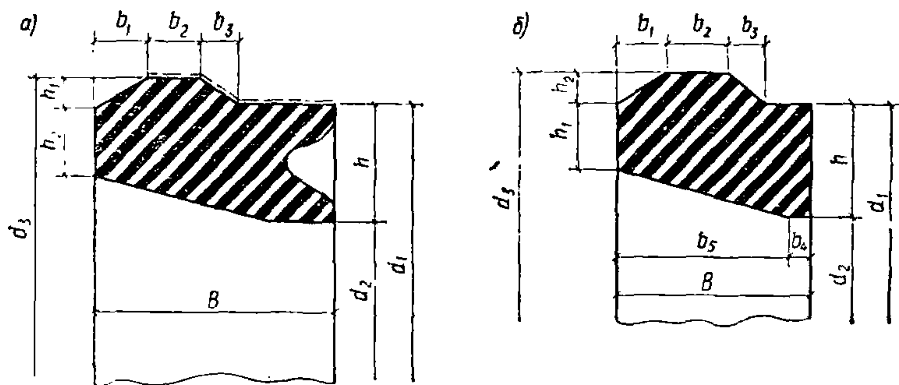
Рис. 30. Резиновая уплотнительная манжета (ТУ 38.105895—75): а — манжета с «ласточкиным хвостом» Б-1 и Б-2 для труб по ТУ 14-3-1247-83; б — манжета укороченная 1-Б-1 и 1-Б-2 и универсальная облегченная БХ для труб по ТУ 14-3-1247-83
