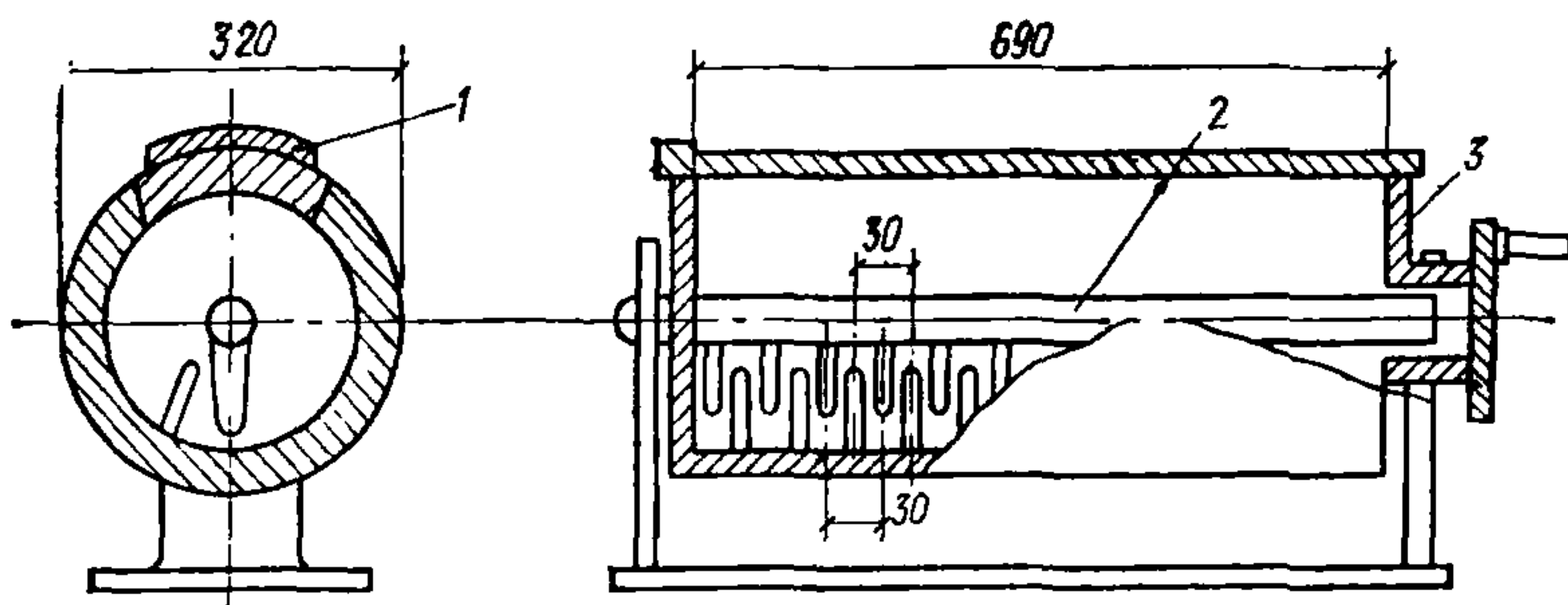
Рис. 38. Смесительный барабан (размеры в миллиметрах): 1 — крышка; 2 — неподвижный вал с лопастями; 3 — вращающийся барабан
