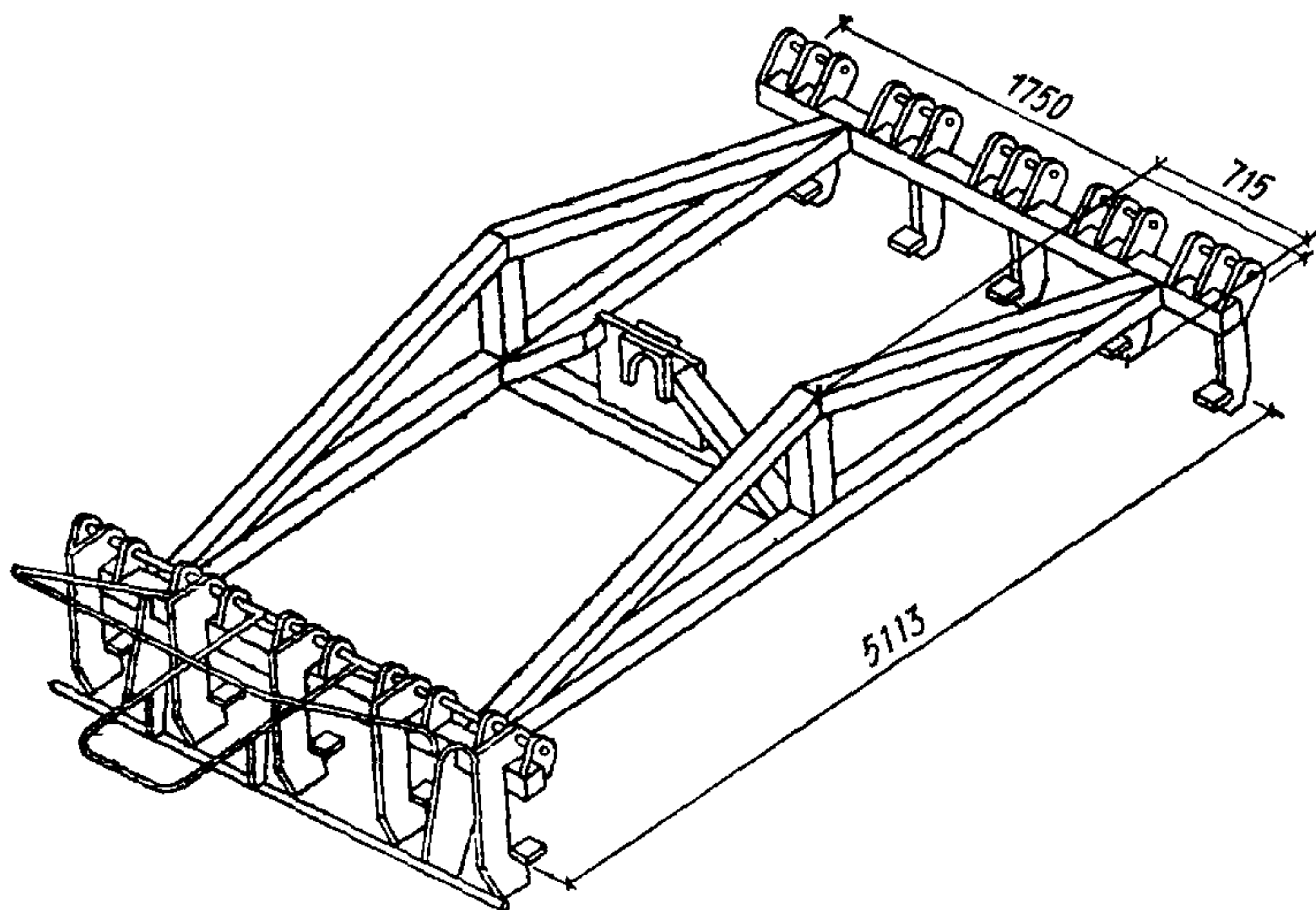
Рис. 5. Траверса ГРТ-0305 для ТНСП-25-40
