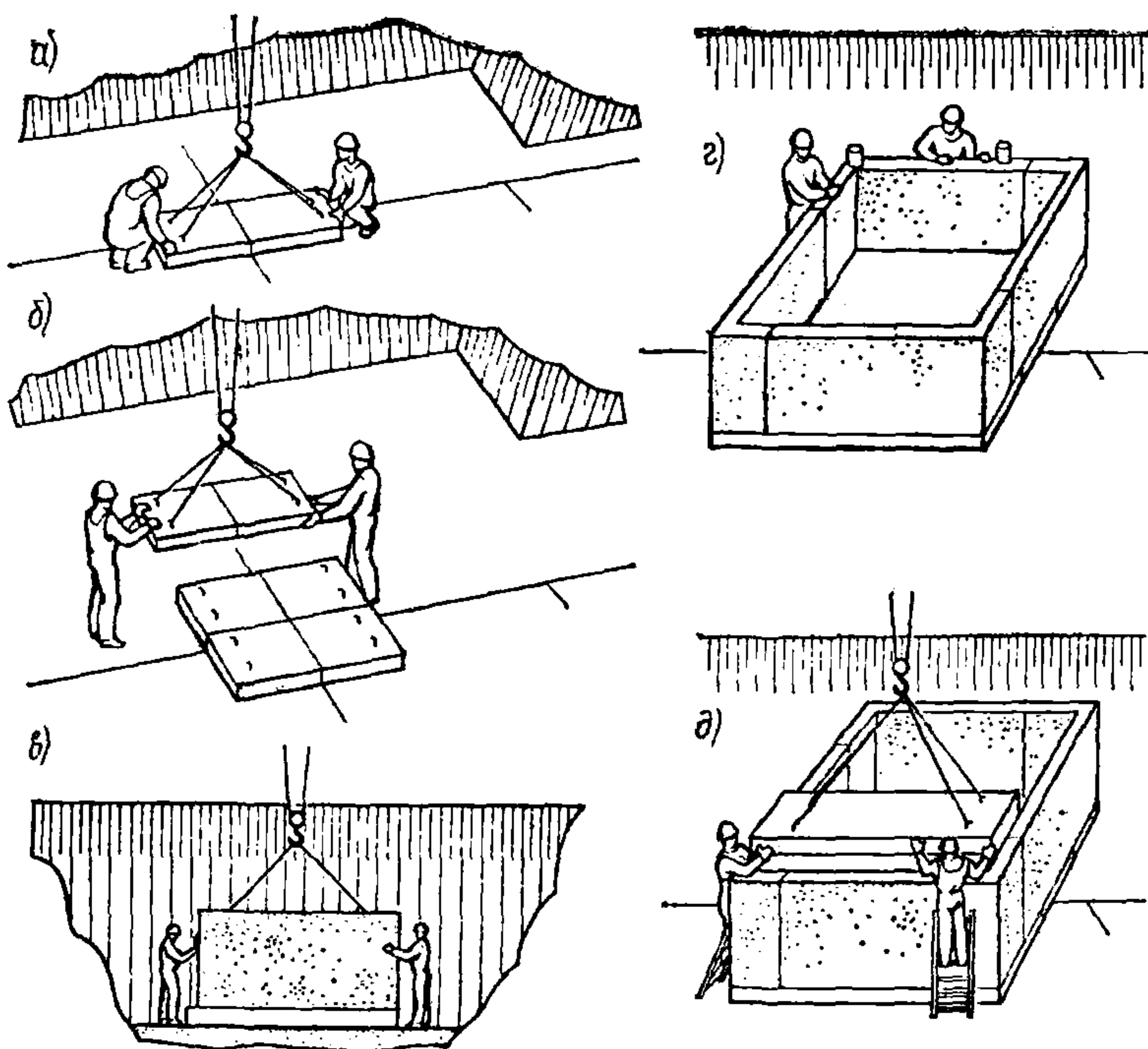
Рис. 56. Монтаж полносборных железобетонных камер. а, б — укладка плит основания; в, г — монтаж Г-образных блоков; д — монтаж плит перекрытия
