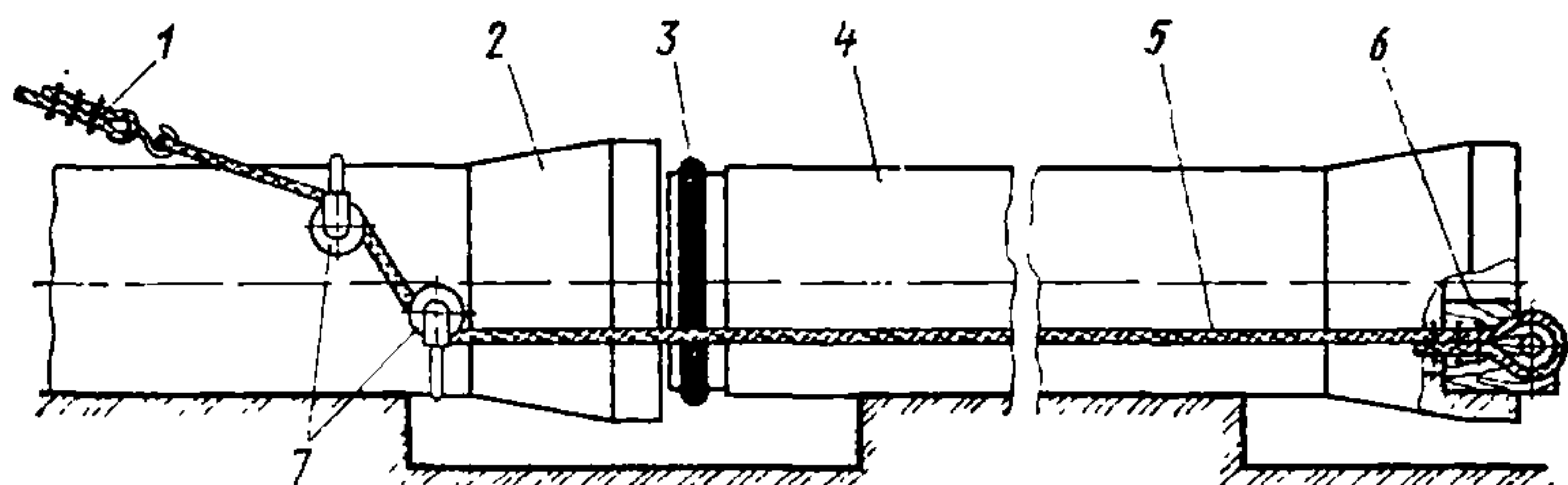
Рис. 20. Монтаж трубопровода с помощью шестереночной лебедки: 1 — трос лебедки; 2 — уложенный трубопровод; 3 — резиновое кольцо; 4 — укладываемая труба; 5 — переносной натяжной трос; 6 — упорный брус; 7 — блоки
