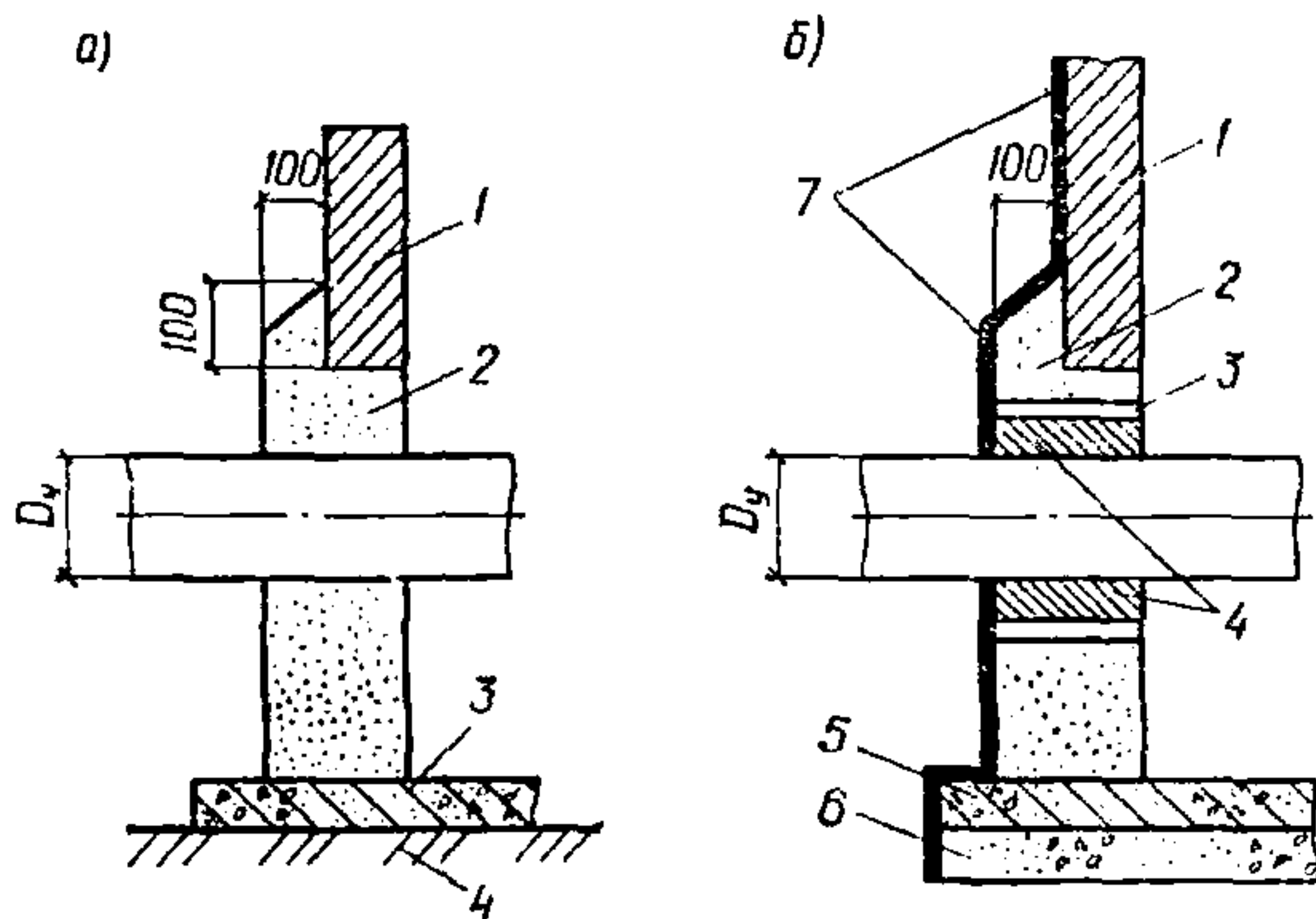
Рис. 54. Детали заделки труб в стенках колодцев:
