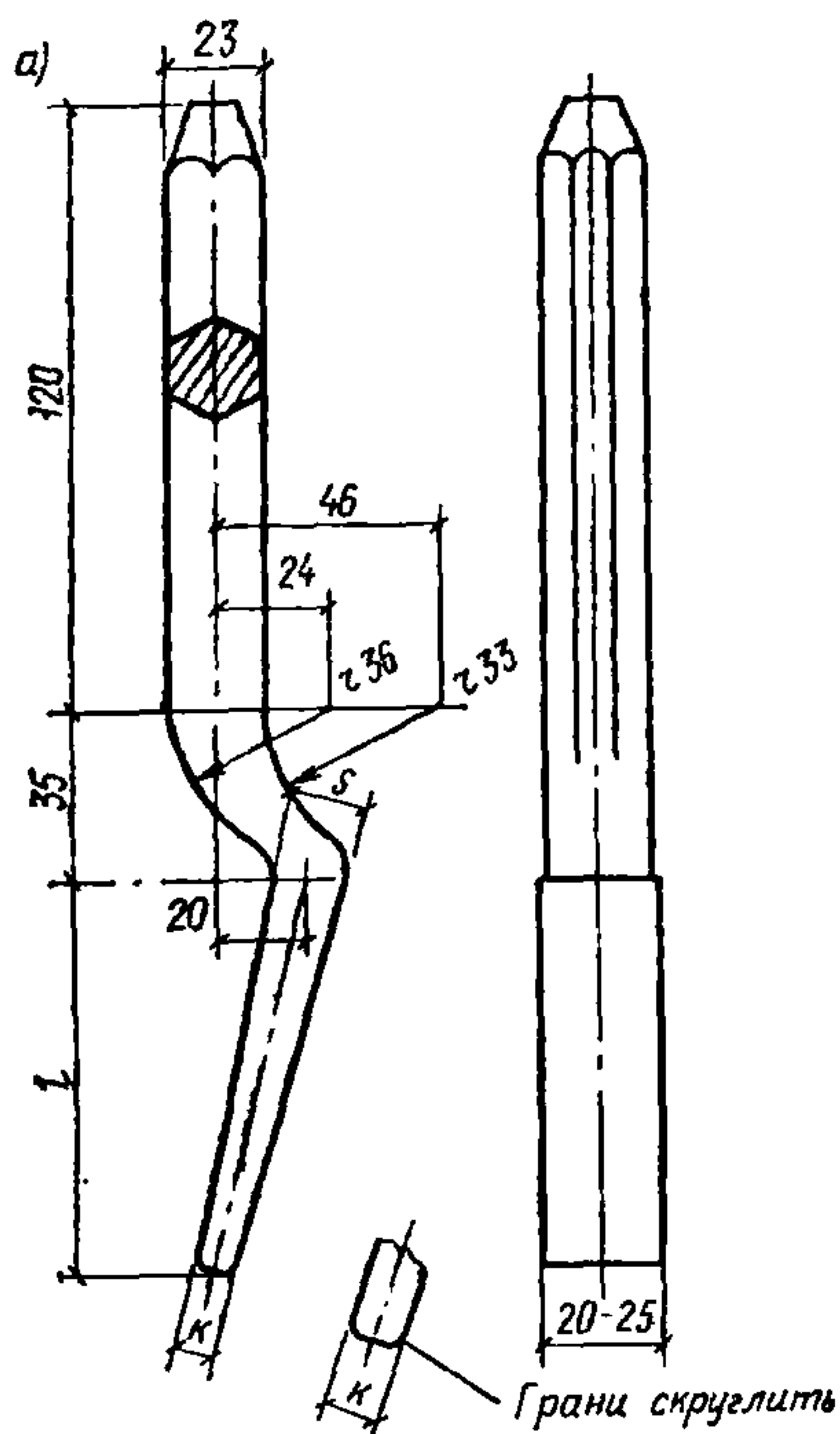
Рис. 35. Конопатки и чеканки: а — ручные; б — кузнечного типа
