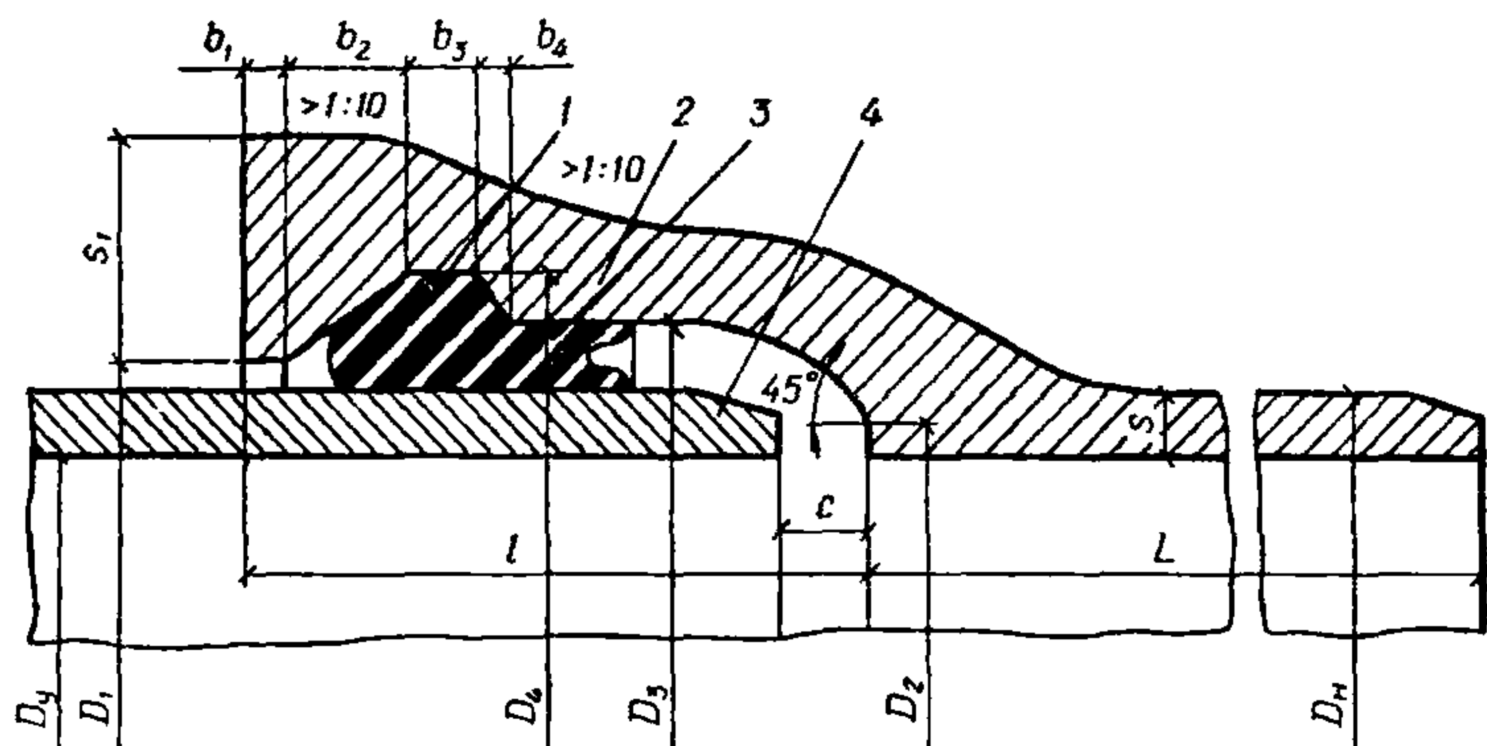
Рис. 28. Раструбное соединение чугунных напорных труб (ТУ 14-3-1247-83): 1 — трапецевидный кольцевой паз; 2 — раструб; 3 — резиновая уплотнительная манжета; 4 — гладкий конец с фаской
