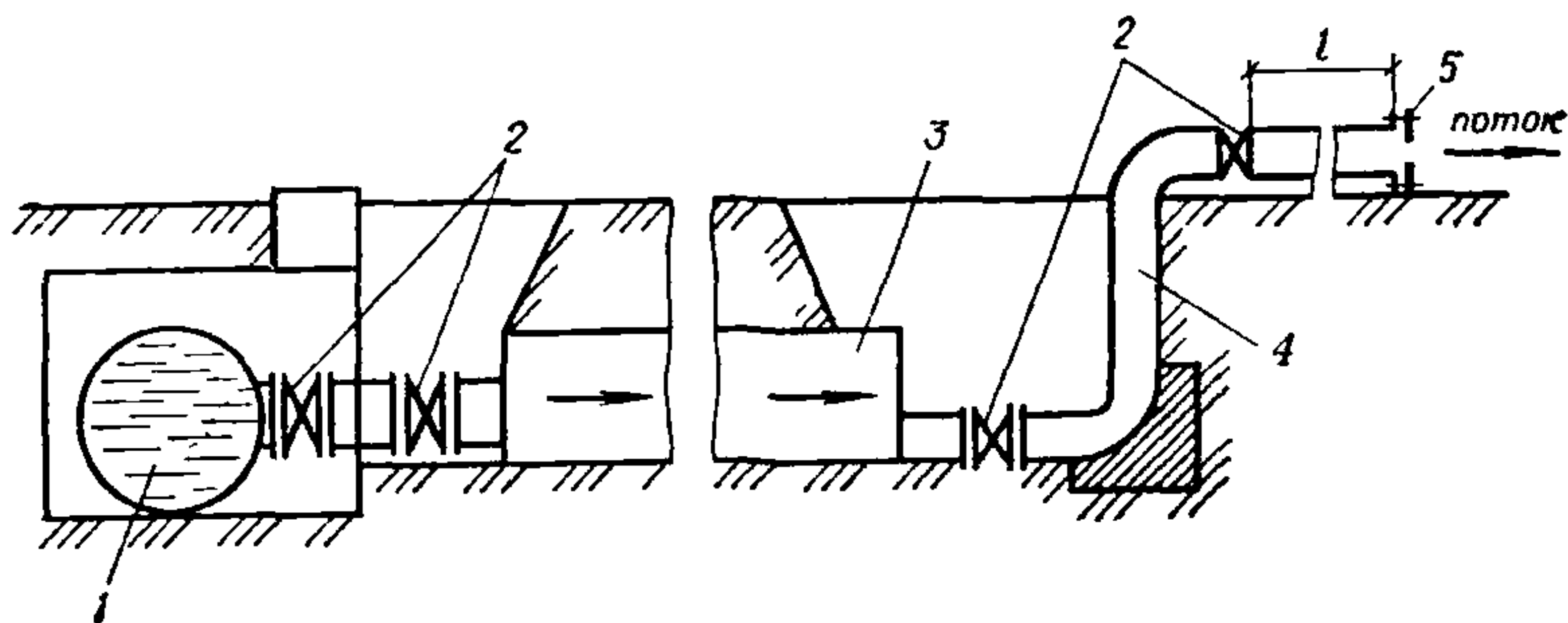
Рис. 1. Схема установки временной диафрагмы для учета воды при промывке трубопроводов
