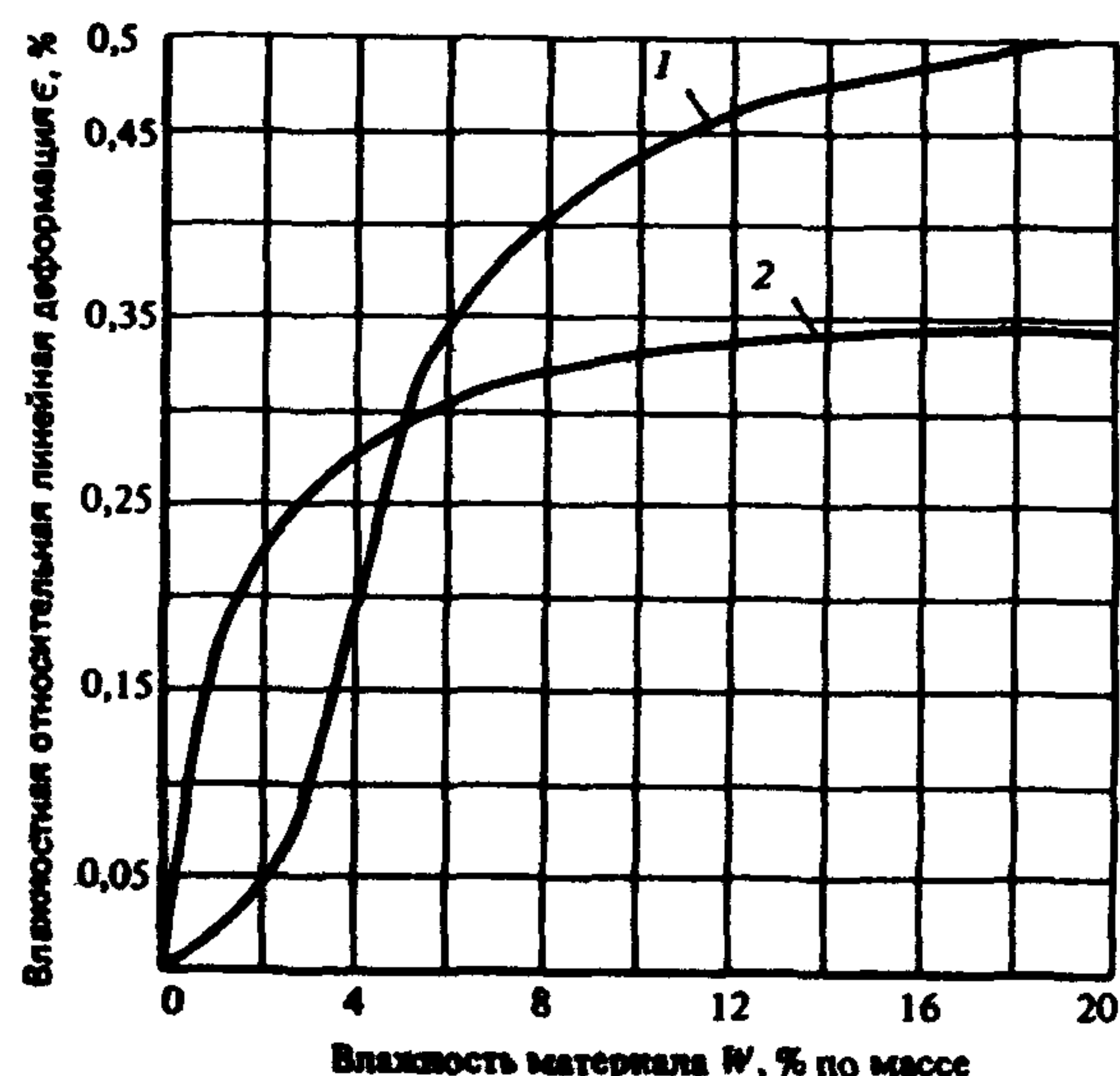
Черт. 1 Зависимость влажностных относительных линейных деформаций \epsilon листового 1 и экструзионного 2 асбестоцементов от их влажности W
