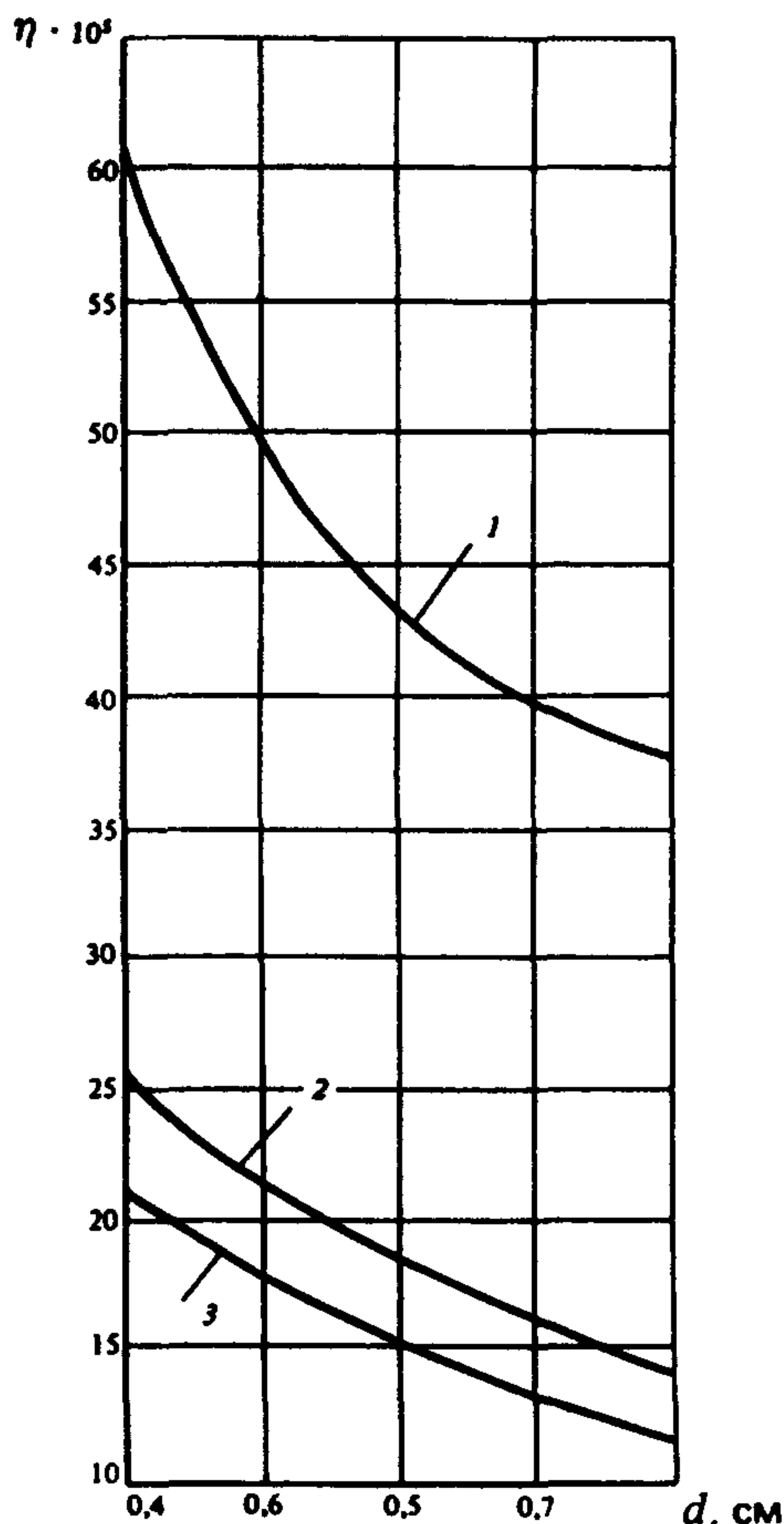
Черт. 3 График для определения коэффициента \eta для плит и панелей с деревянным 1, алюминиевым 2 и стальным 3 каркасами
