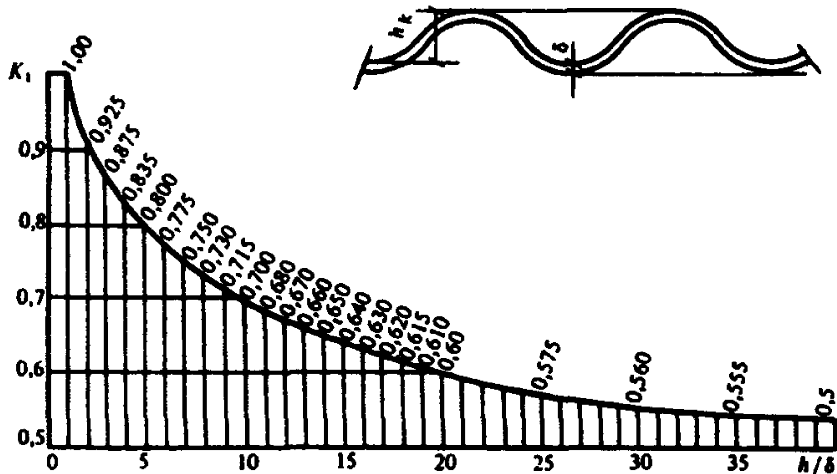
Черт. 7. График для определения коэффициента K_1
