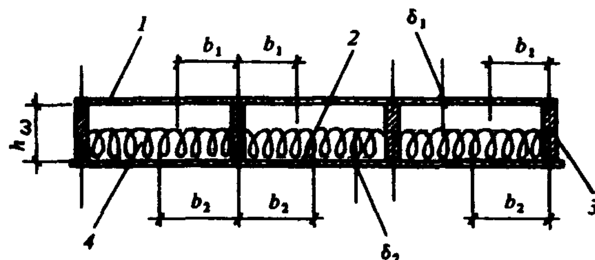
Черт. 2 Поперечное сечение каркасной плиты 1, 2 — асбестоцементные обшивки, 3 — элементы каркаса плиты, 4 — утеплитель
