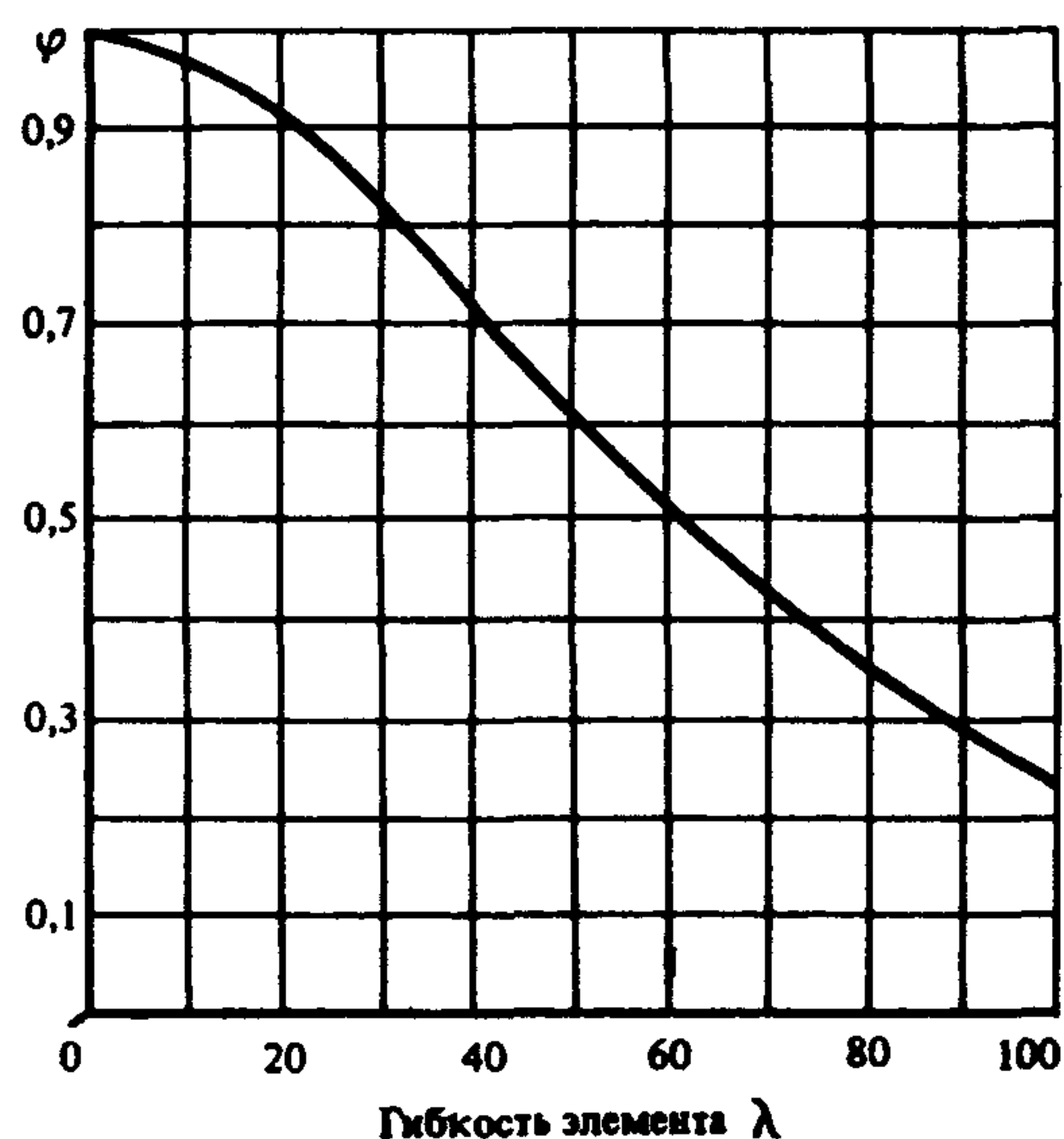
Черт 10 График для определения коэффициента продольного изгиба \varphi
