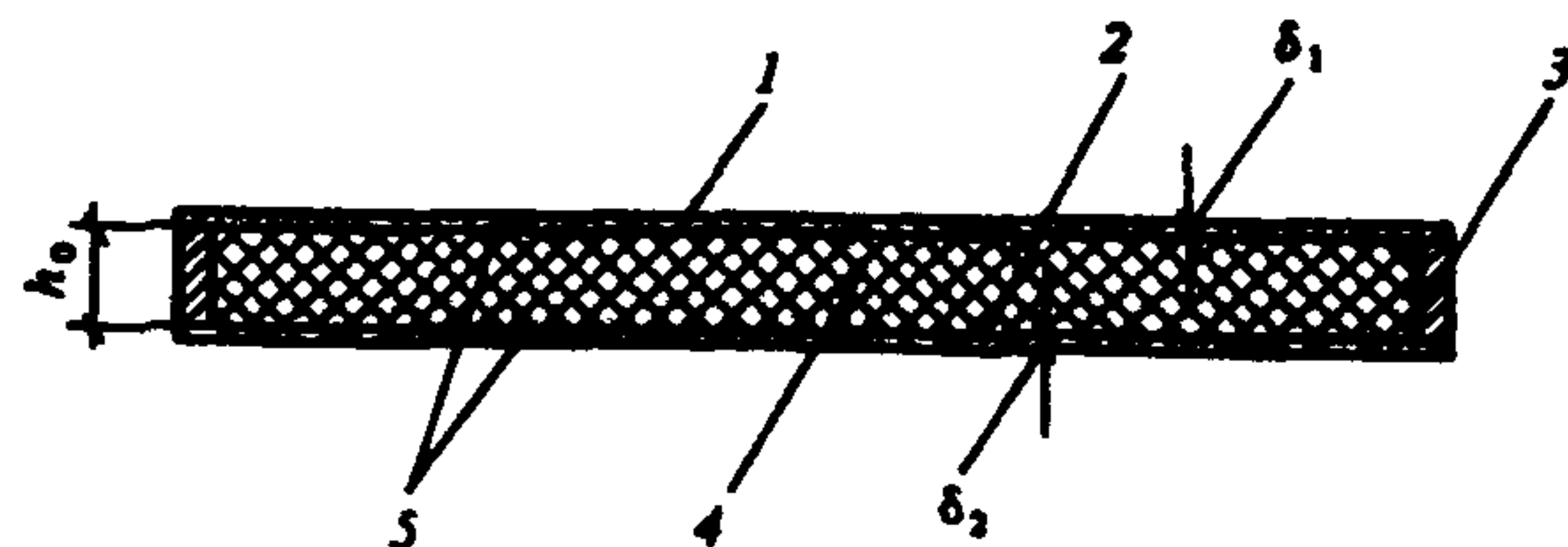
Черт. 5 Поперечное сечение бескаркасной панели с обрамлением
