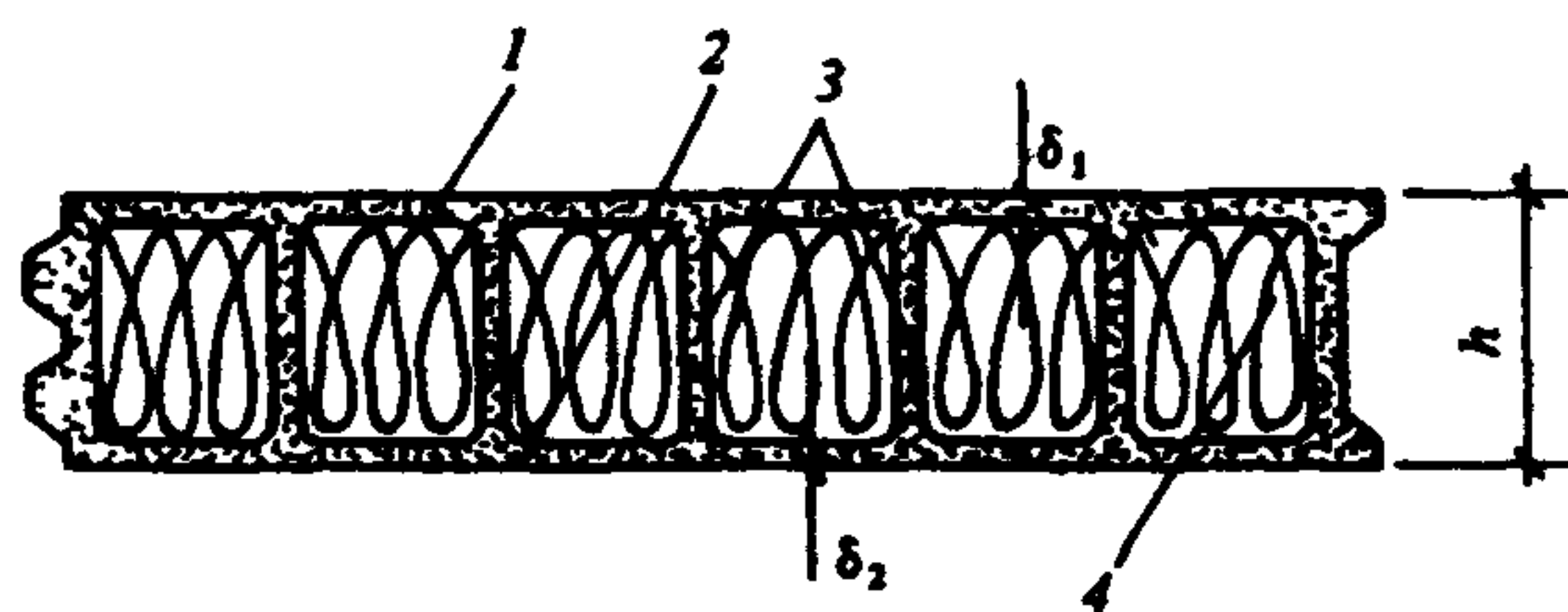
Черт. 4 Поперечное сечение экструзионной панели 1, 2 — полки панели, 3 — ребра панели; 4 — утеплитель
