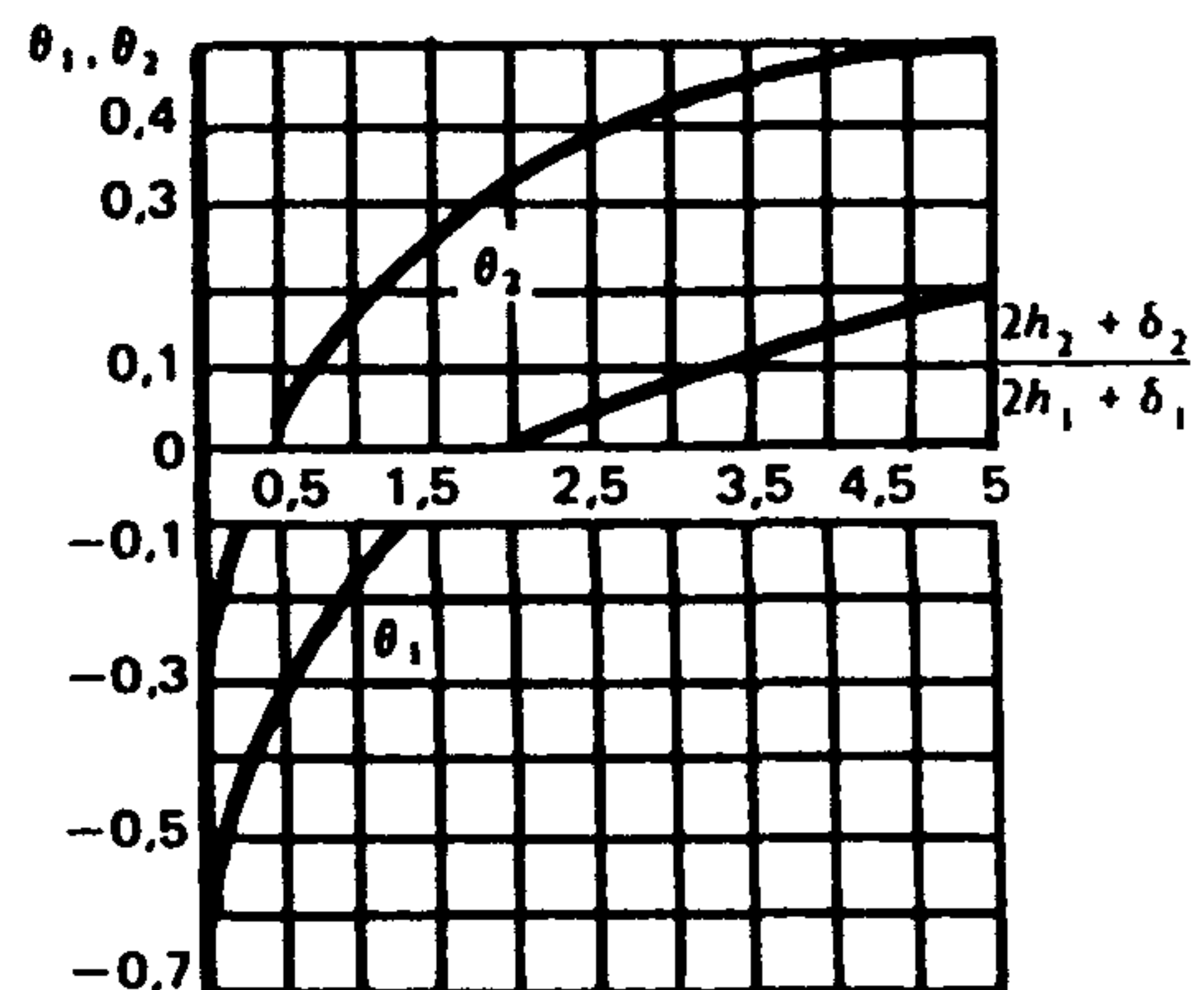
Черт. 8. График для определения коэффициентов \theta_1 и \theta_2
