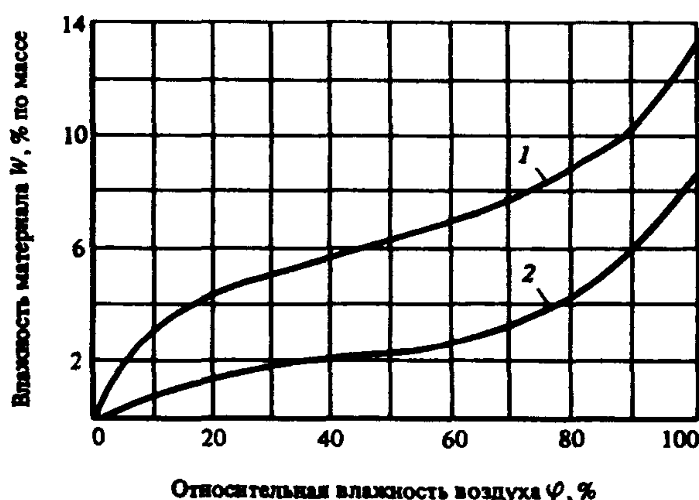
Черт 9. Зависимость влажности W листового 1 и экструзионного 2 асбестоцементов от относительной влажности воздуха \varphi
