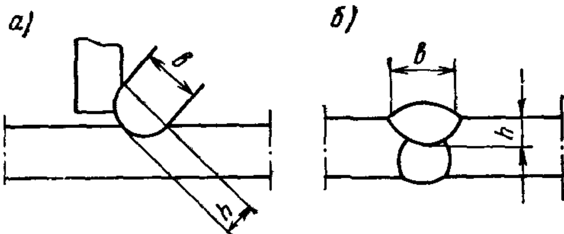
Рис. 1. Форма провара сварных соединений
