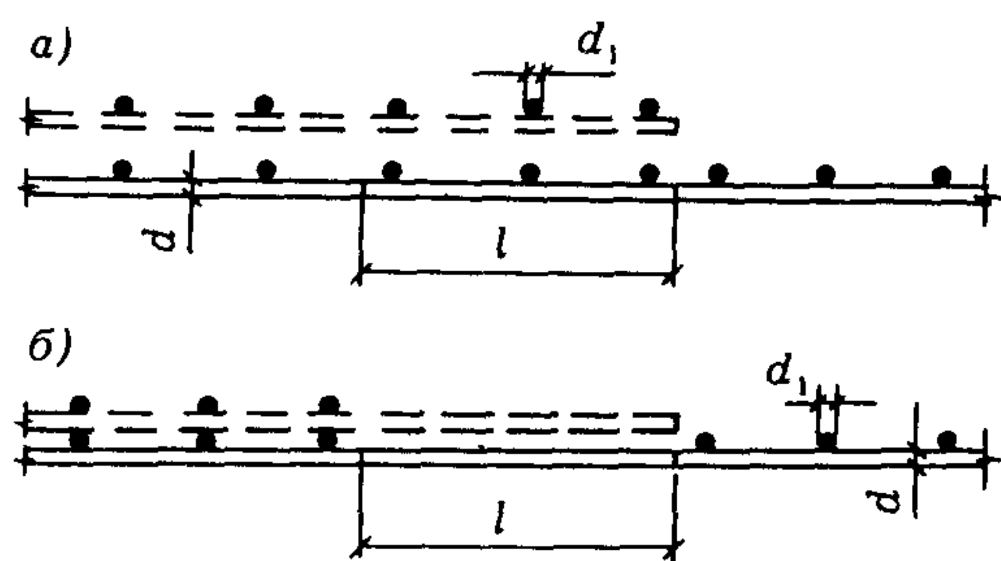
Черт. 25. Стыки сварных сеток внахлестку (без сварки) в направлении рабочей арматуры, выполненной из стержней периодического профиля
