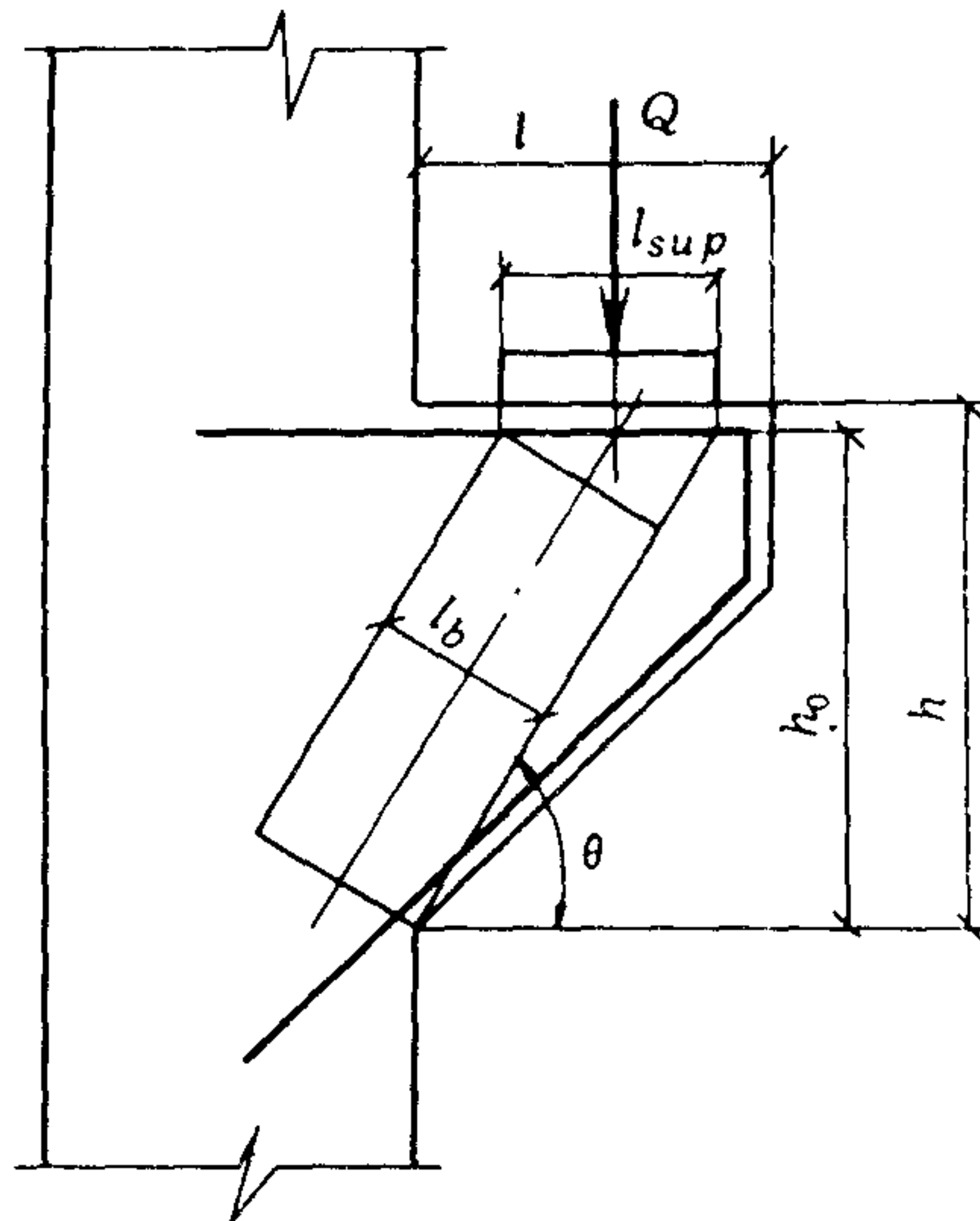
Черт. 11. Схема для расчета коротких консолей
