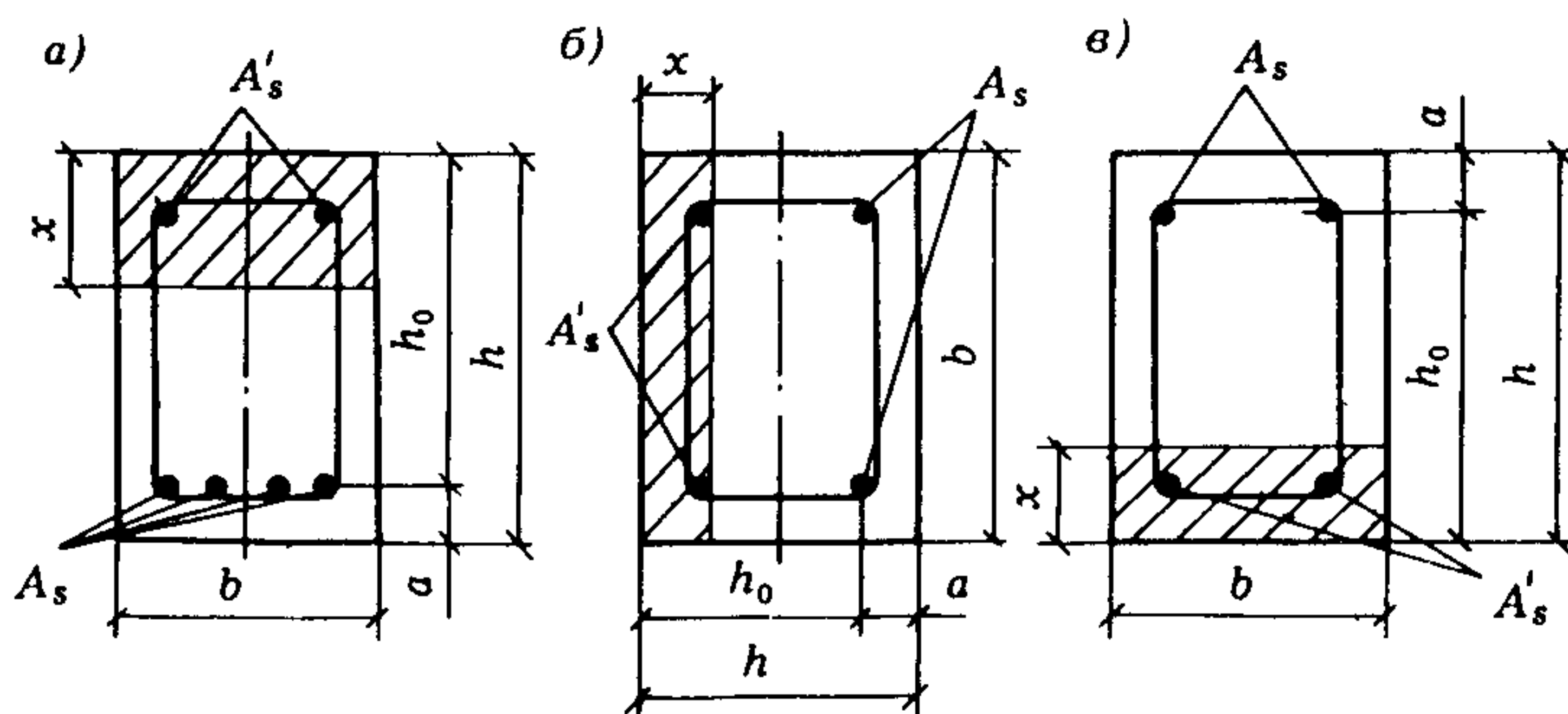
Черт. 14. Схемы расположения сжатой зоны пространственного сечения
