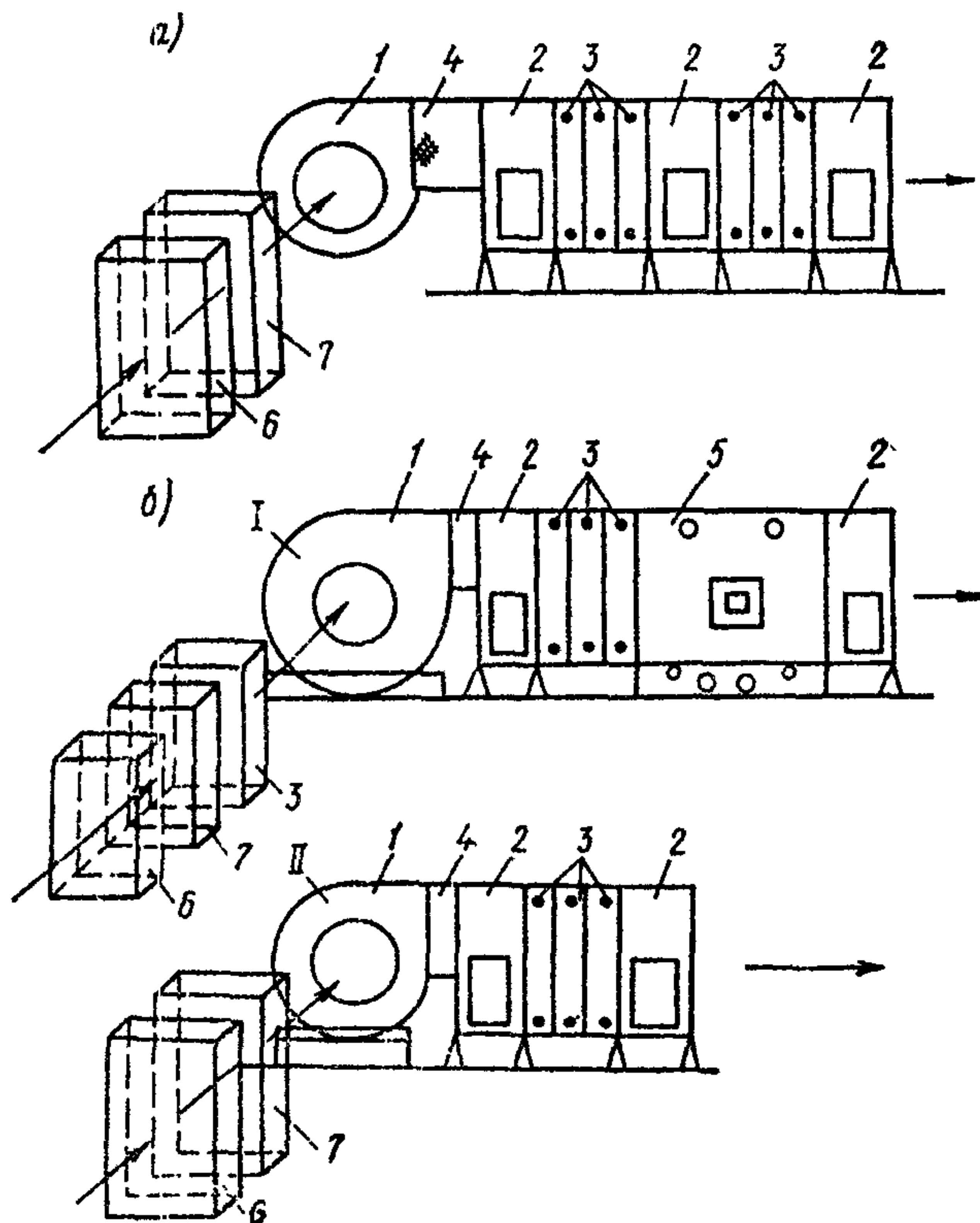
Рис. 5. Типовые компоновки приточных кондиционеров
