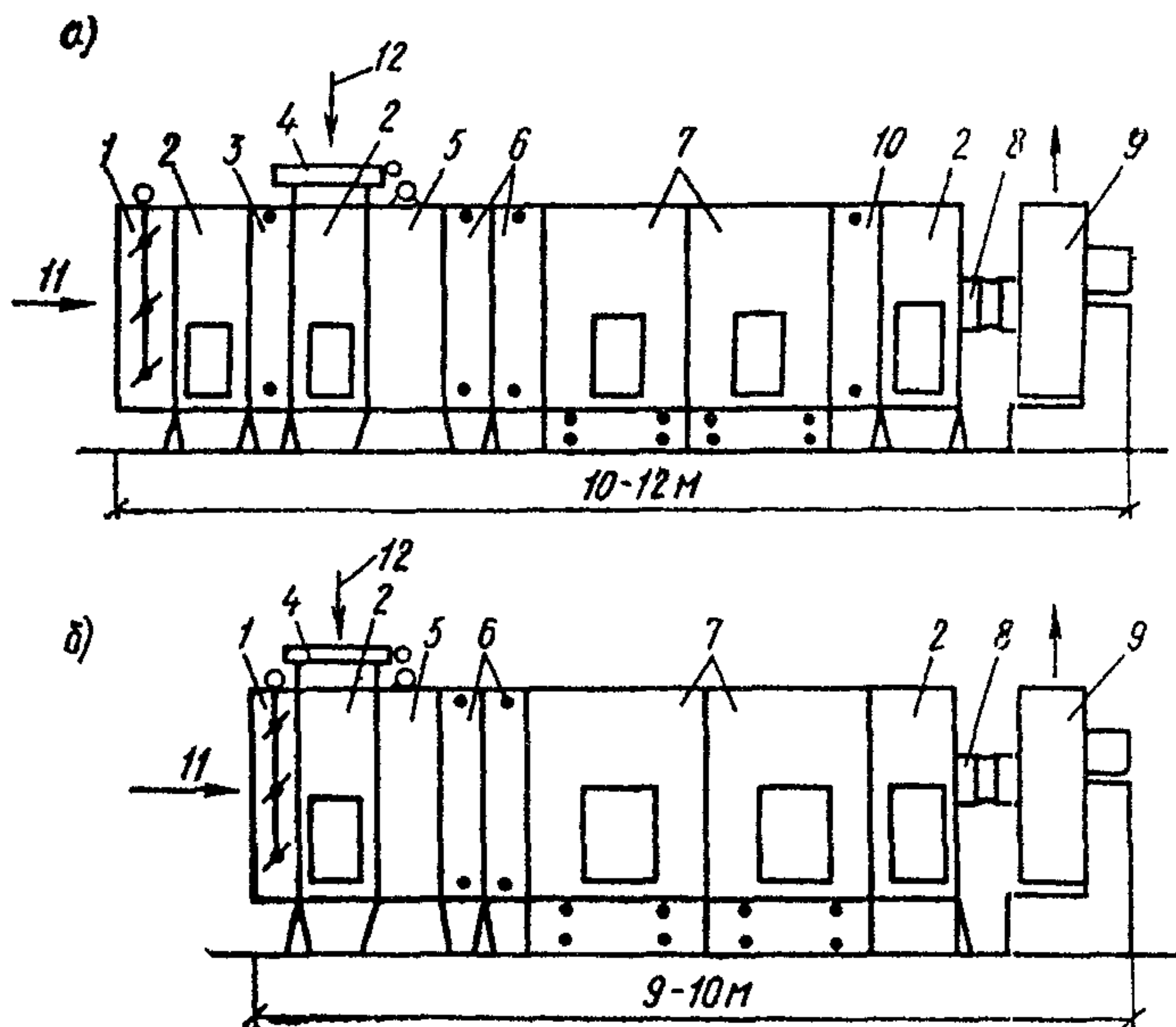
Рис. 4. Типовые компоновки испарительного кондиционера
