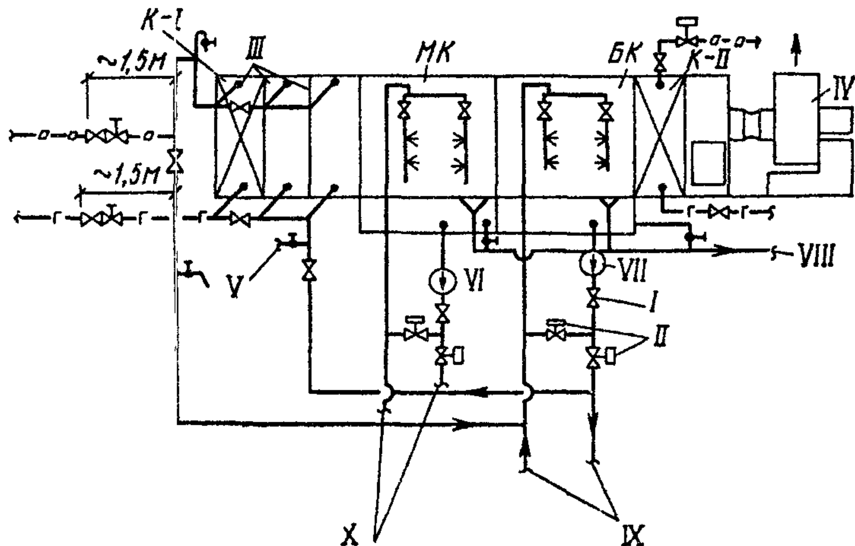
Рис. 3. Схема обвязки трубопроводами испарительного кондиционера I — обратный клапан; II — взаимобратные клапаны; III — теплообменник (воздухоохладитель); К-I — теплообменник первого подогрева (элемент теплообменника III ); МК — оросительная камера малого контура циркуляции; БК — оросительная камера большого контура циркуляции; К-II — теплообменник второго подогрева; IV — вентилятор испарительного кондиционера; V — спуск воды в канализацию; VI , VII — соответственно циркуляционные насосы малого и большого контура циркуляции; VIII — канализационная линия; IX — трубопроводы к теплообменнику I приточного кондиционера; X — трубопроводы к теплообменнику II приточного кондиционера; —г—г— горячая магистраль; —о—о— обратная магистраль
