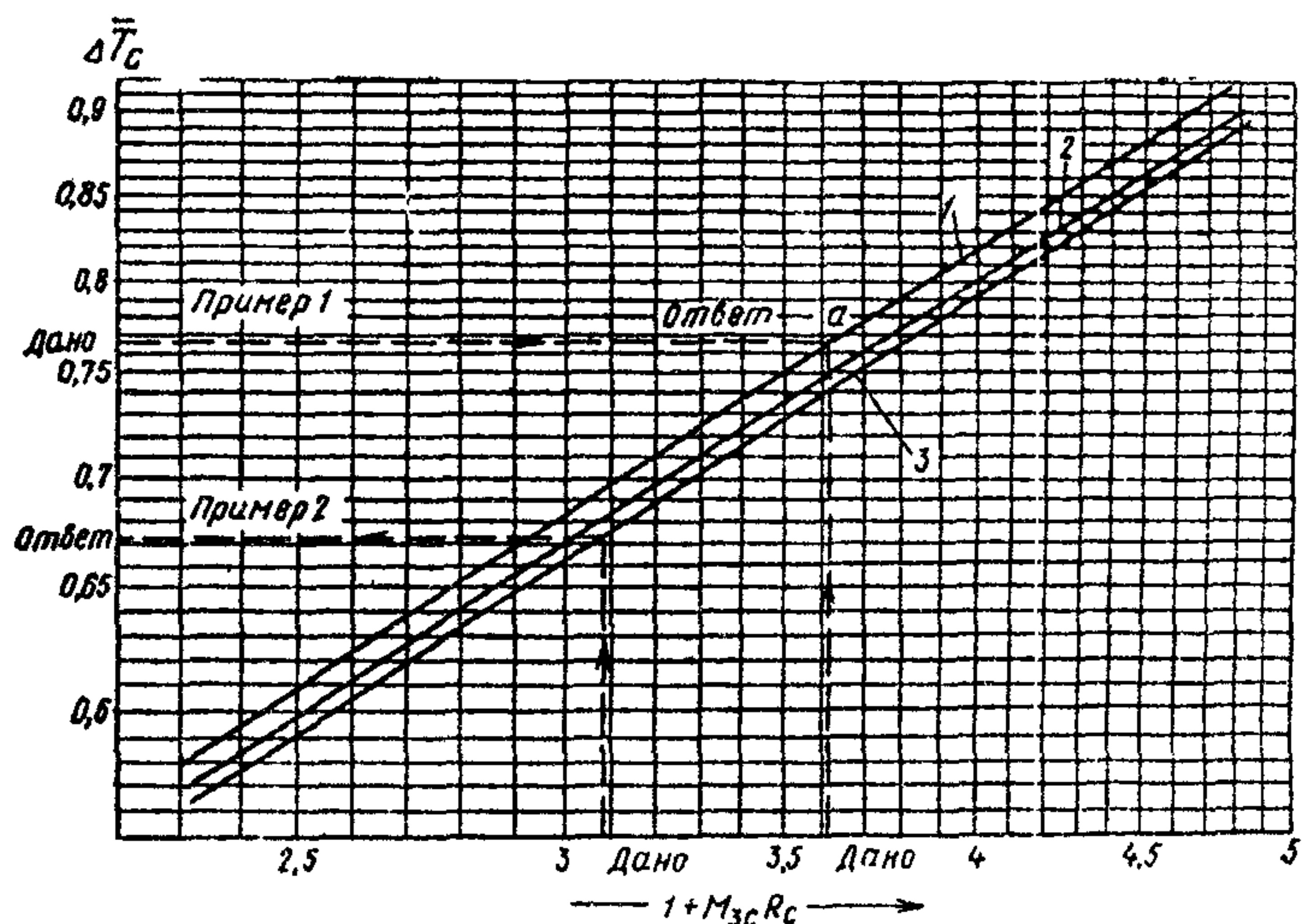
Рис. 10. График для определения величины охлаждения воздуха \Delta T_c в бескомпрессорных системах кондиционирования воздуха Линии 1, 2 и 3 соответствуют характеристикам систем в табл. 1
