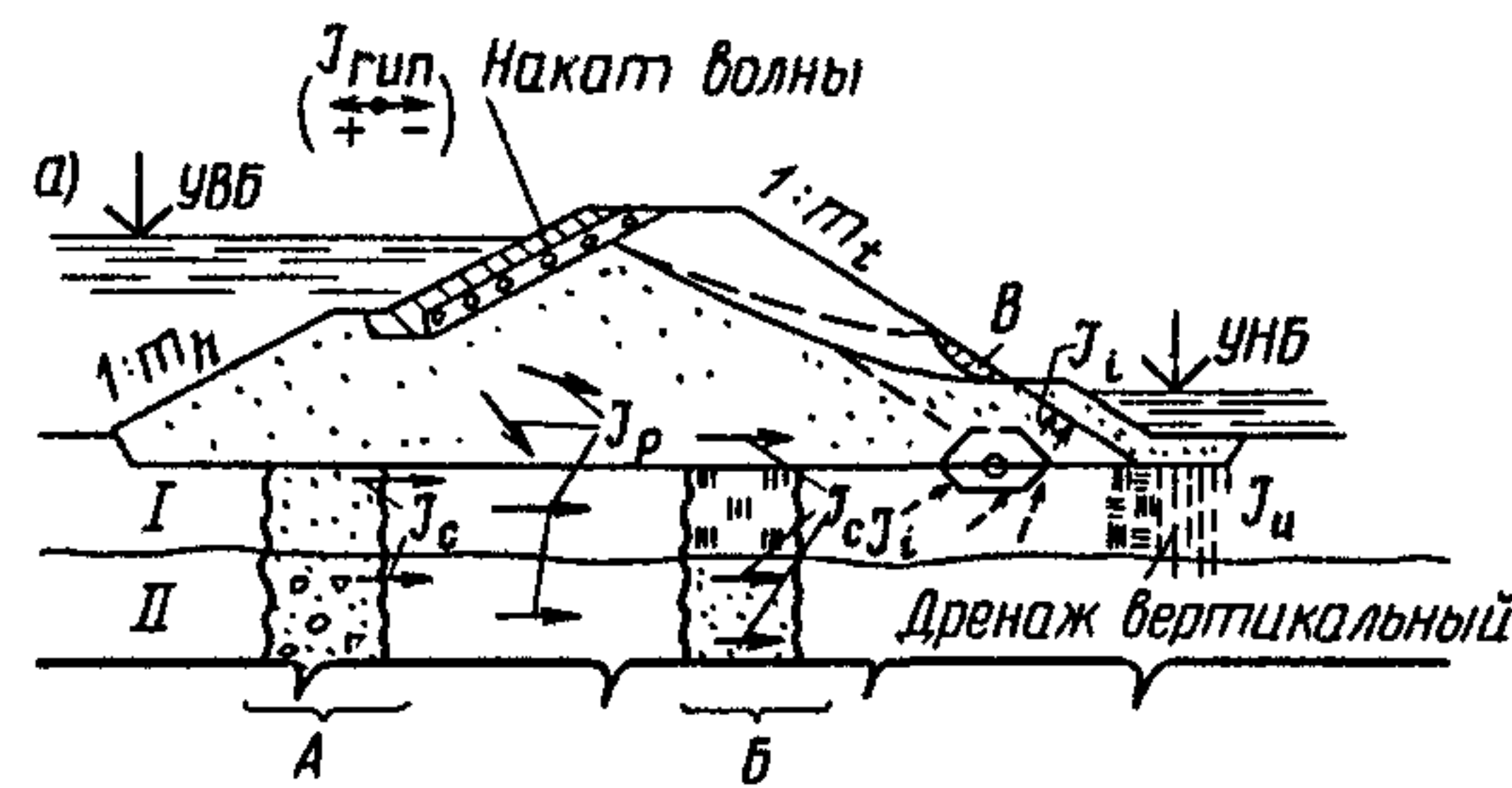
Черт. 9. Фильтрационные деформации в земляных и каменно-земляных плотинах и их основаниях
