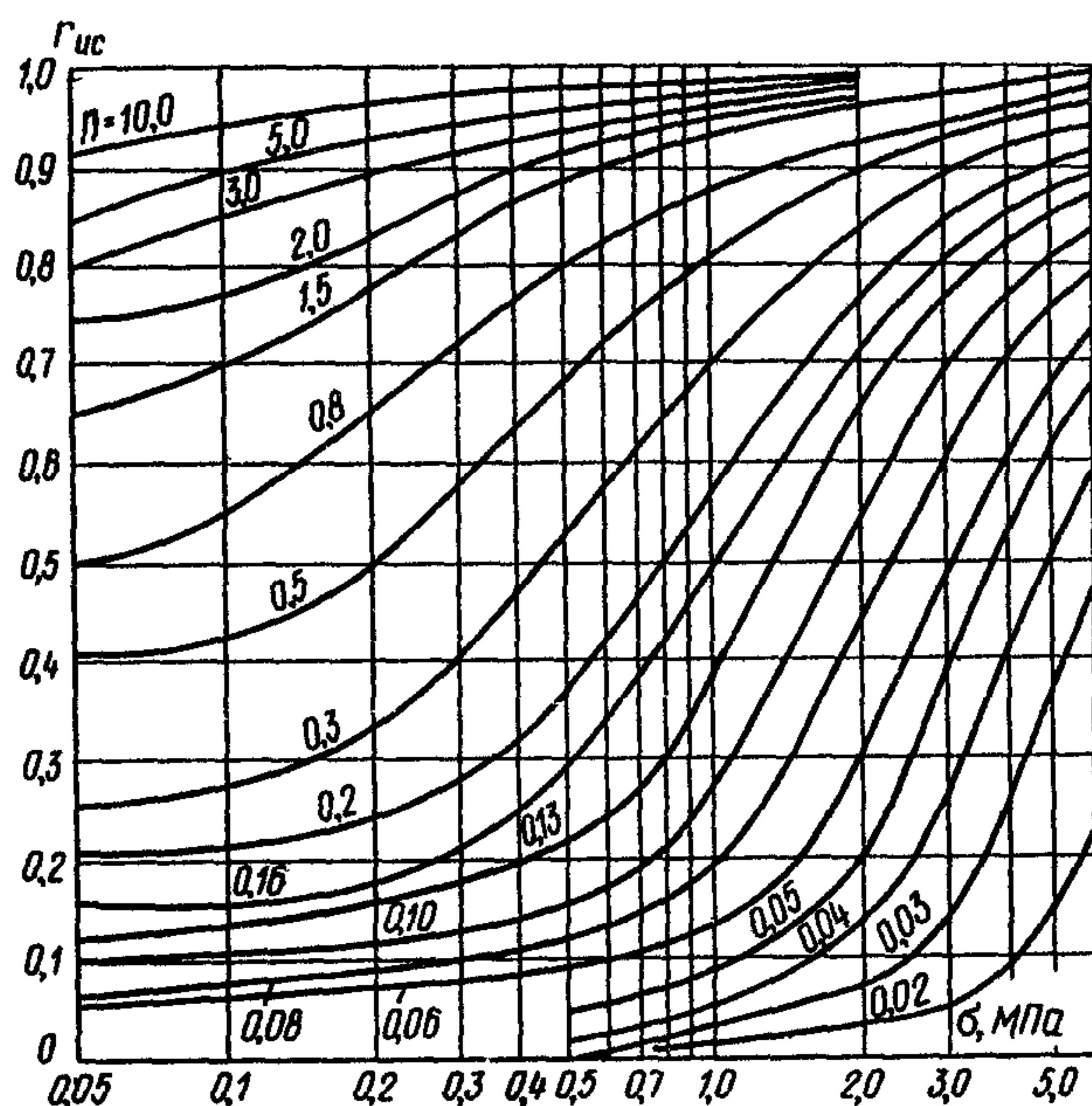
Черт. 1. Номограмма для определения коэффициента порового давления r_{uc}
