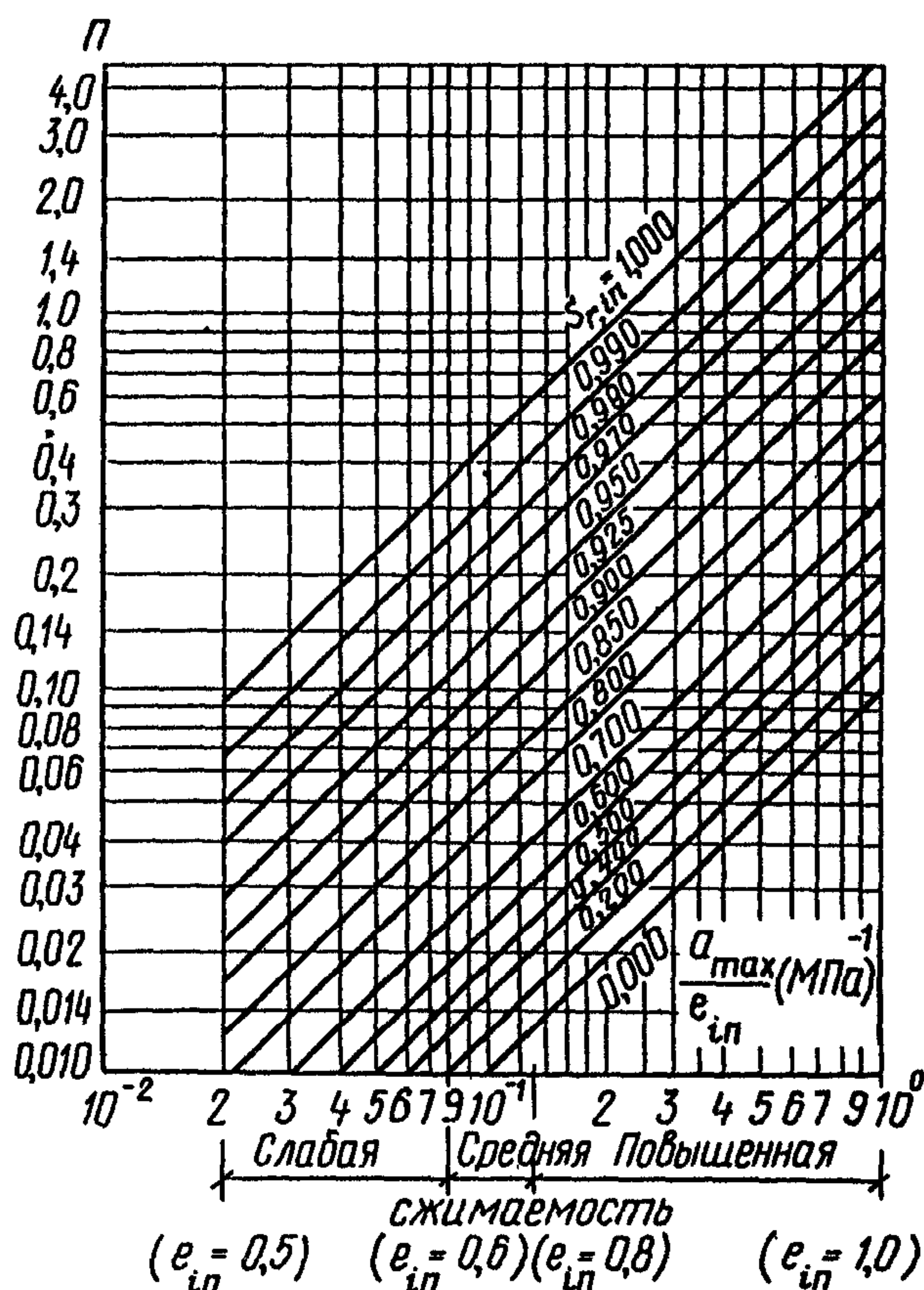
Черт. 2. Номограмма для определения параметра \Pi
