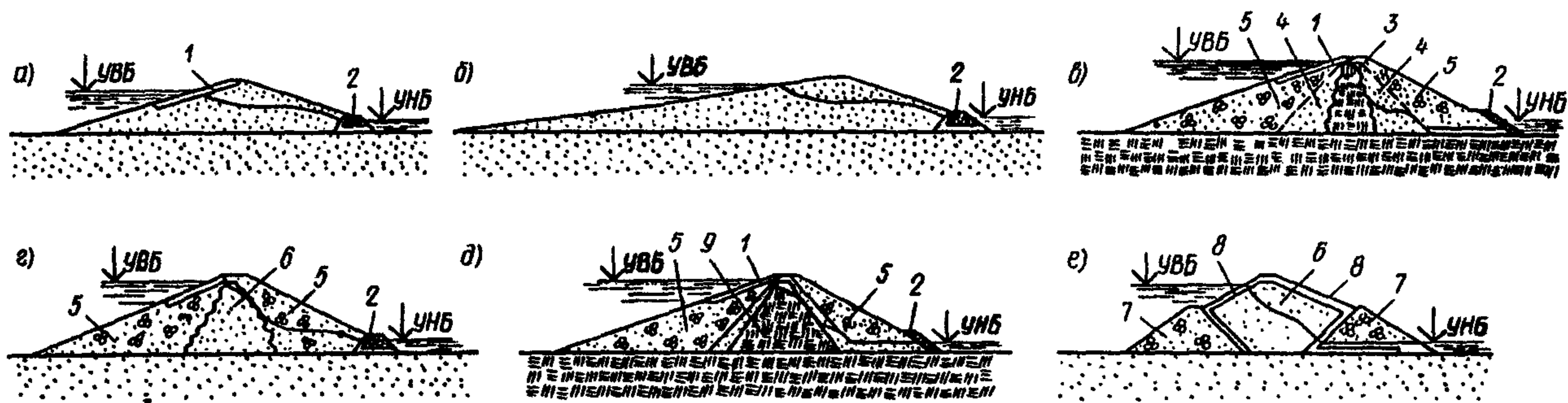
Черт. 3. Виды намывных плотин
