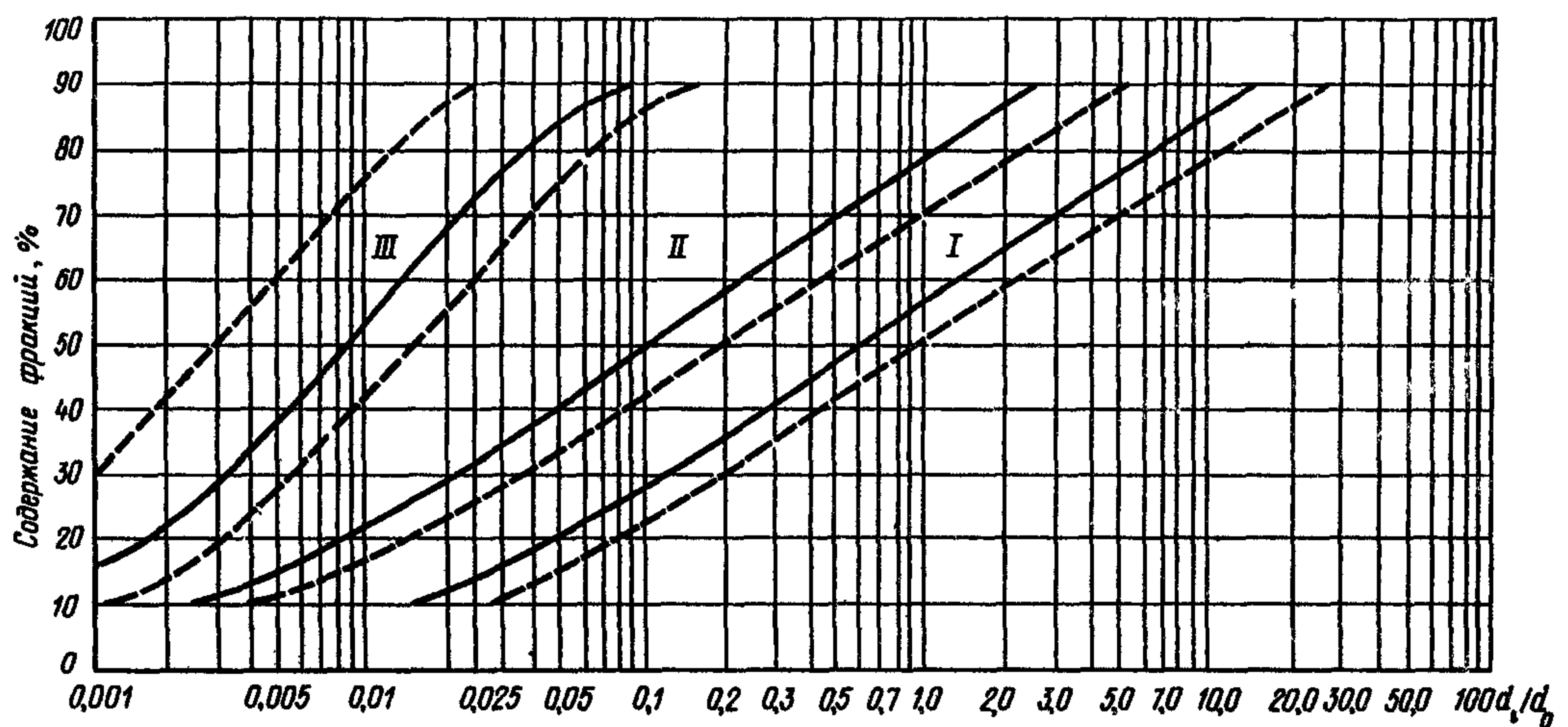
Черт. 5. График зависимости \alpha = f\left(\frac{d_i}{d_o}\right) . Гравийные плотины с ядром высотой более 30 м
