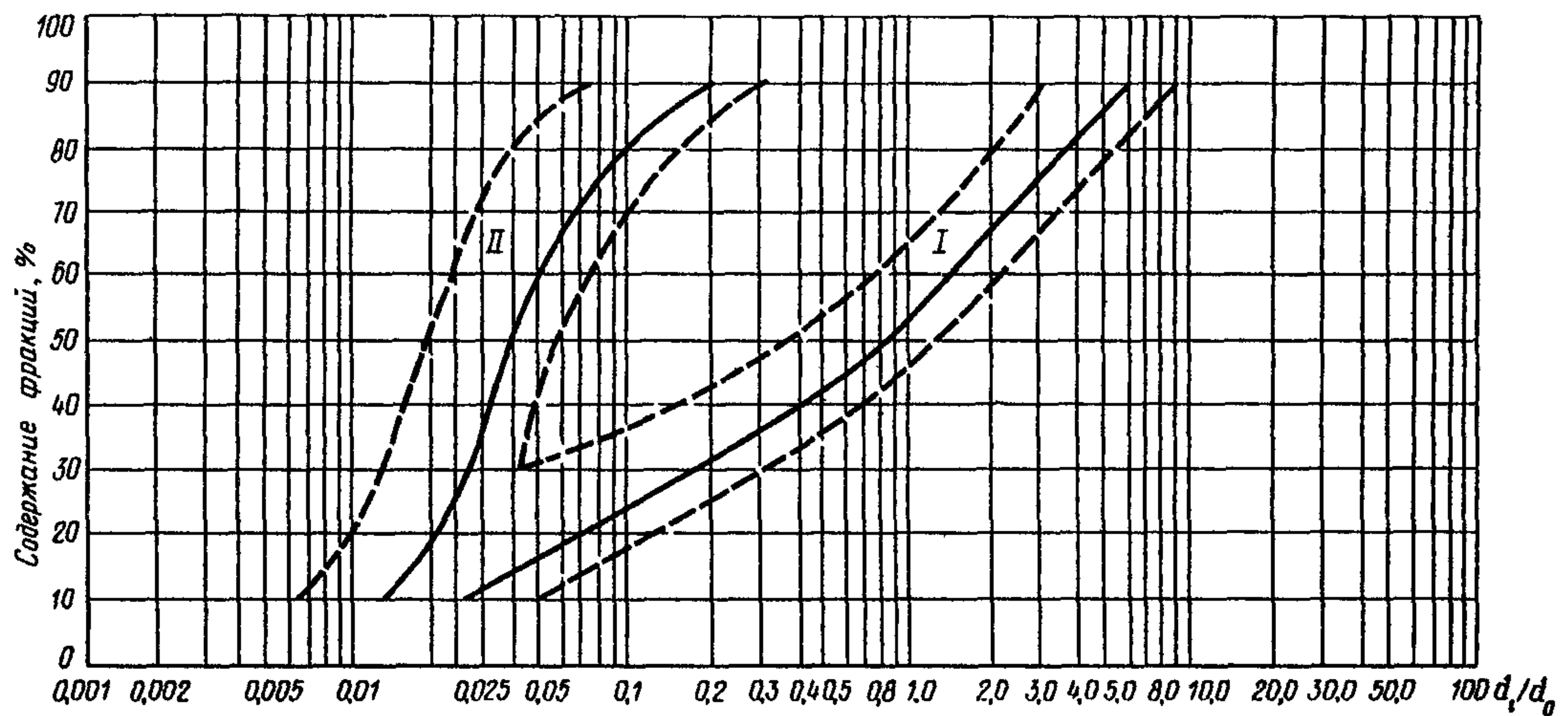
Черт. 3. График зависимости \alpha = f\left(\frac{d_i}{d_o}\right) . Неоднородные плотины из крупного песчано-гравийного грунта с центральной песчаной зоной
