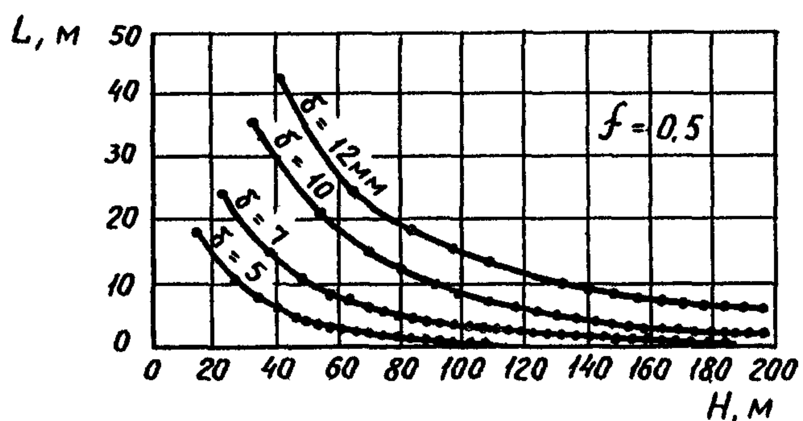
Черт. 1. Зависимость расстояния между горизонтальными швами диафрагмы по высоте L от толщины диафрагмы \delta , величины коэффициента трения грунта по диафрагме f и высоты диафрагмы H
