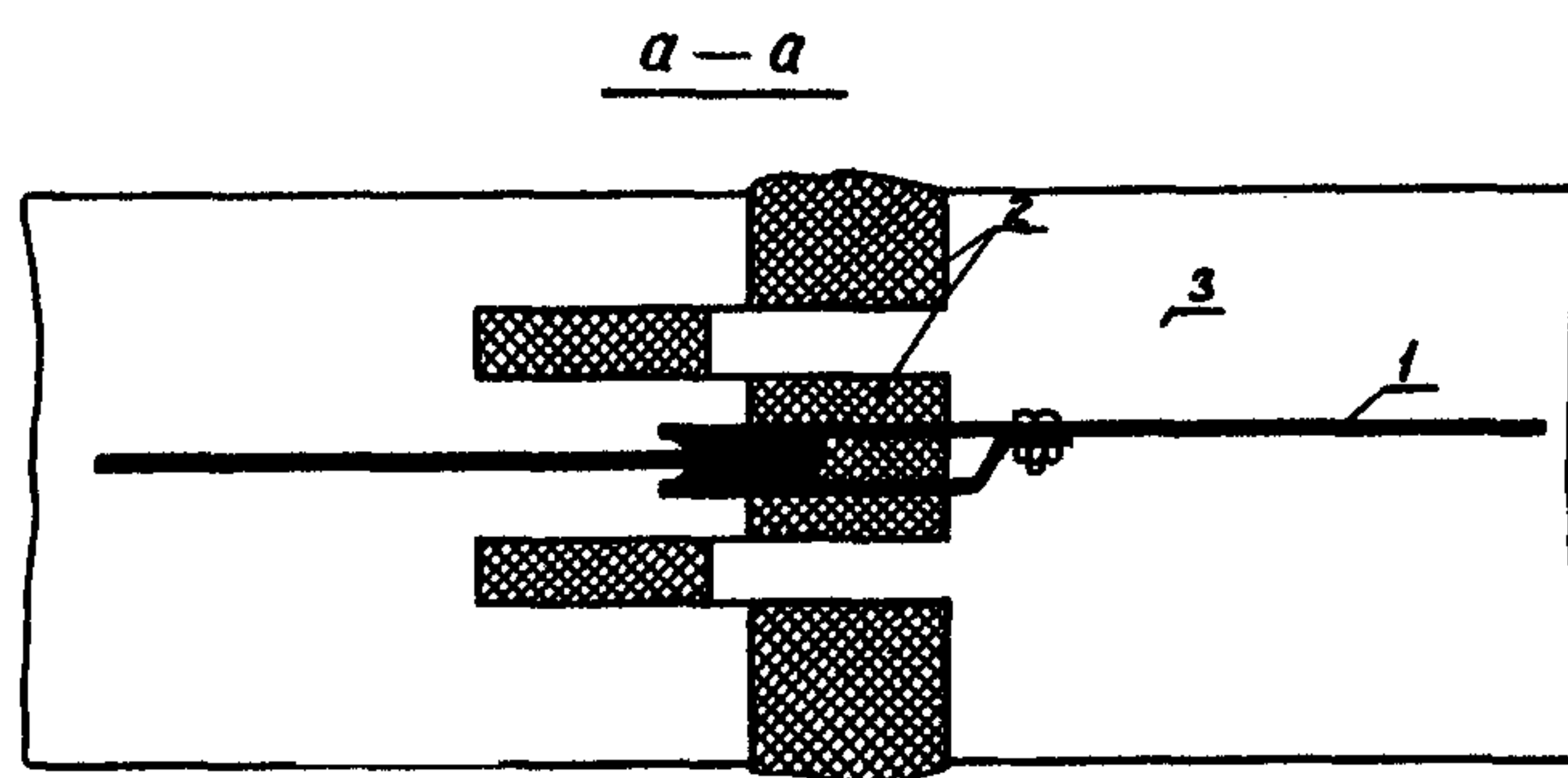
Черт. 2. Устройство деформационного шва в опорном элементе диафрагмы
