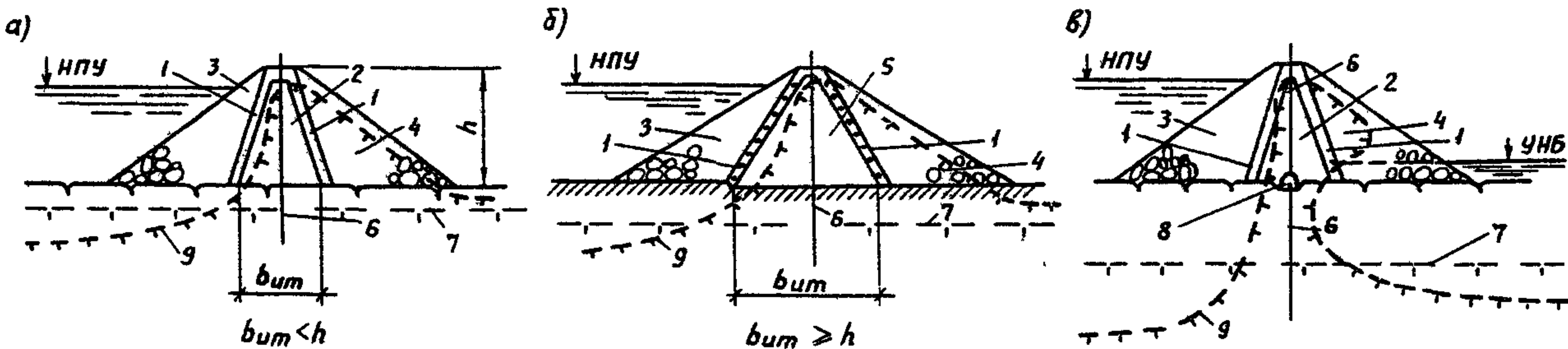
Черт. 6.1. Виды мерзлых каменно-земляных плотин в северной строительной-климатической зоне
