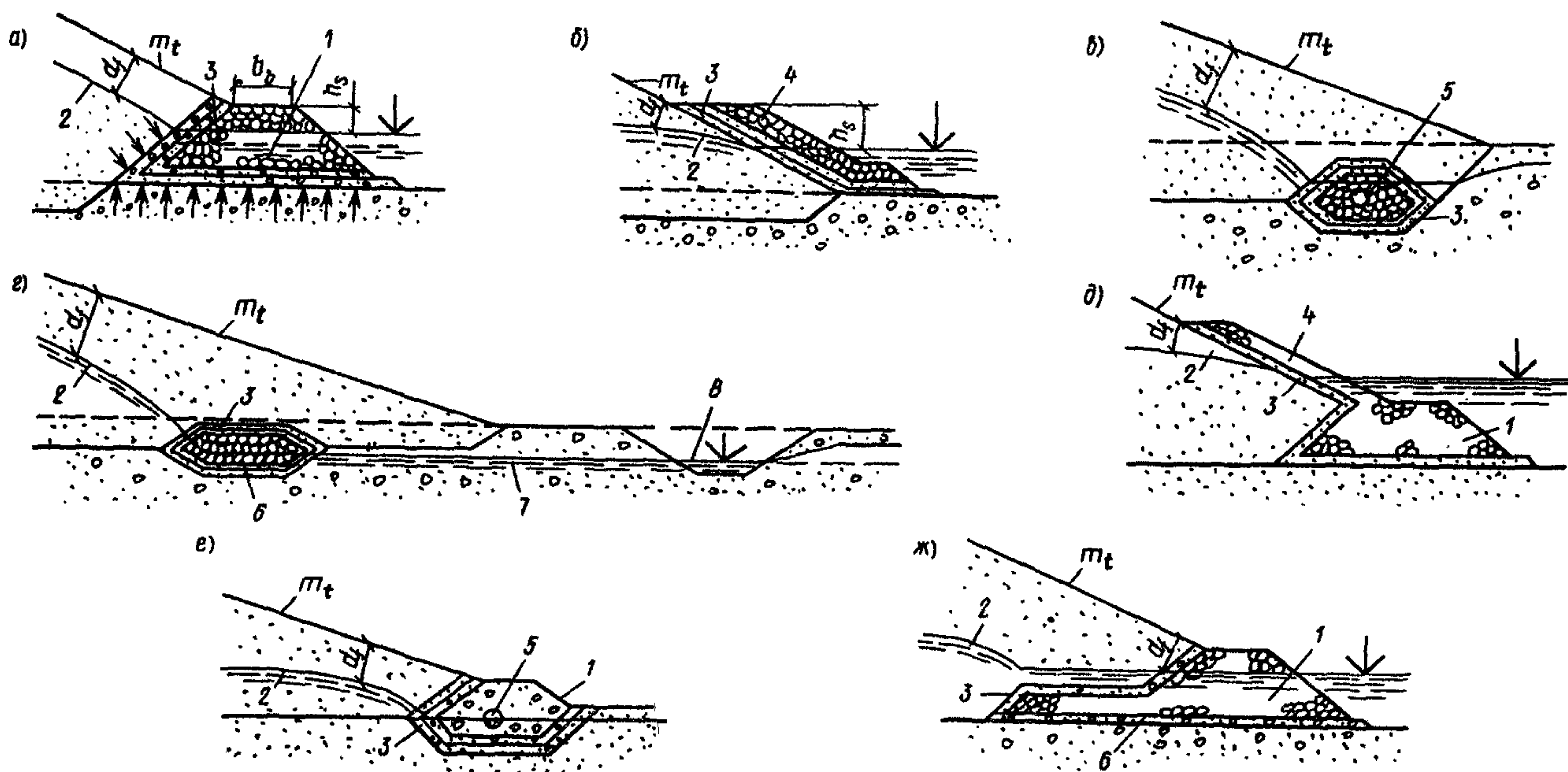
Черт. 2. Схемы основных видов дренажа
