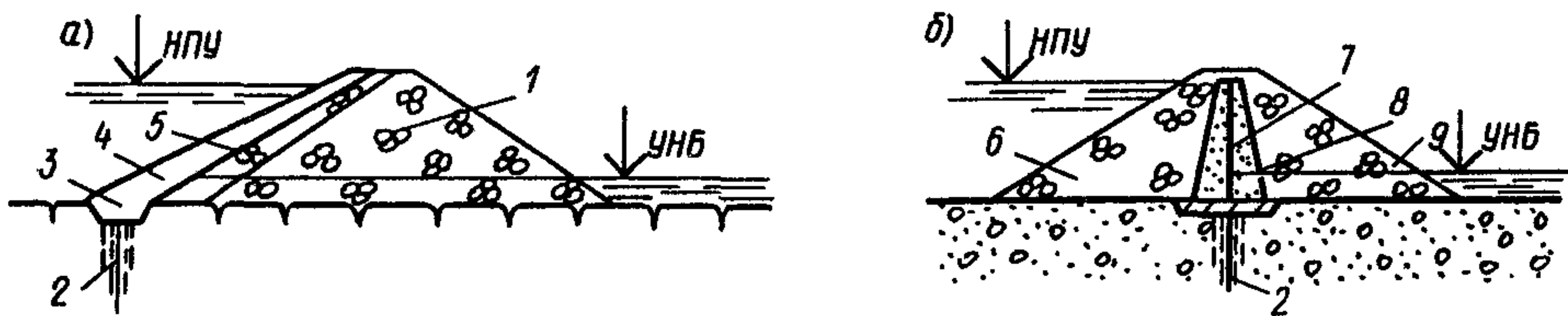
Черт. 8. Виды каменно-набросных плотин
