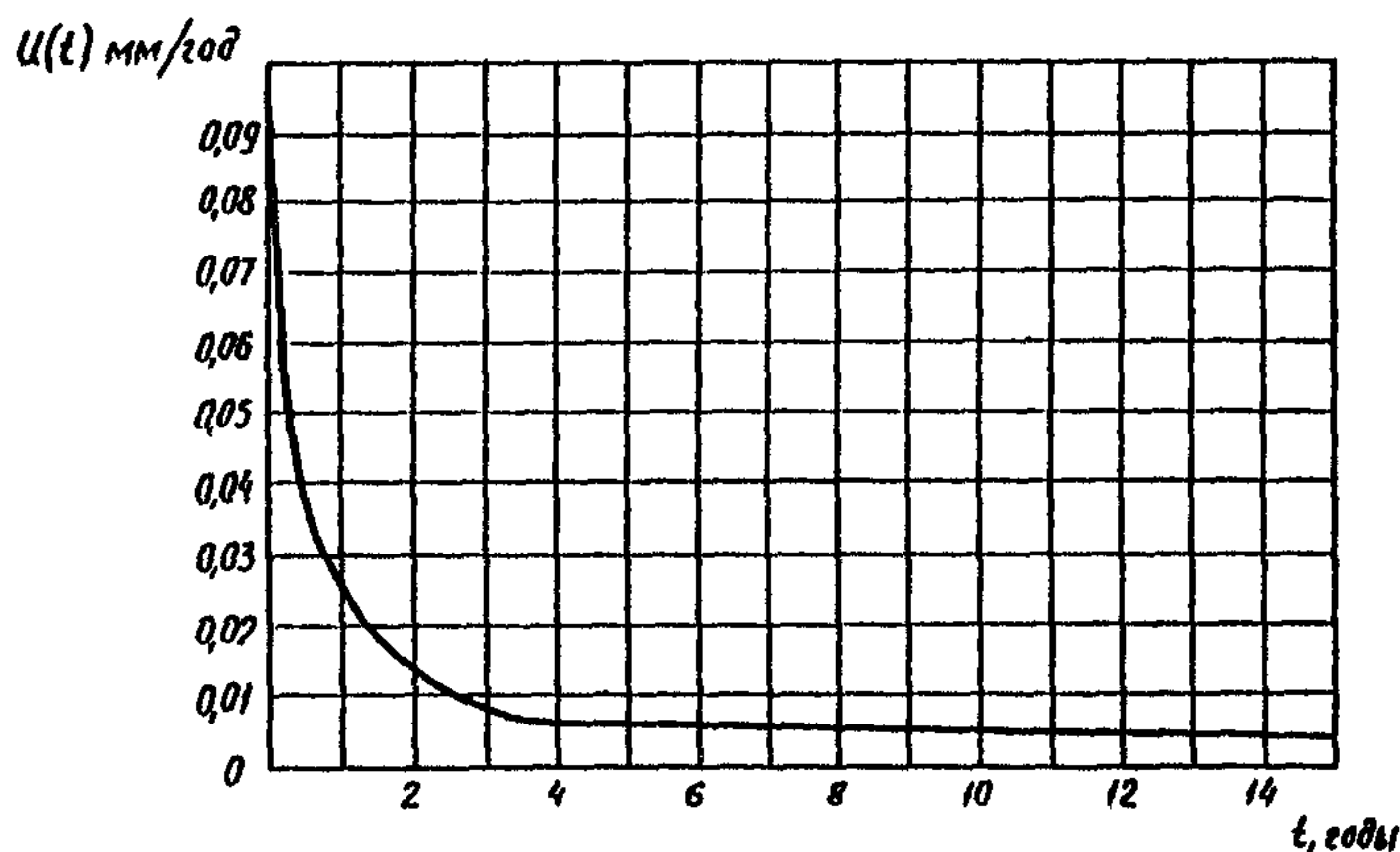
Черт. 6. Изменение средней скорости коррозии стальной диафрагмы в водно-грунтовой среде северной строительно-климатической зоны
