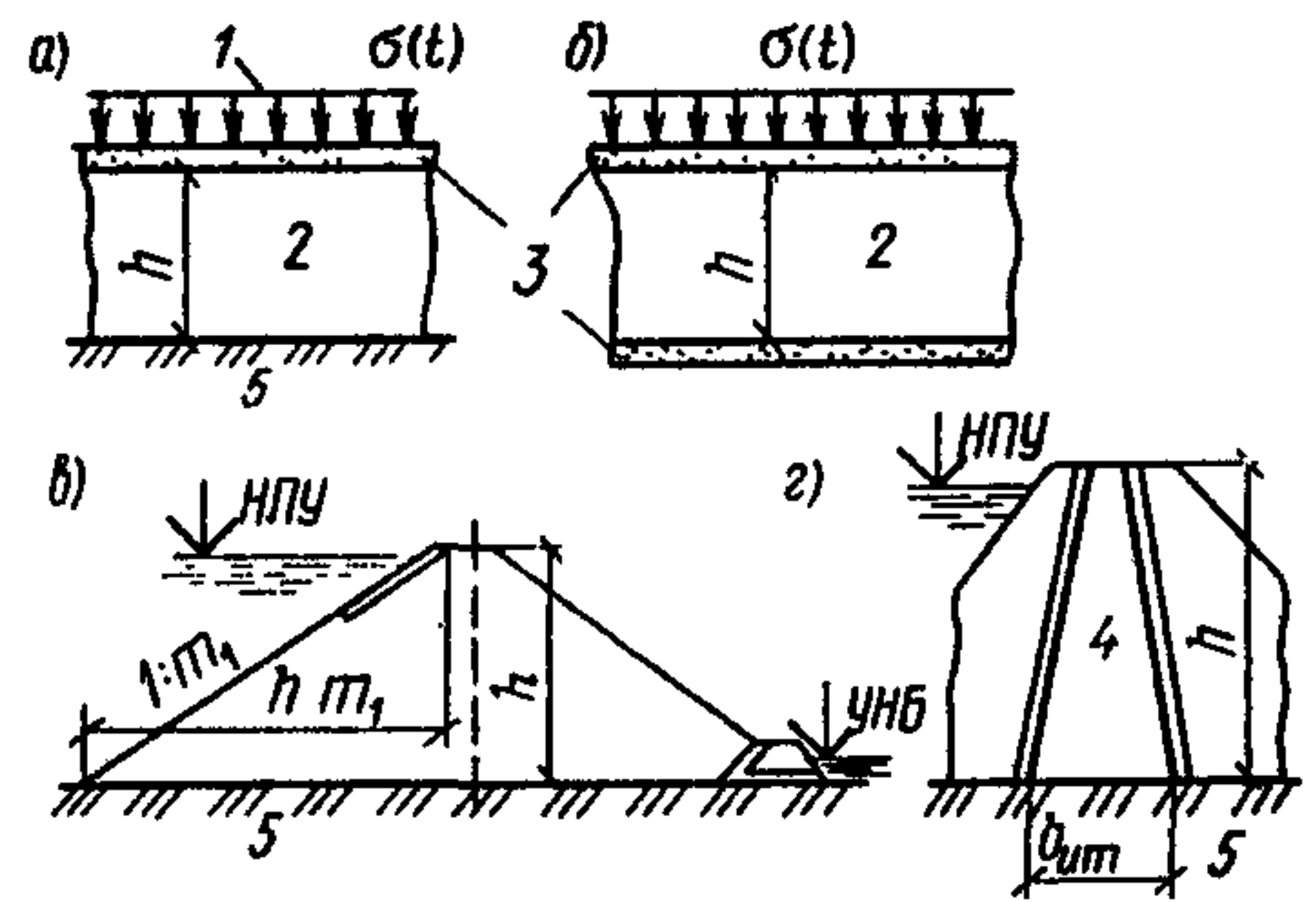
Черт. 4. Различные случаи определения коэффициента порового давления r_{uo}
