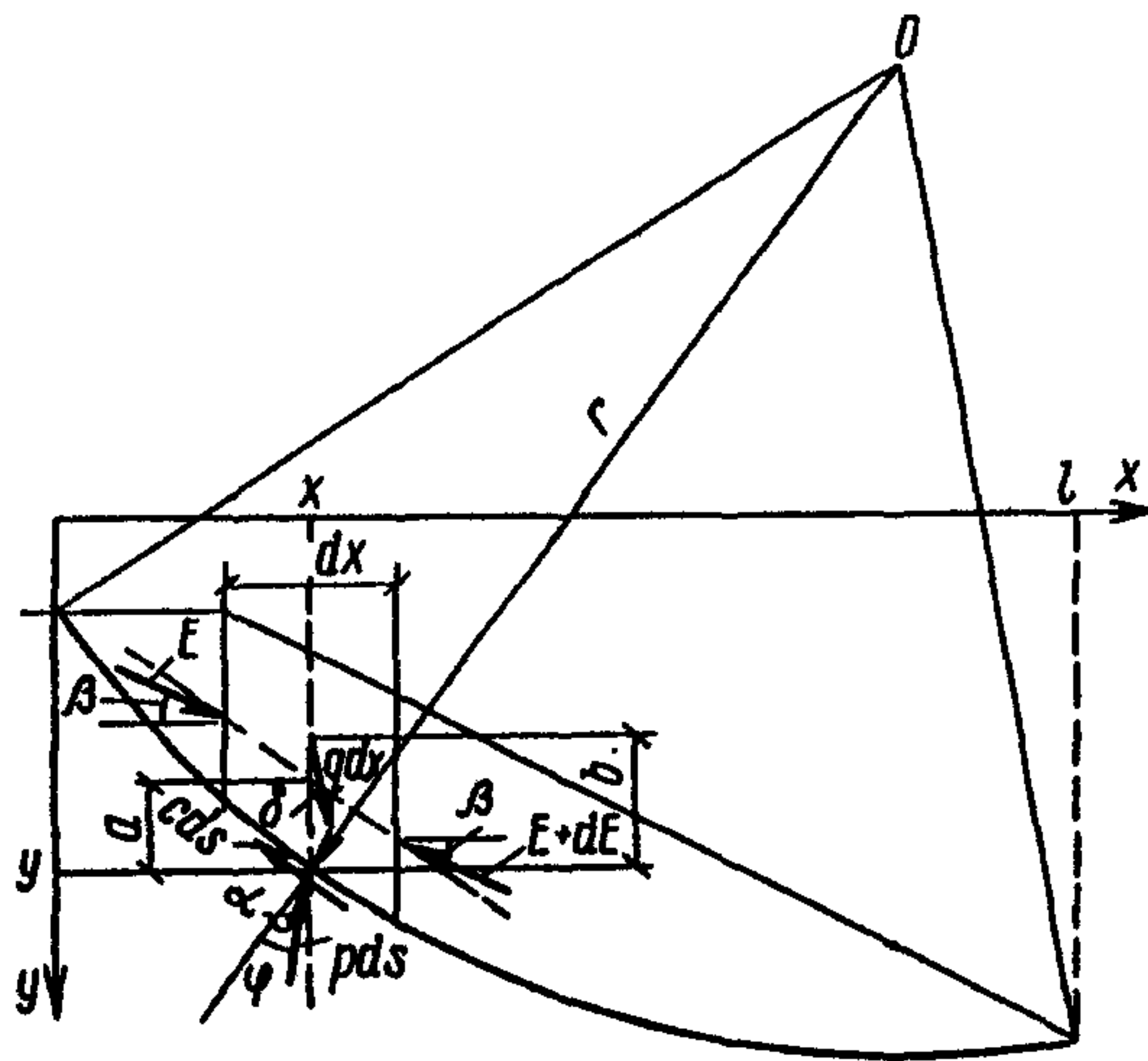
Схема сил, действующих на элемент призмы обрушения
