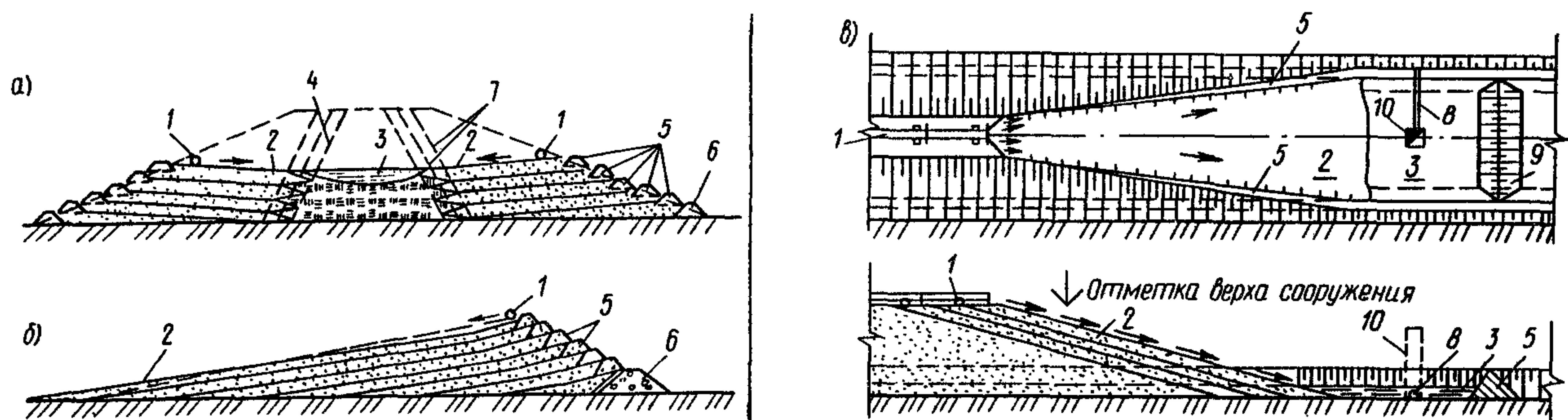
Черт. 4. Основные схемы возведения намывных плотин
