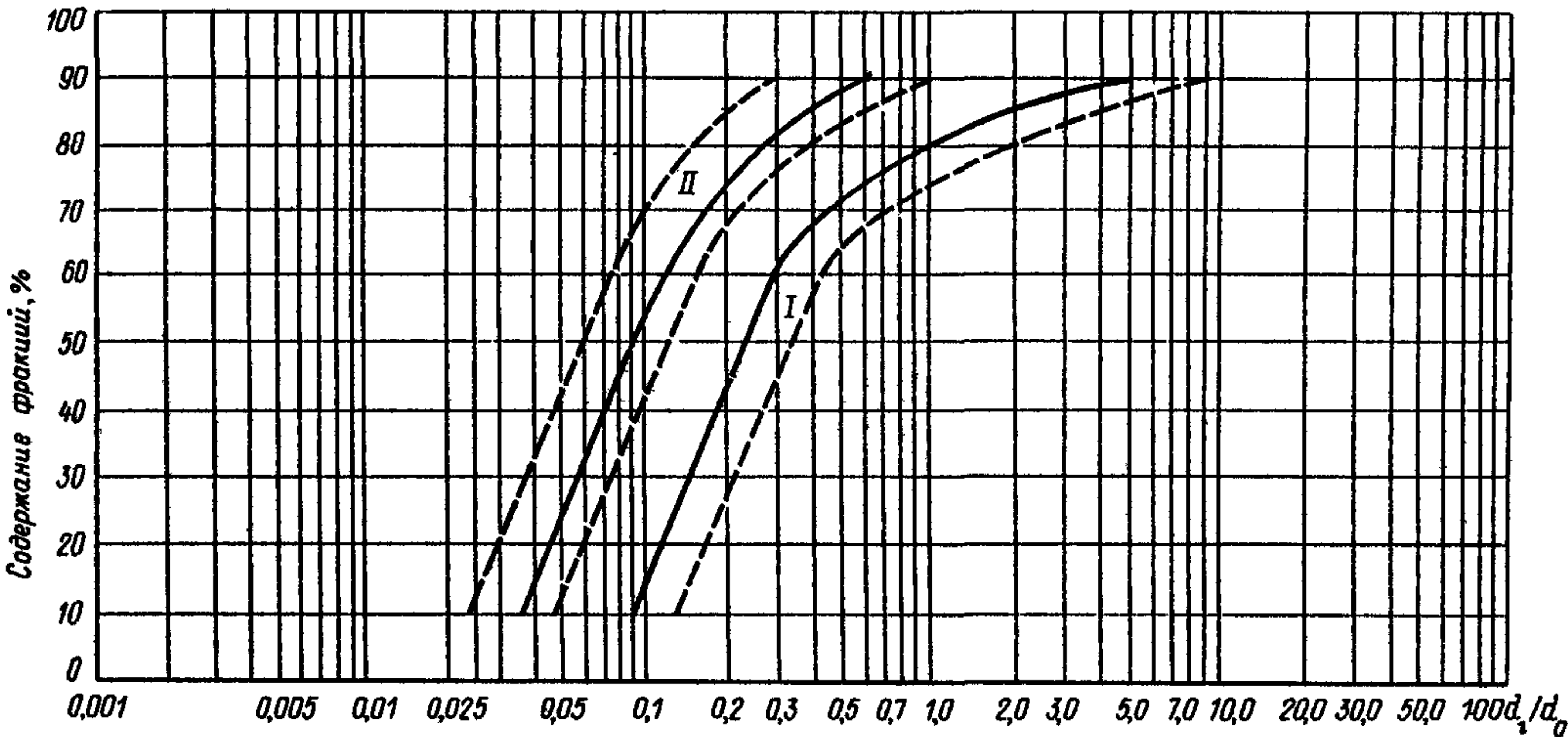
Черт. 2. График зависимости \alpha = f\left(\frac{d_i}{d_o}\right) . Неоднородные плотины из мелкого песчано-гравийного грунта с центральной песчаной зоной I — боковая зона; II — центральная зона
