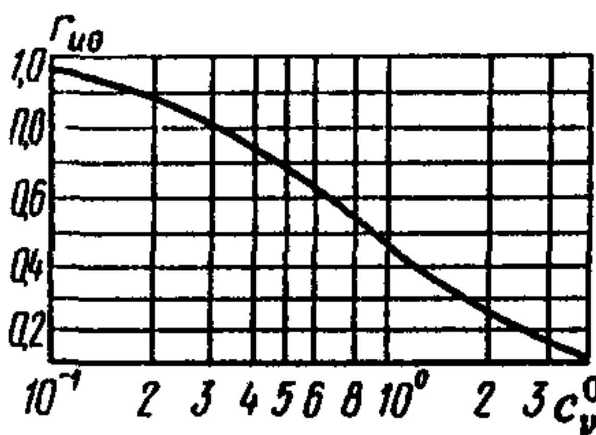
Черт. 3. График зависимости коэффициента порового давления r_{uo} от c_v^0
