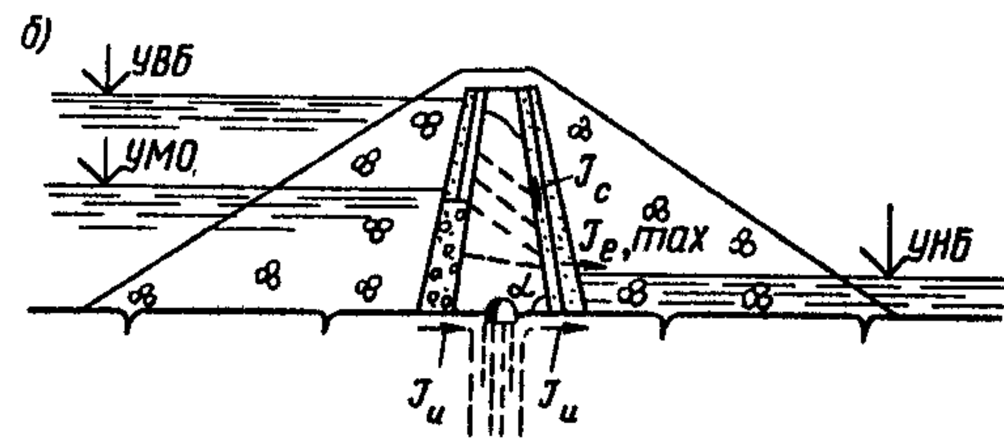
Черт. 9. Фильтрационные деформации в земляных и каменно-земляных плотинах и их основаниях
