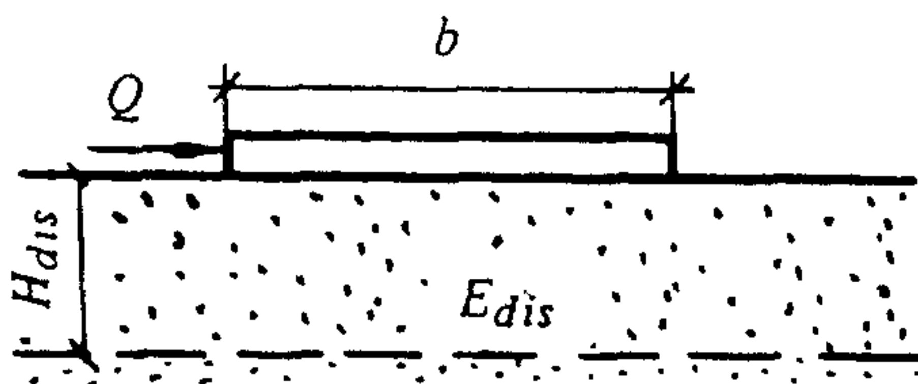
Черт. 1. Схемы к определению горизонтальных смещений сооружений
