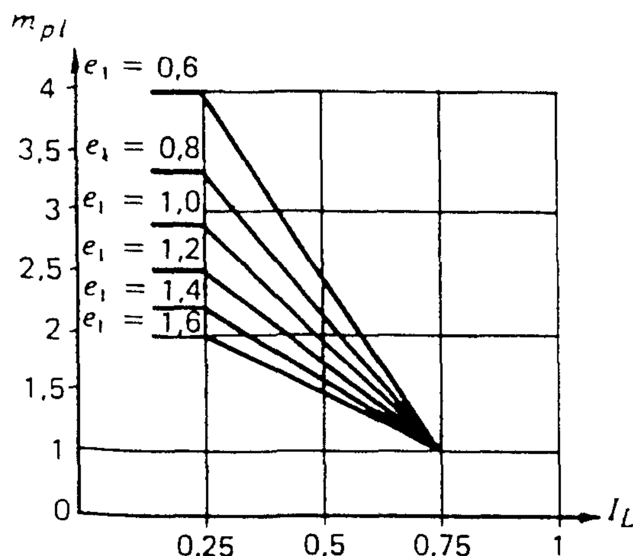
График для определения коэффициента m_{pl}
