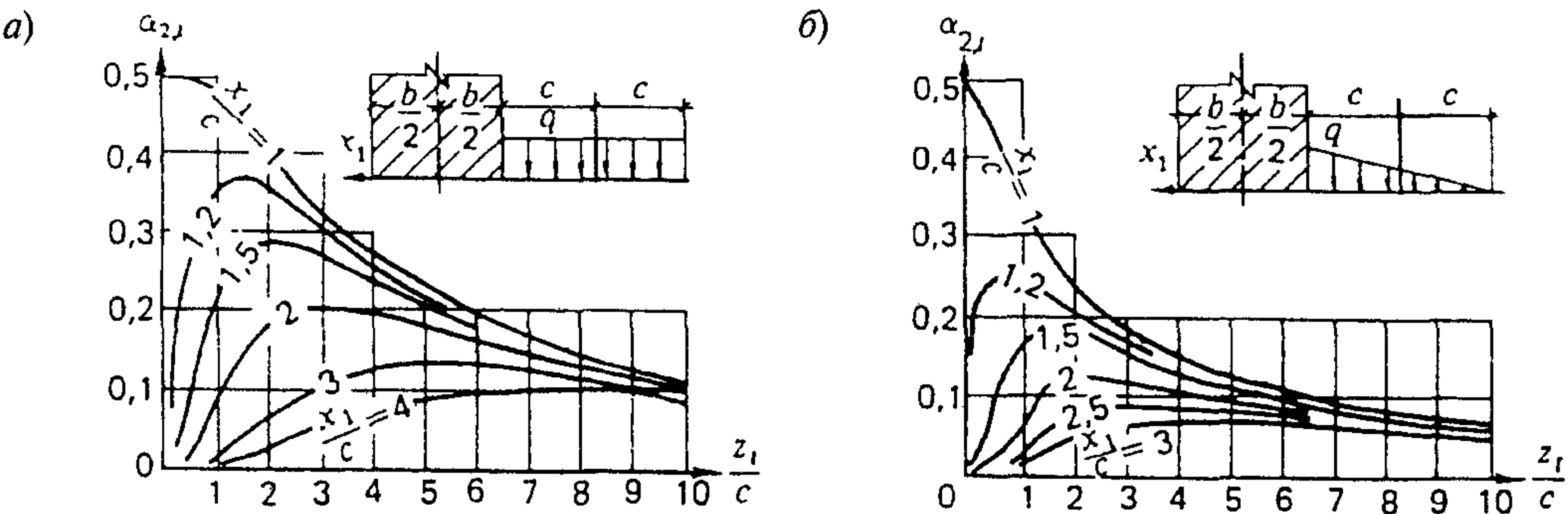
Графики для определения коэффициента \alpha_{2,i}
