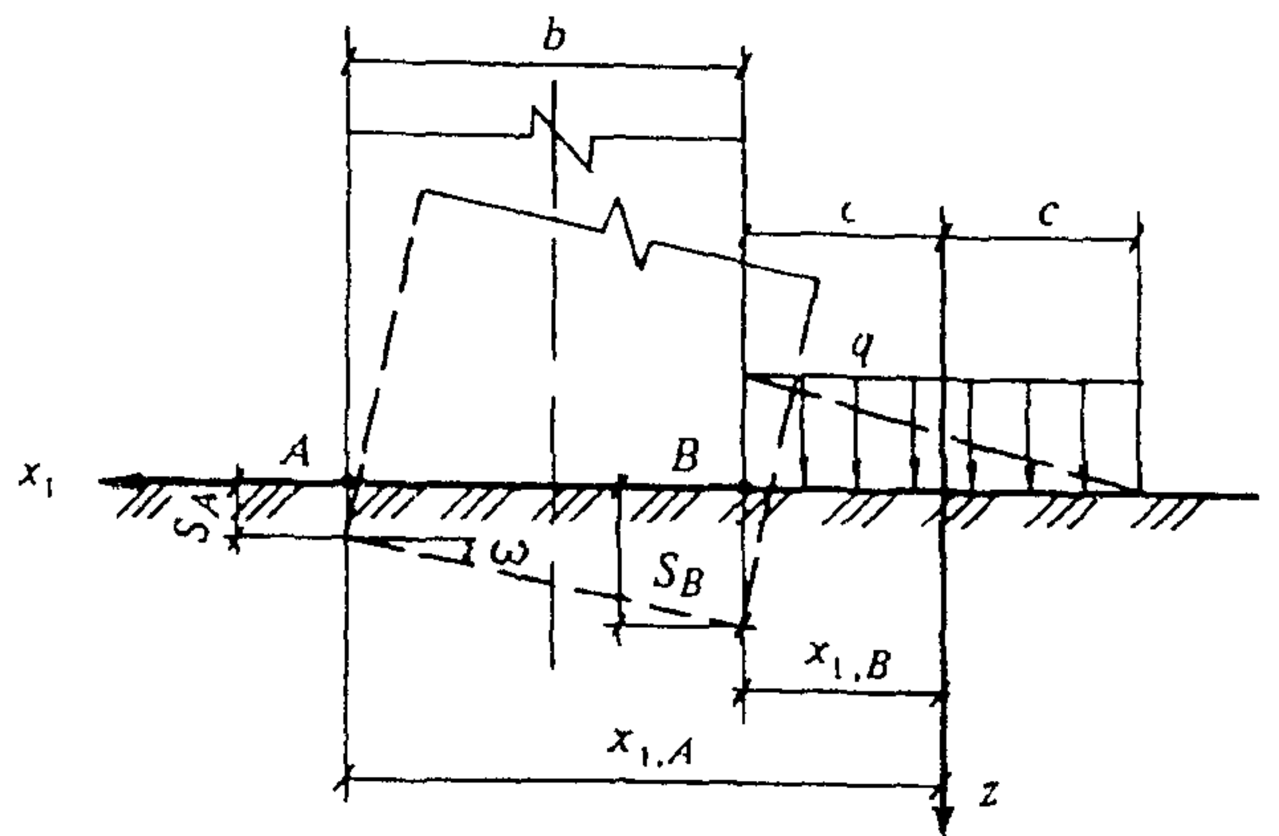
Черт. 4. Схема к определению крена сооружения от пригрузки
