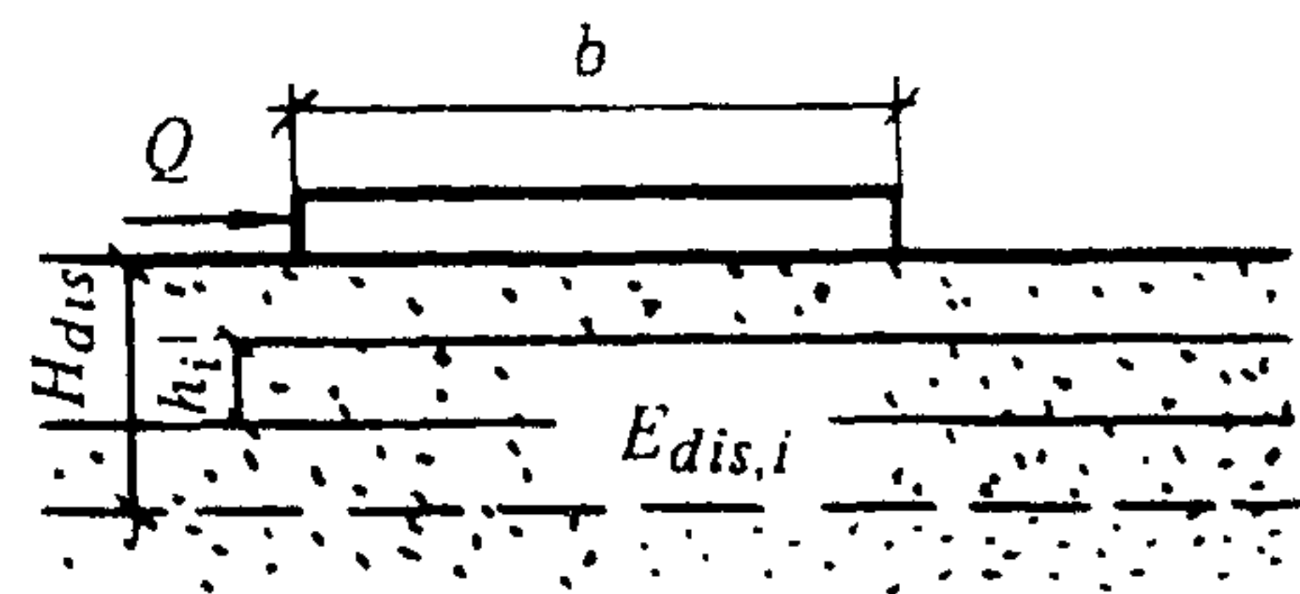
Черт. 1. Схемы к определению горизонтальных смещений сооружений
