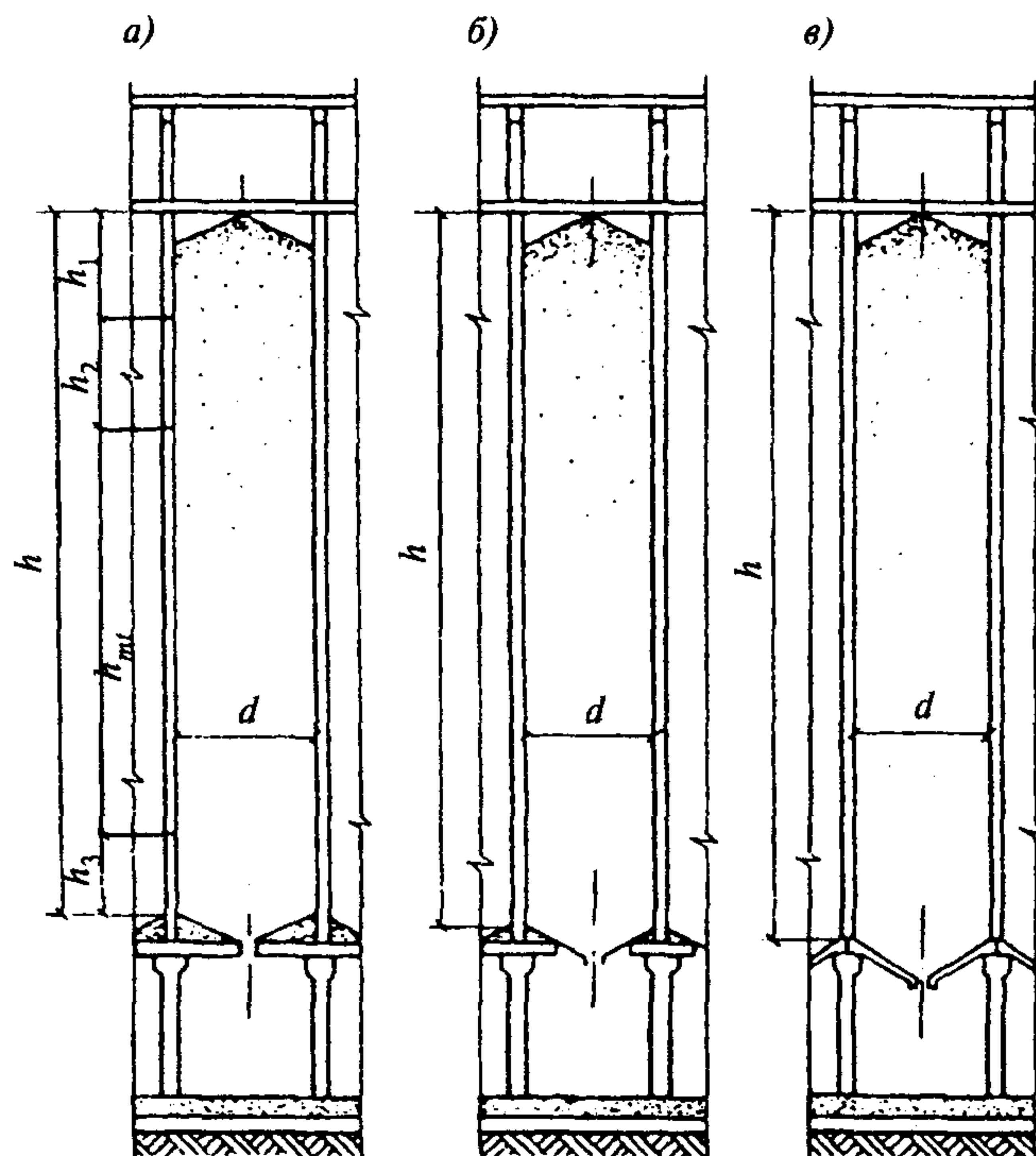
Черт. 1. Разрезы силосов
