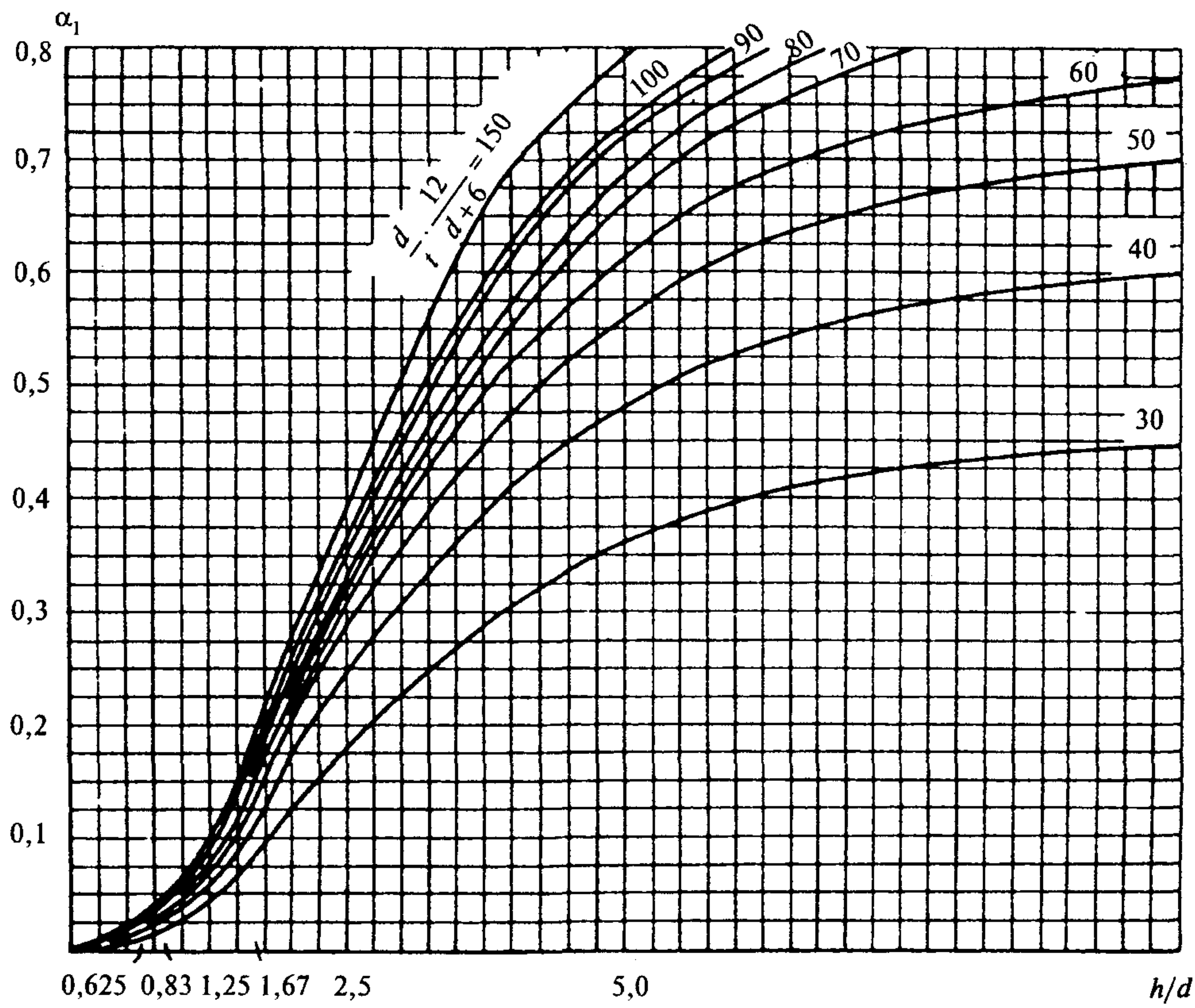
Черт. 4. Значения коэффициента \alpha_1
