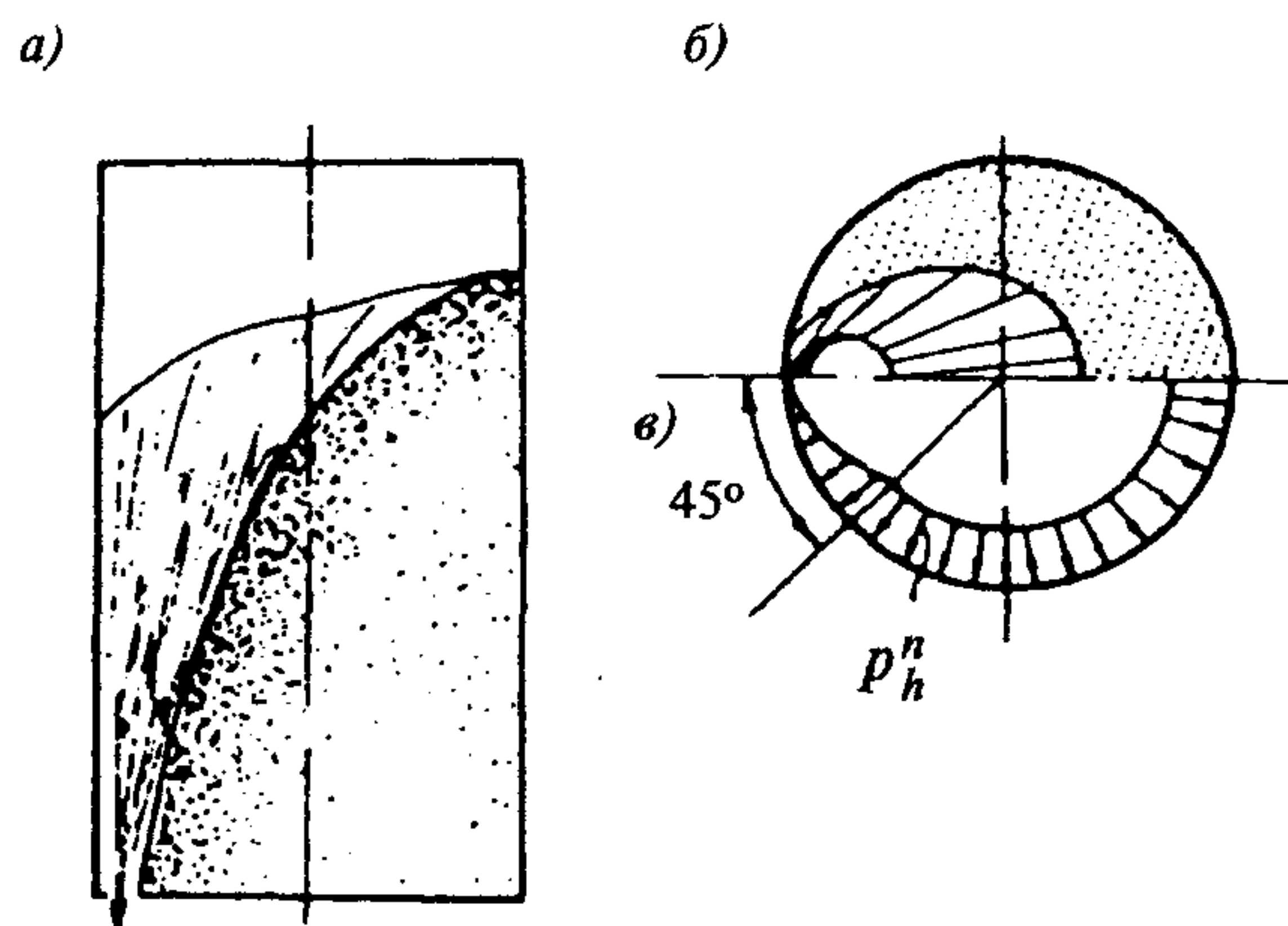
Черт. 3. Пристенный выпуск зерна
