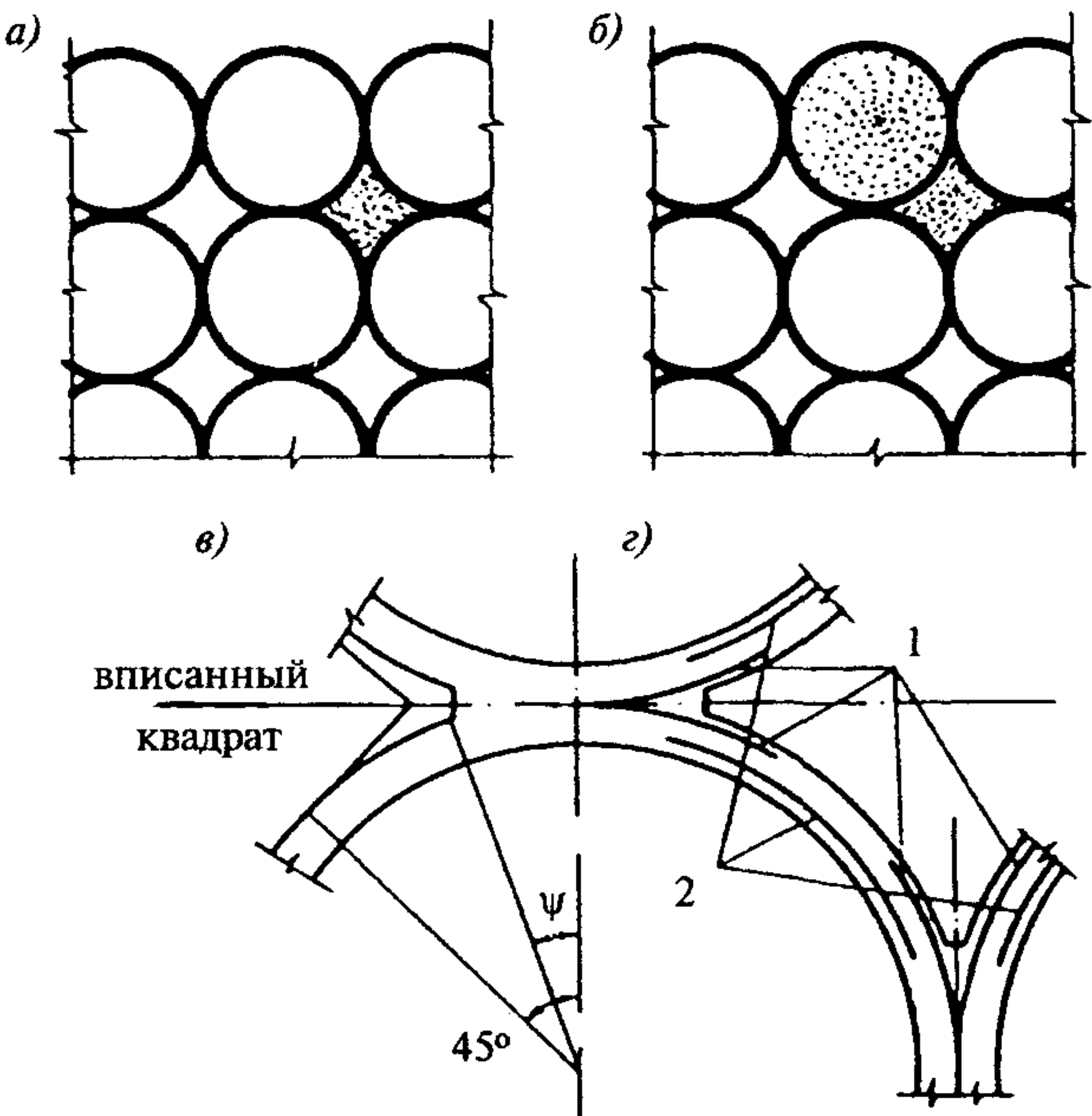
Черт. 6. К расчету звездочки
