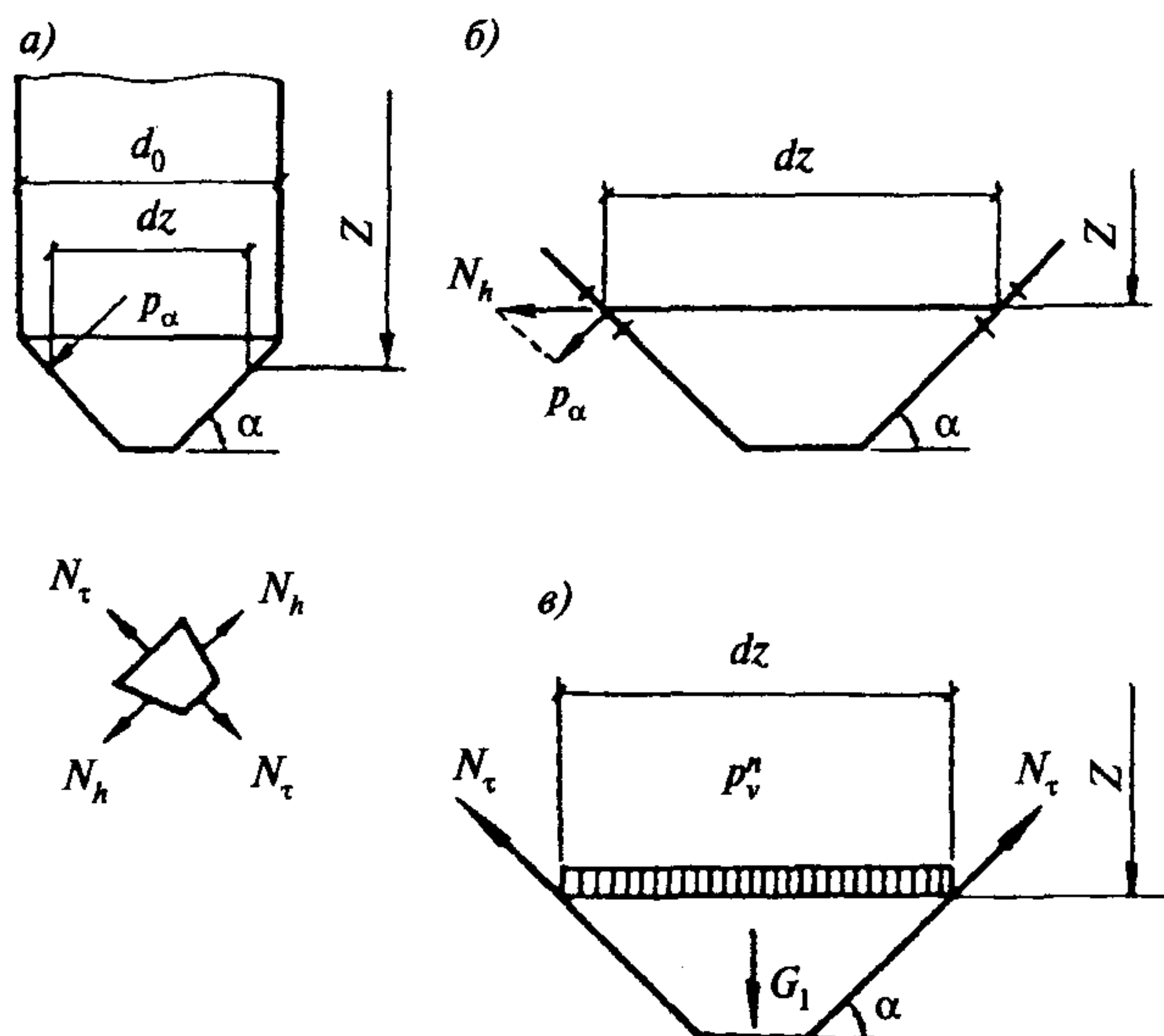
Черт. 7. Расчетные схемы конической воронки
