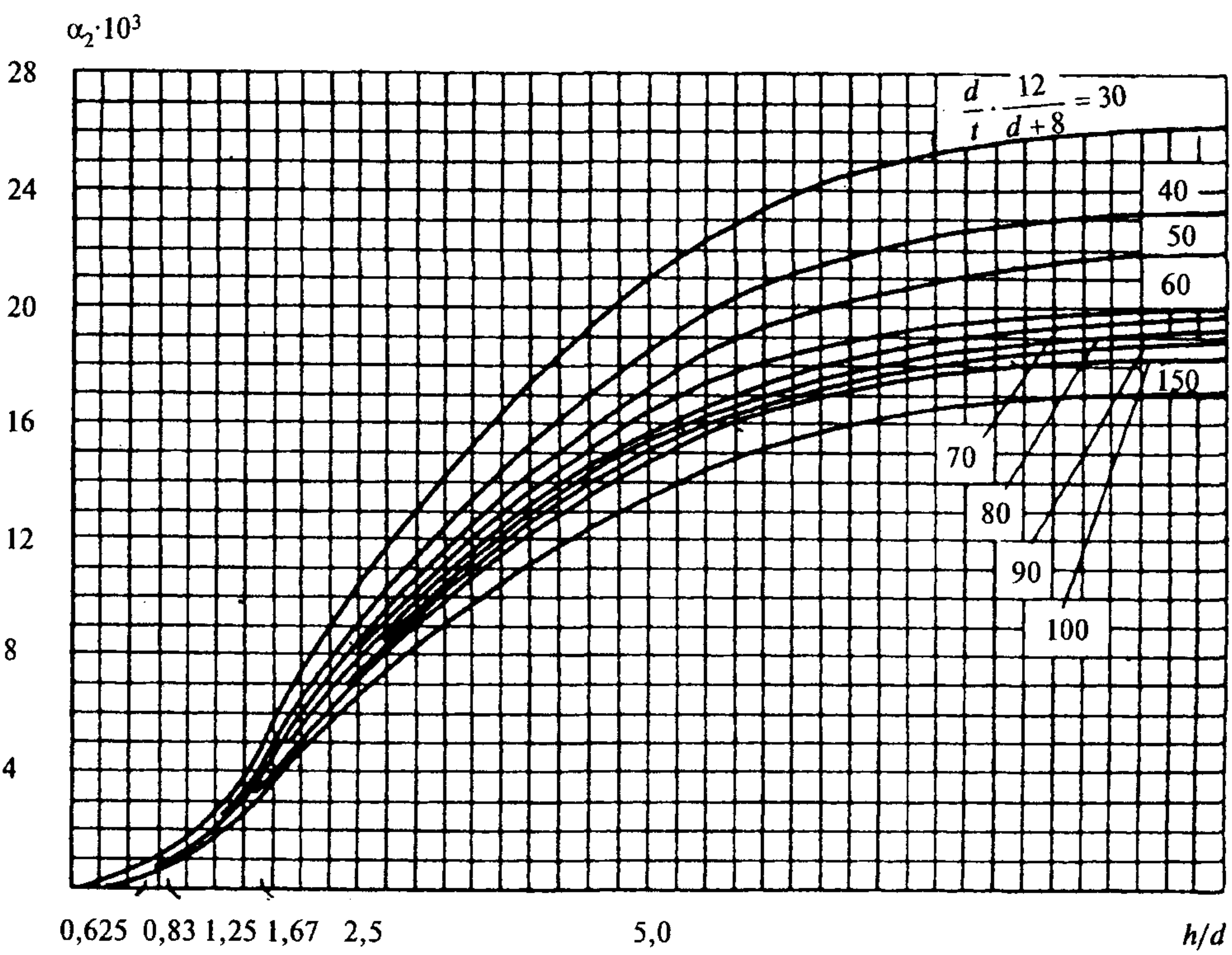
Черт. 5. Значения коэффициента \alpha_2
