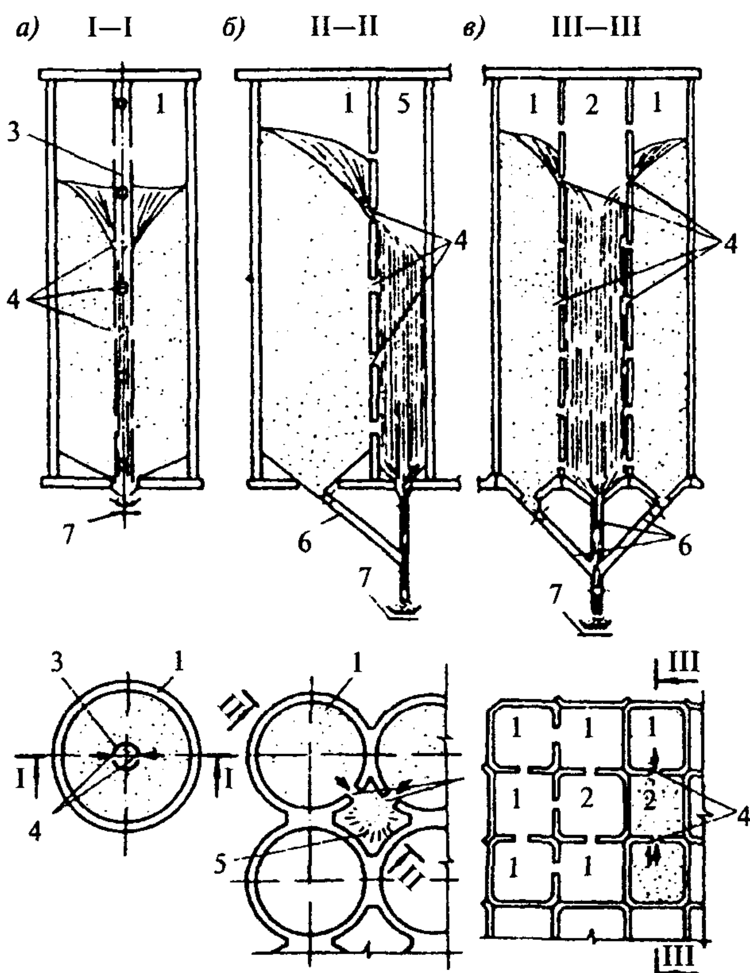
Черт. 2. Выпуск сыпучего материала из силоса
