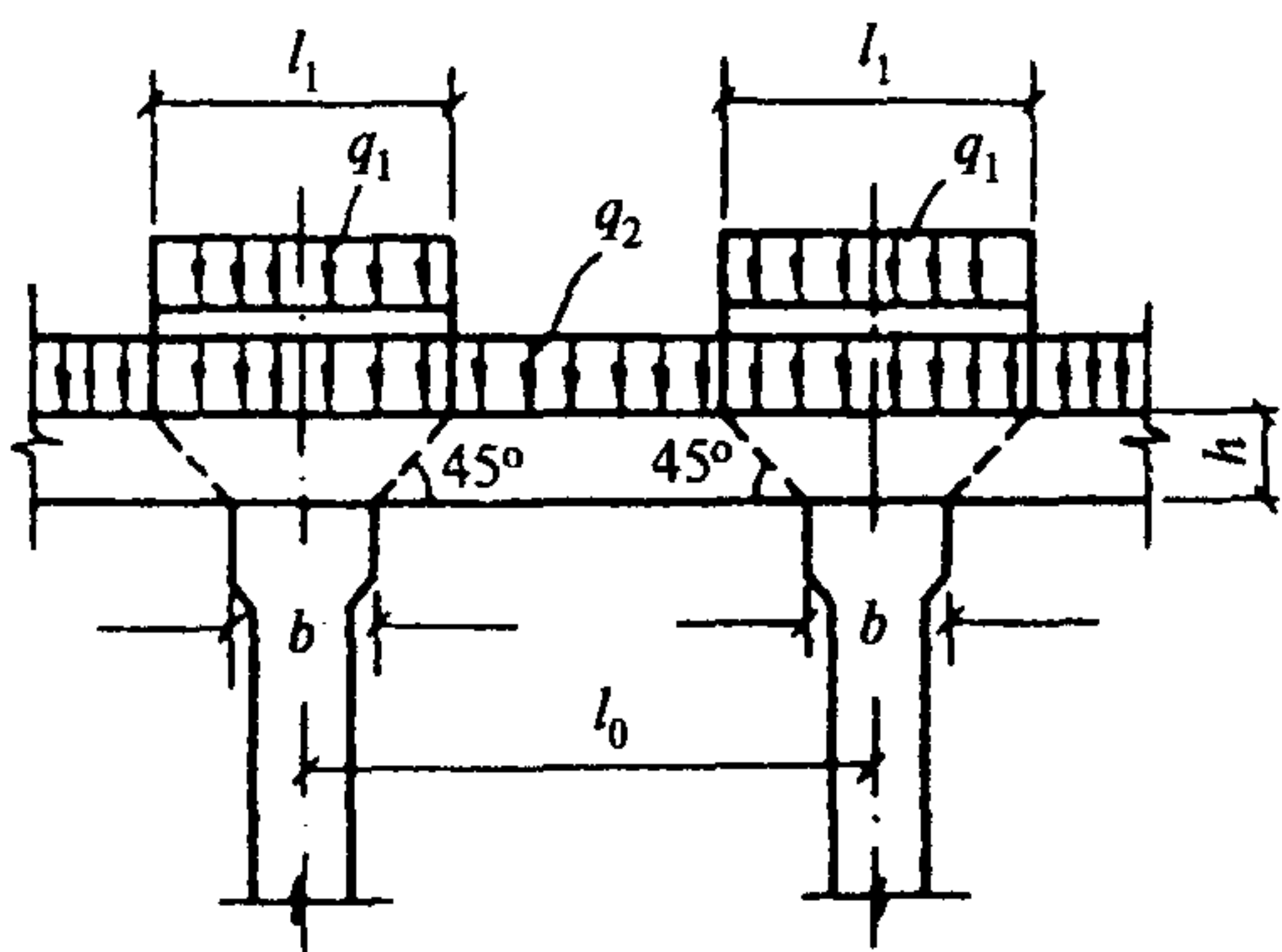
Черт. 8. Передача нагрузки от балки на колонну
