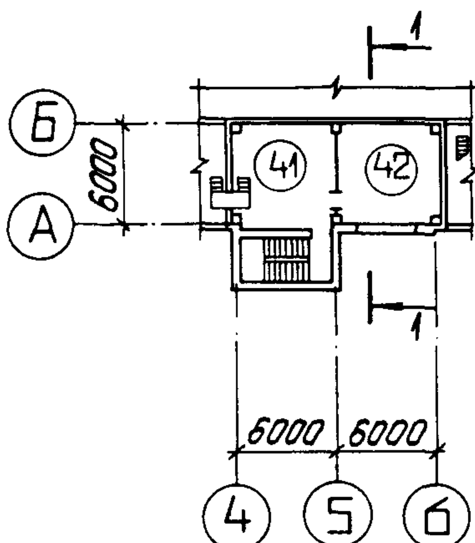
ПЛАН НА ОТМ. 18,600
