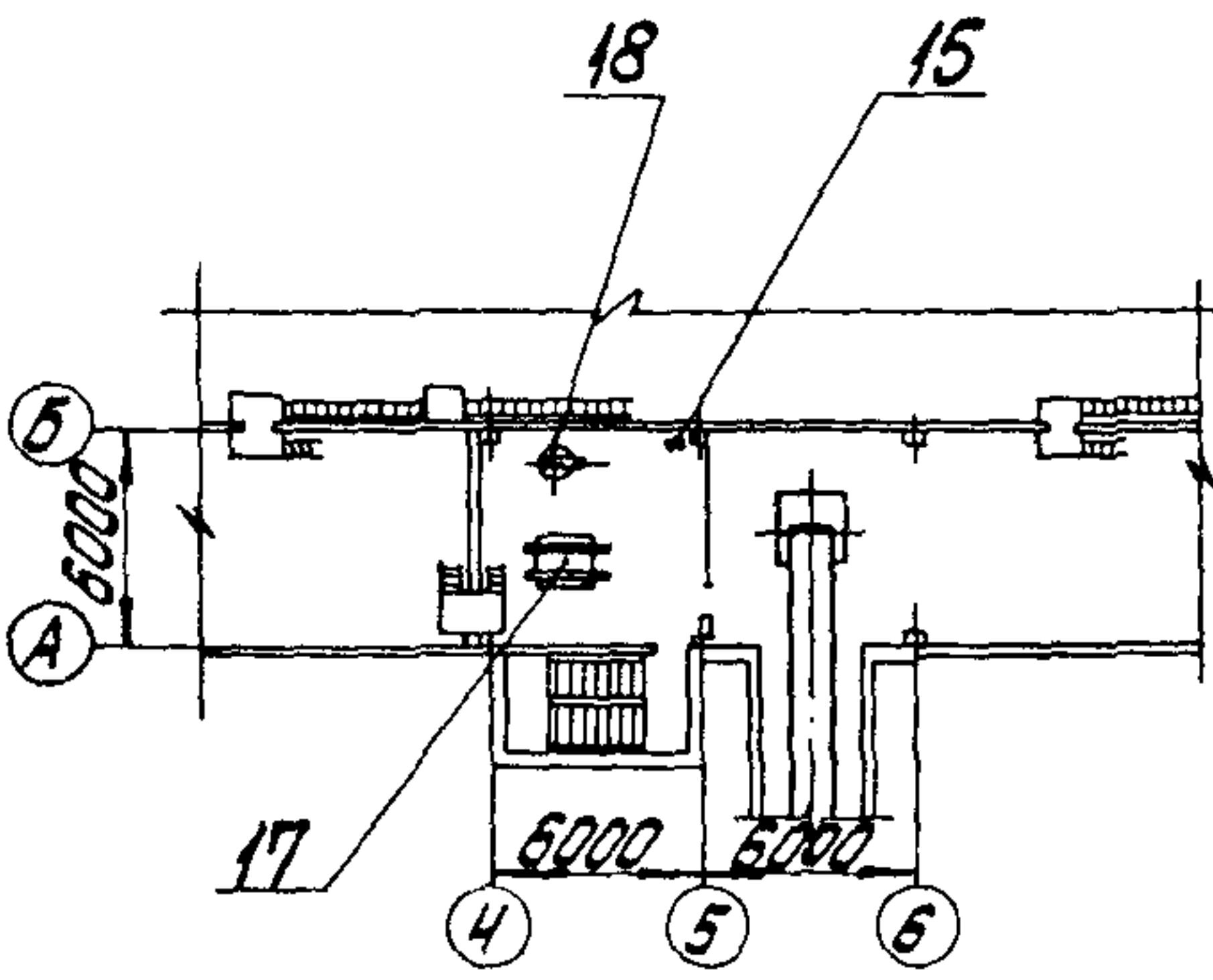
ПЛАН НА ОТМ. 18,600
