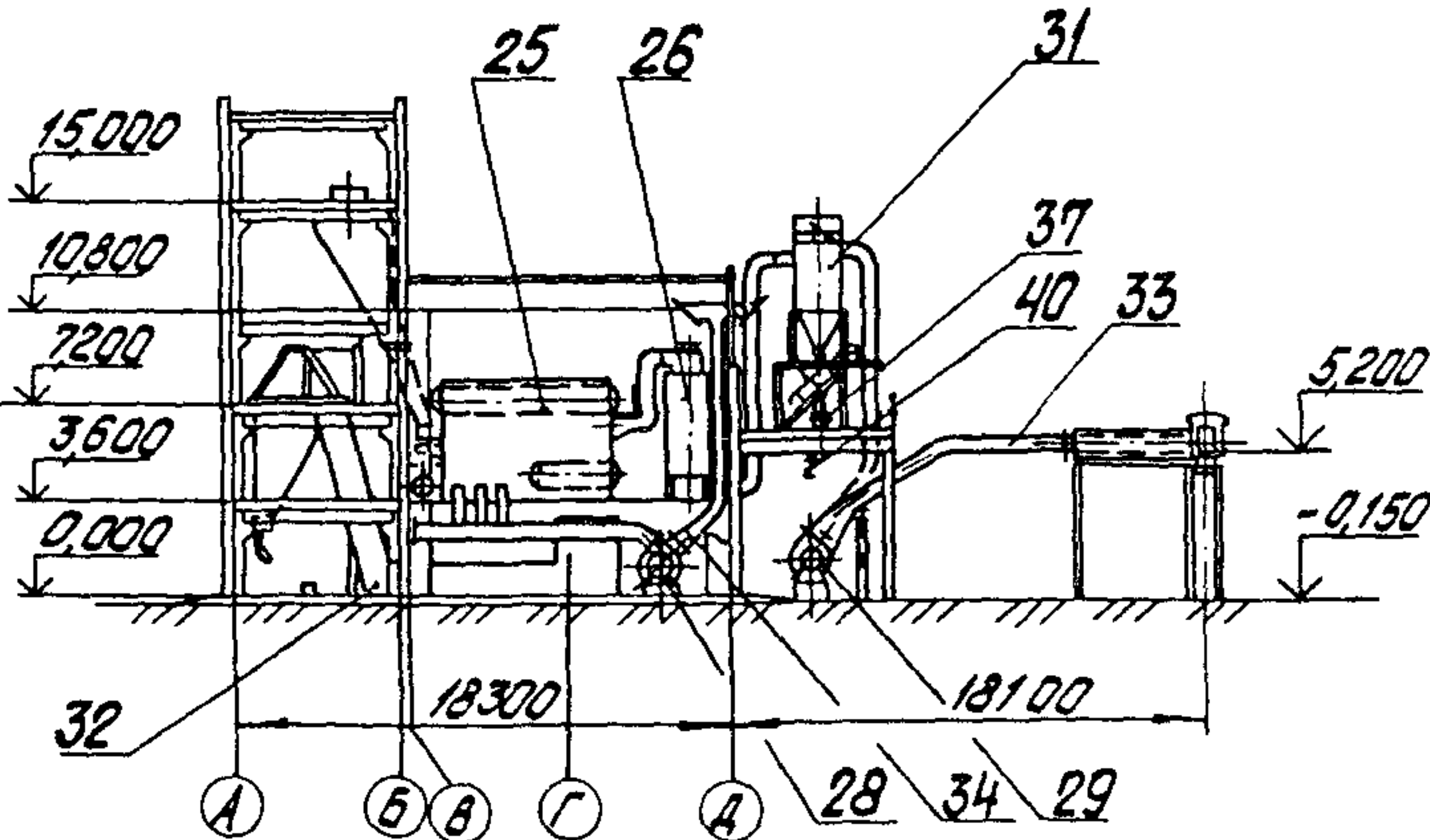
РАЗРЕЗ Б-Б
