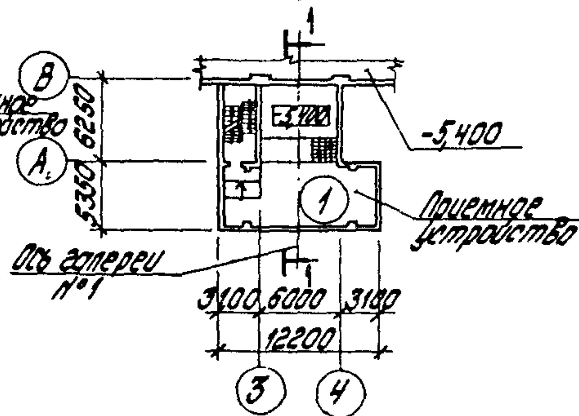
ПЛАН НА ОТМ. -3,400
