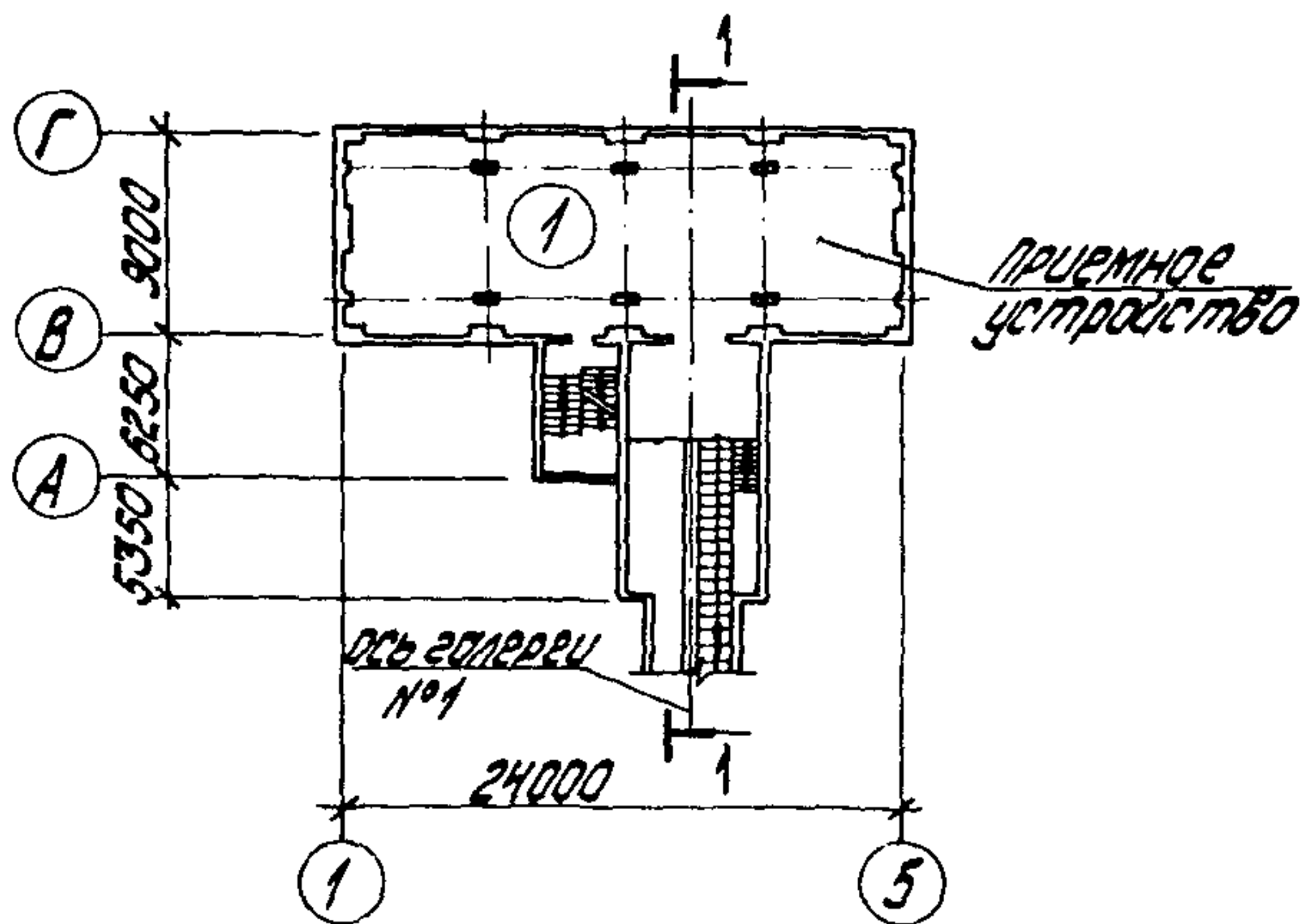
ПЛАН НА ОТМ. -10,800
