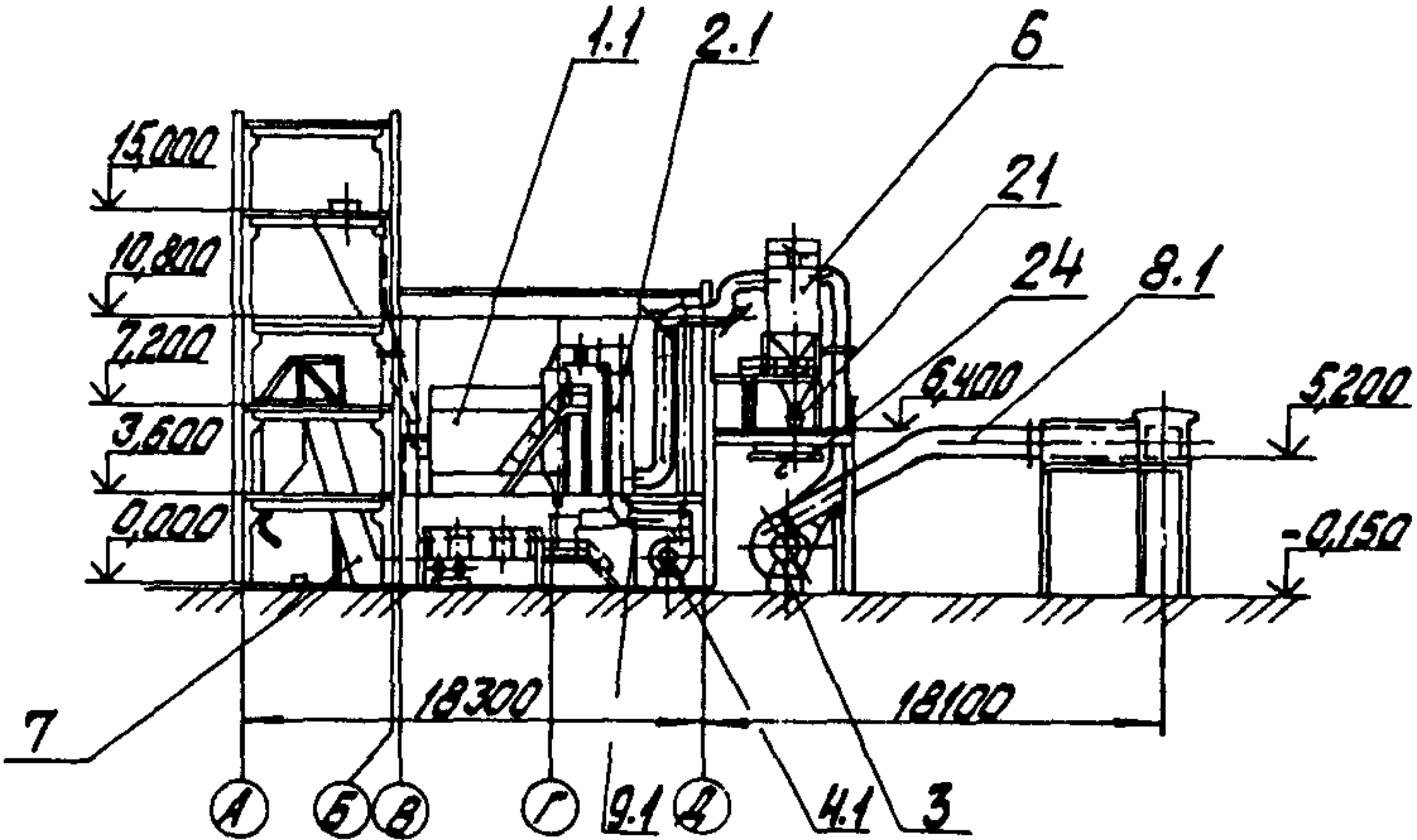
РАЗРЕЗ Г-Г
