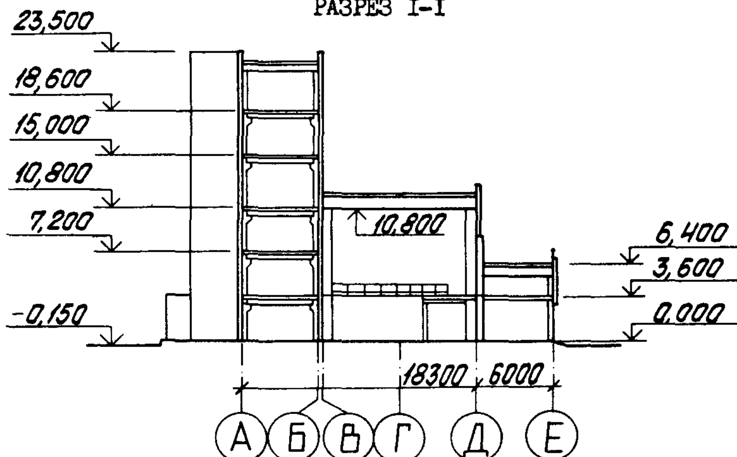
РАЗРЕЗ I-I
