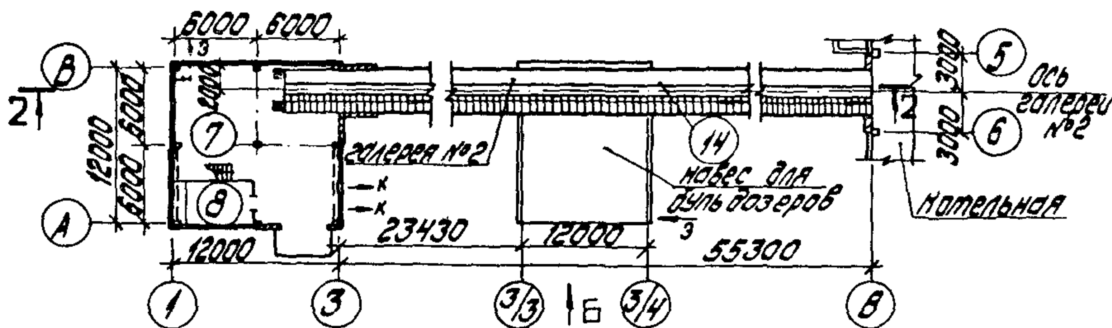
ПЛАН НА ОТМ. 0,000
