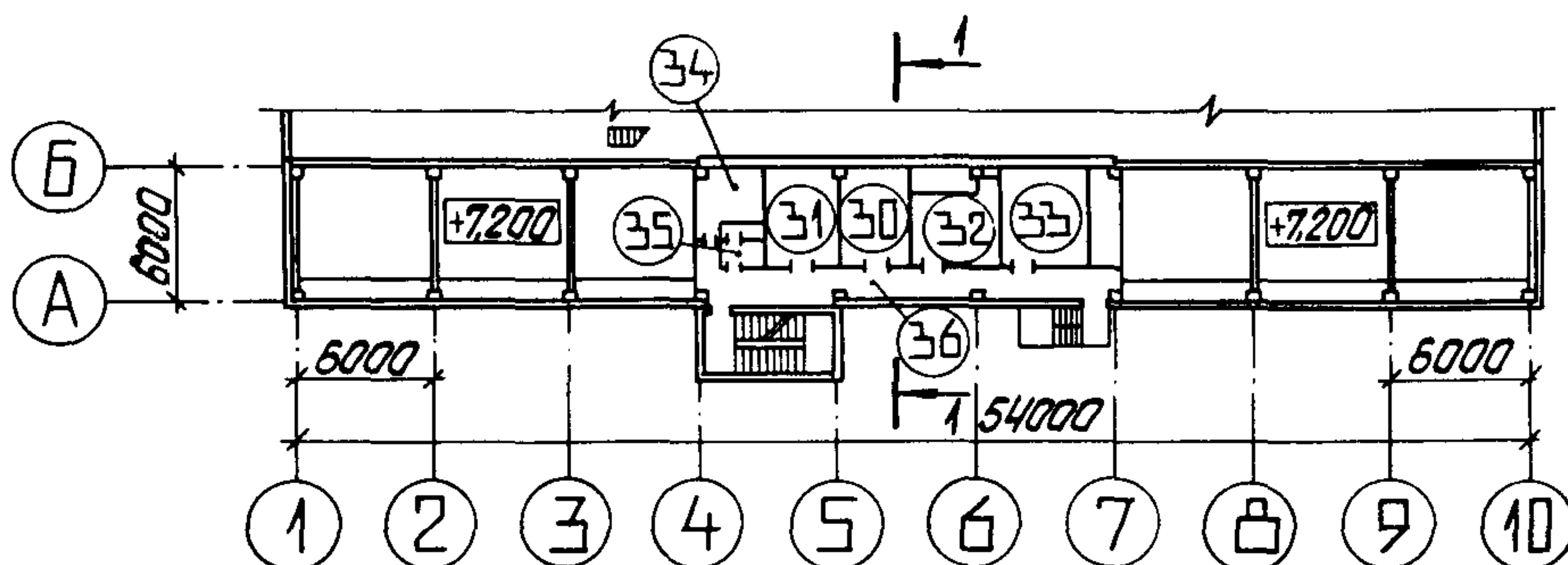
ПЛАН НА ОТМ. 10,800
