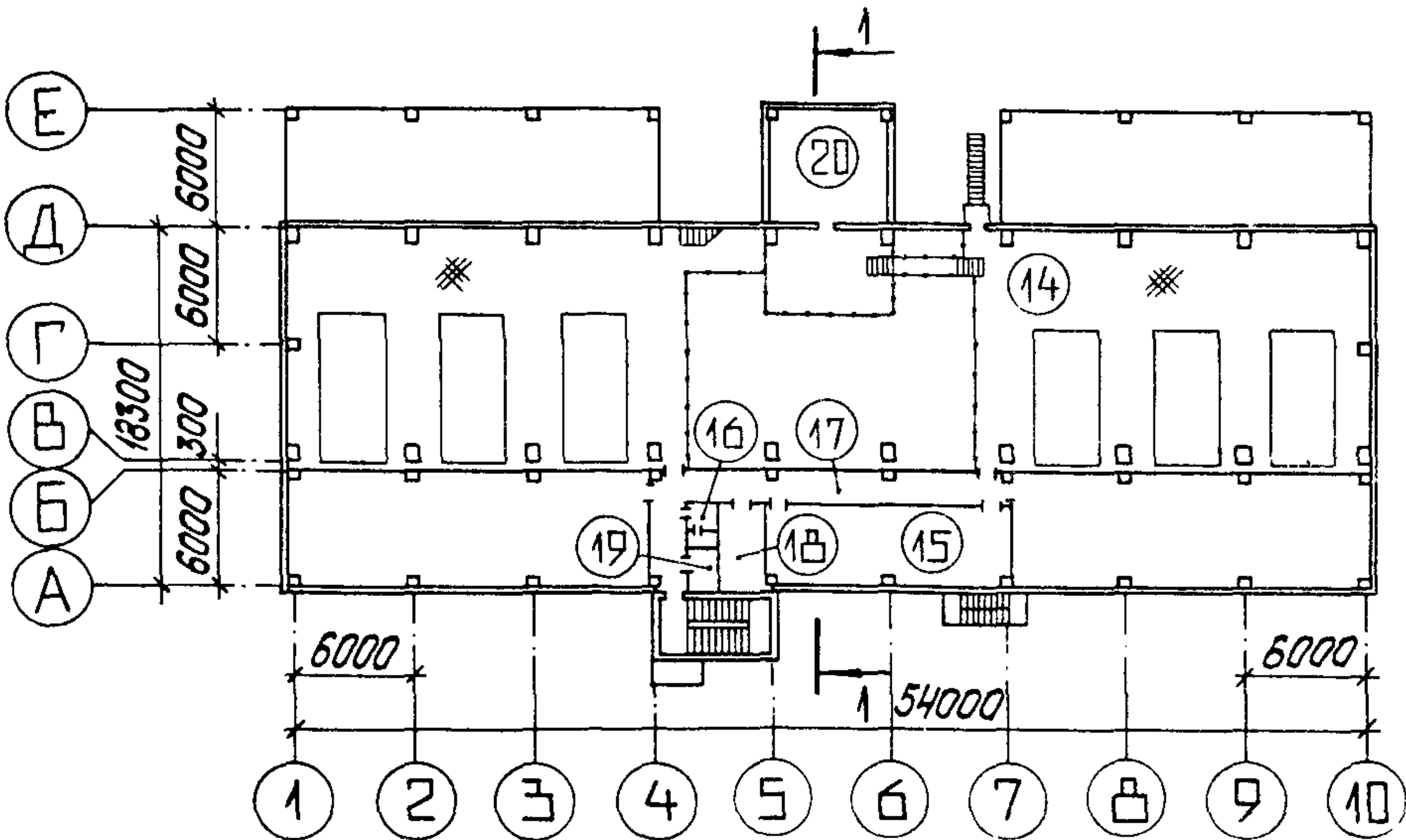
ПЛАН НА ОТМ. 3,600
