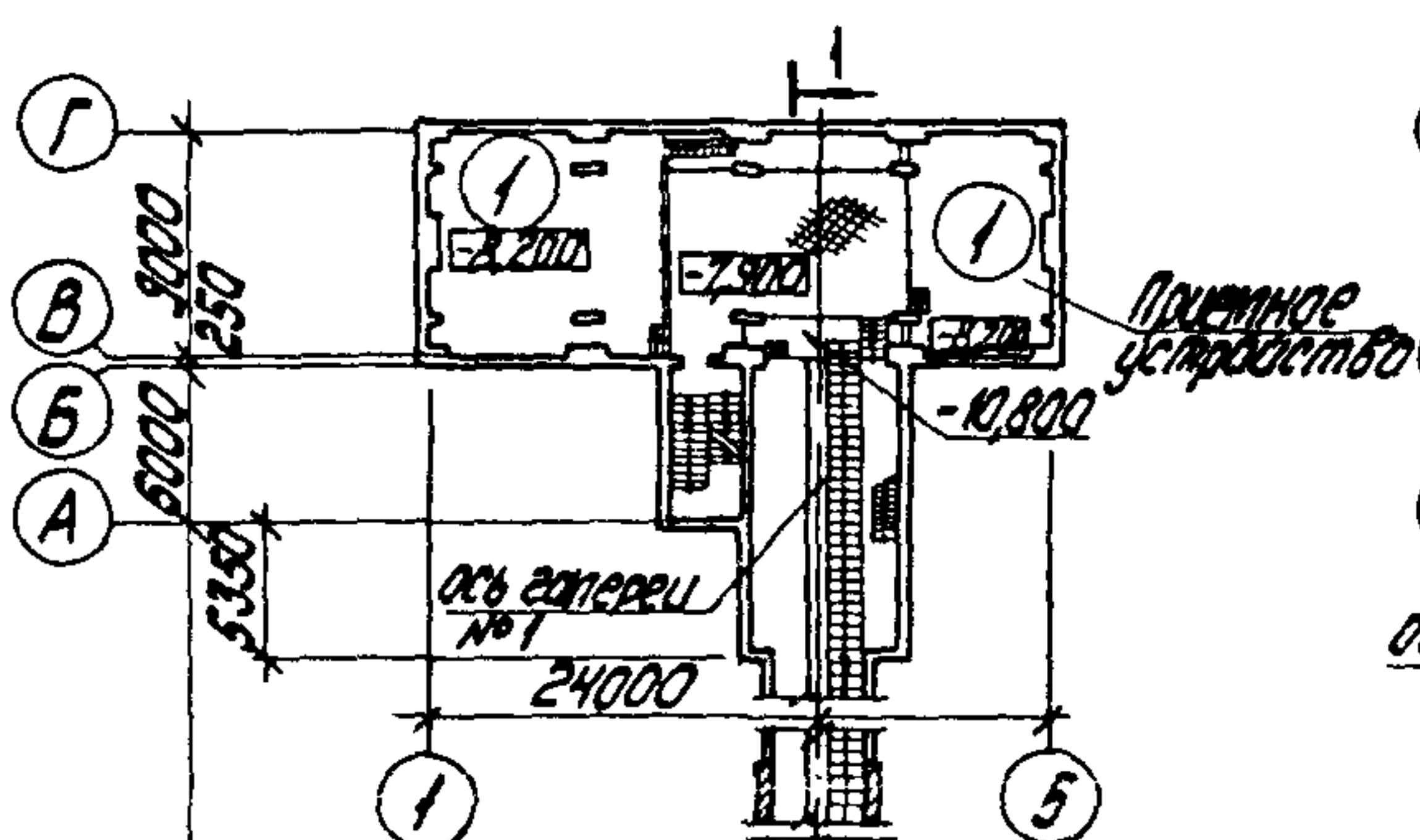
ПЛАН НА ОТМ. -8,200; -7,900; +11,400
