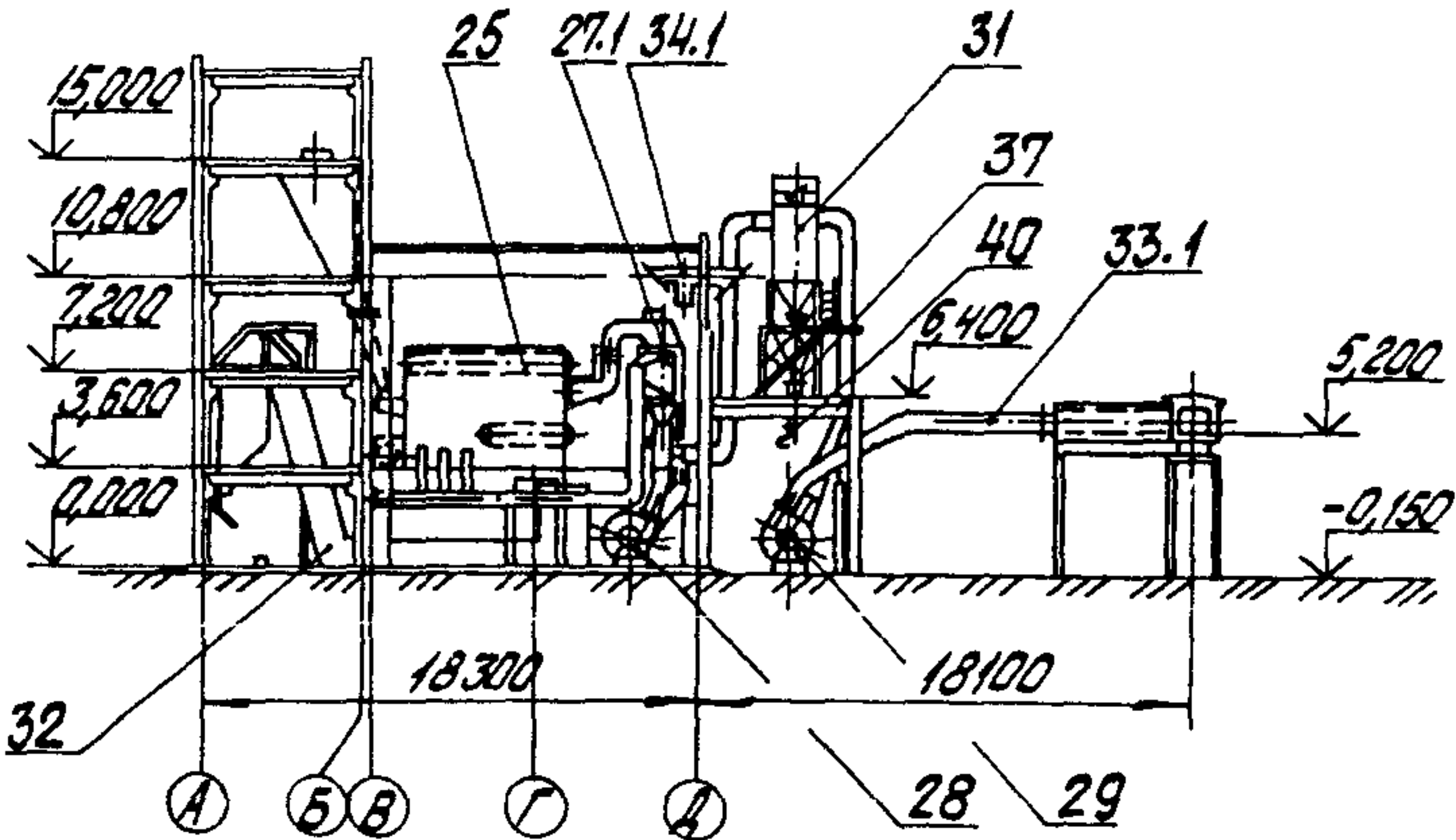
РАЗРЕЗ В-В
