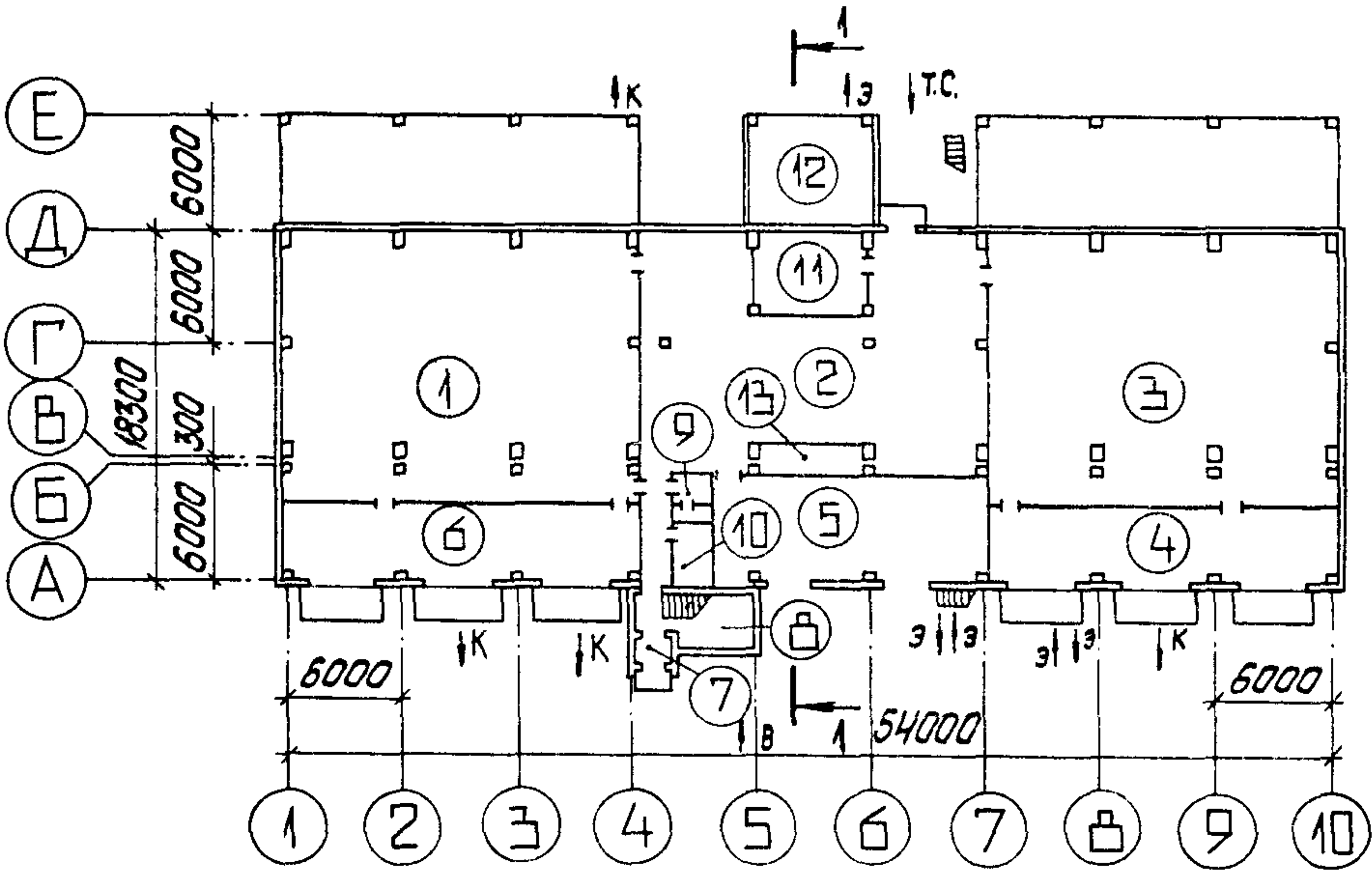
ПЛАН НА ОТМ. 0,000
