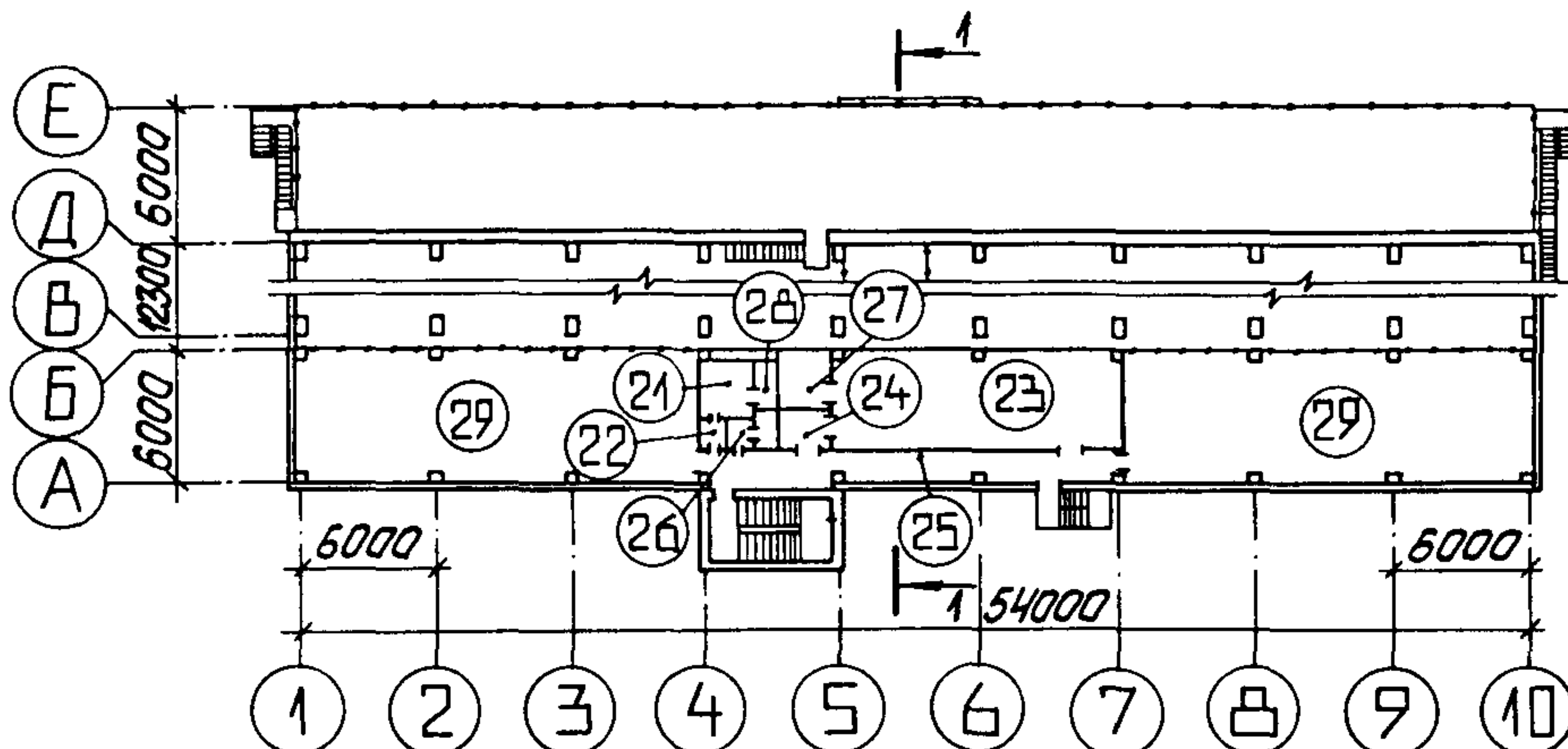
ПЛАН НА ОТМ. 10,800
