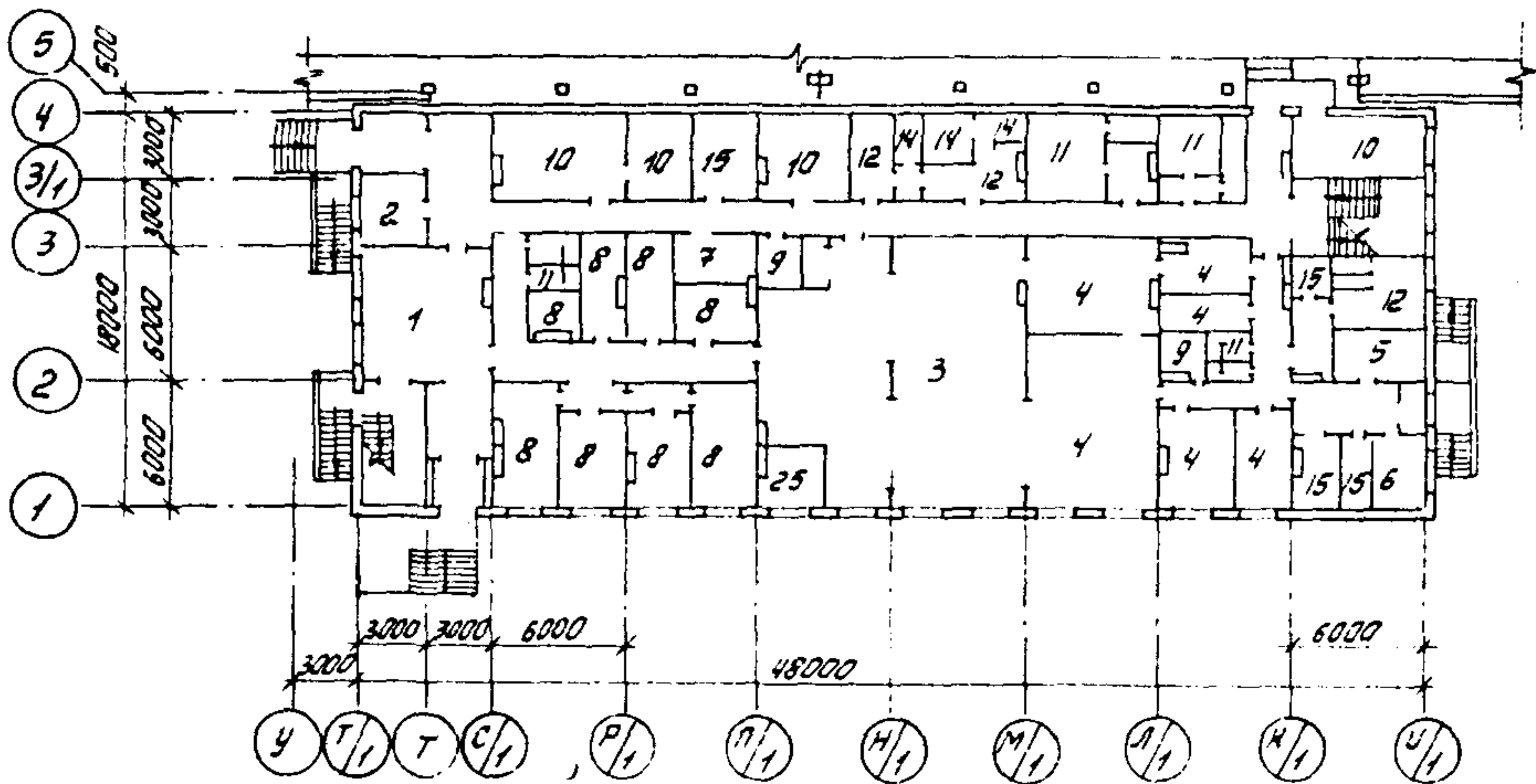
ПЛАН НА ОТМ. І,050
