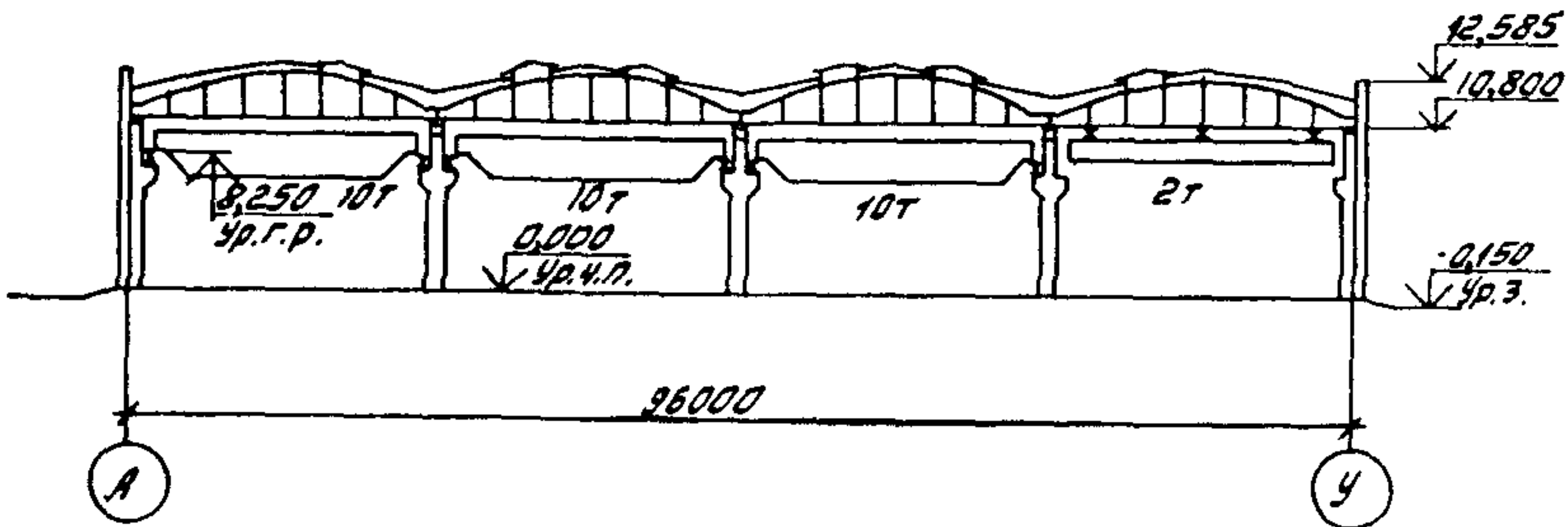
РАЗРЕЗ I-I
