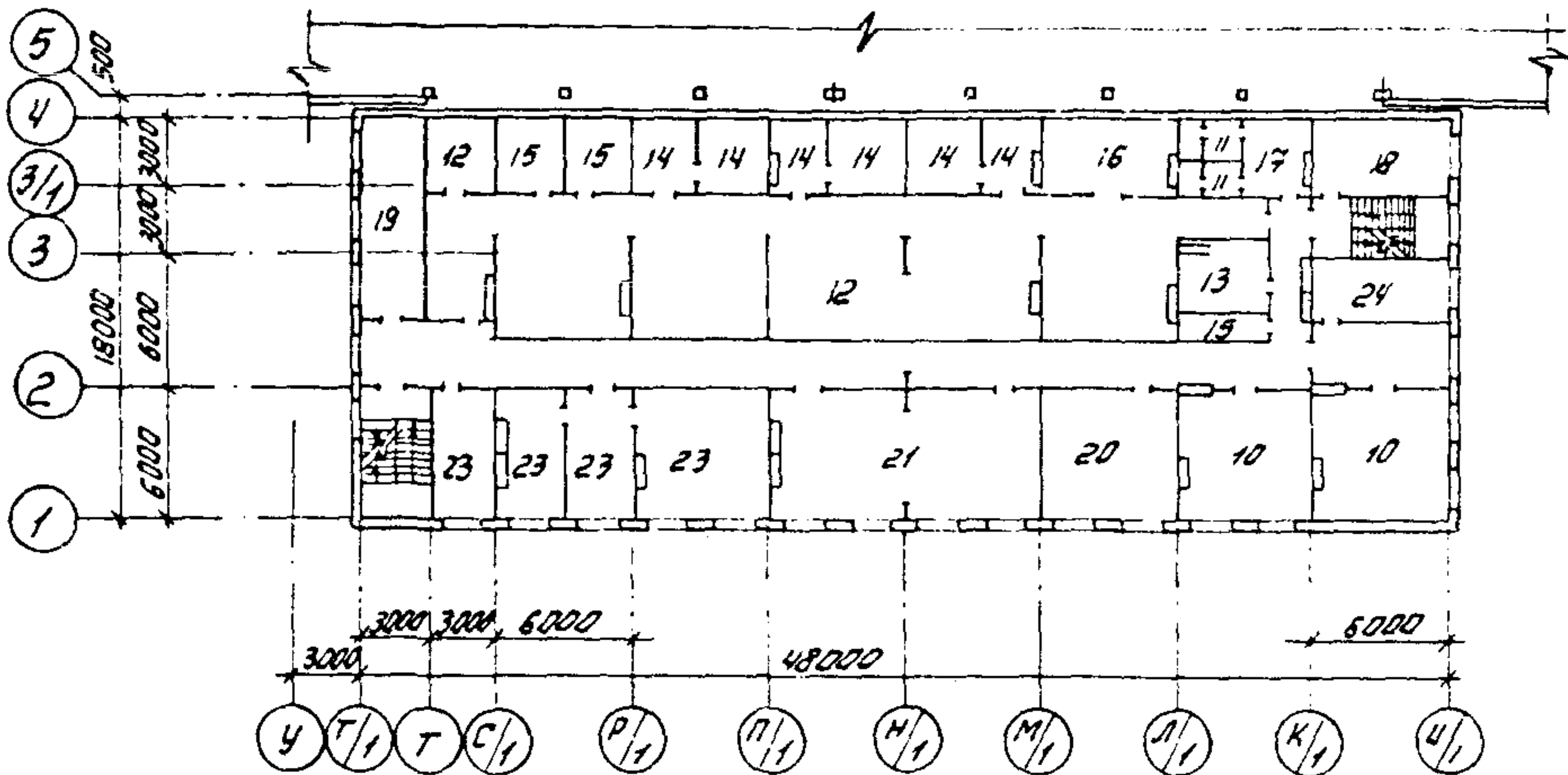
ПЛАН НА ОТМ. 4,050
