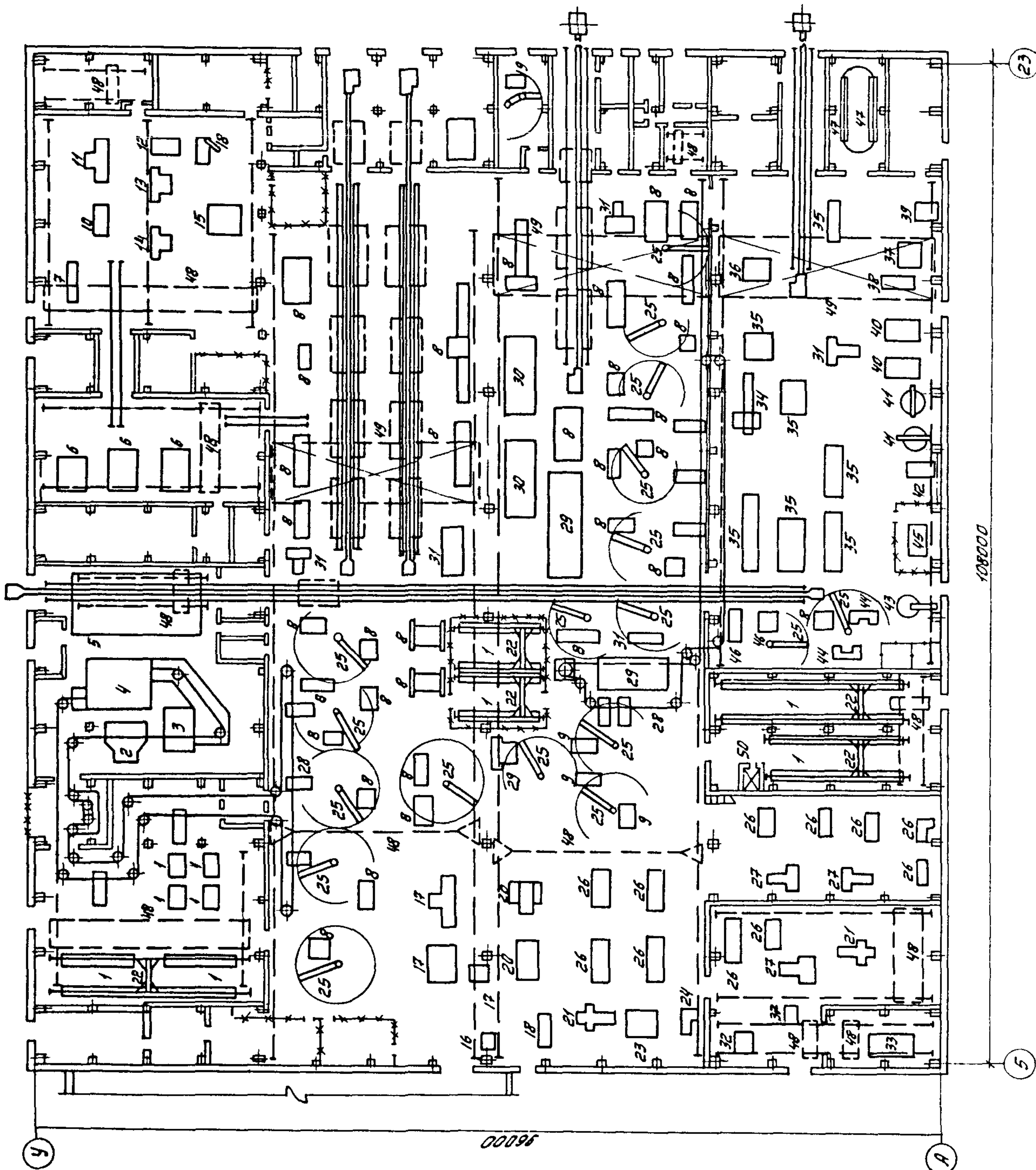
ПЛАН РАЗМЕЩЕНИЯ ТЕХНОЛОГИЧЕСКОГО ОБОРУДОВАНИЯ НА ОТМ. 0,000
