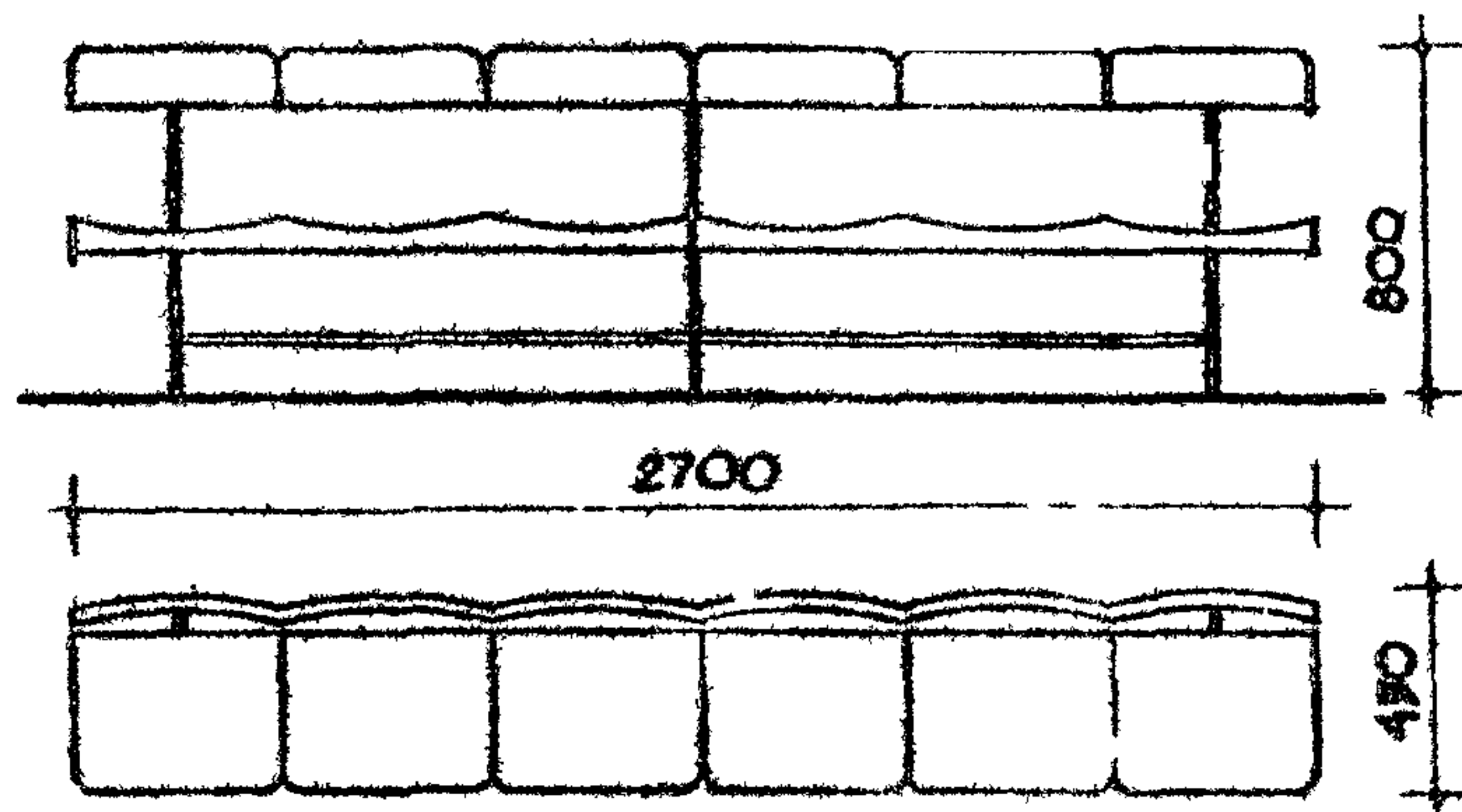
9) СКАМЬЯ СКЛАДЫВАЮЩАЯСЯ
