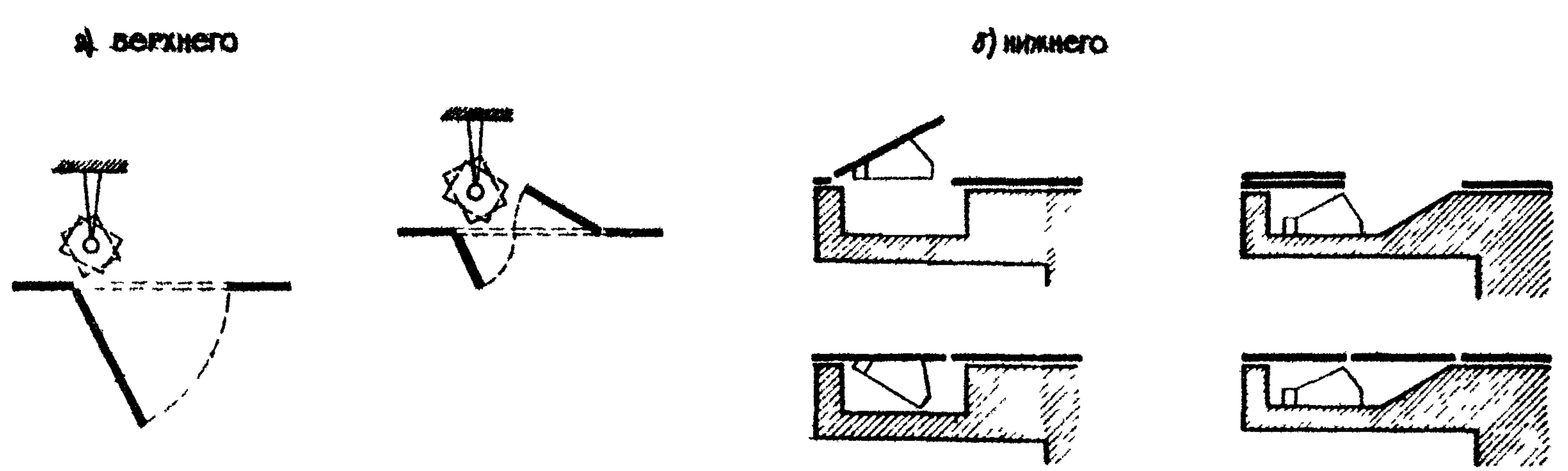
СХЕМЫ ВАРИАНТОВ ТРАНСФОРМАЦИИ ОСВЕЩЕНИЯ:
