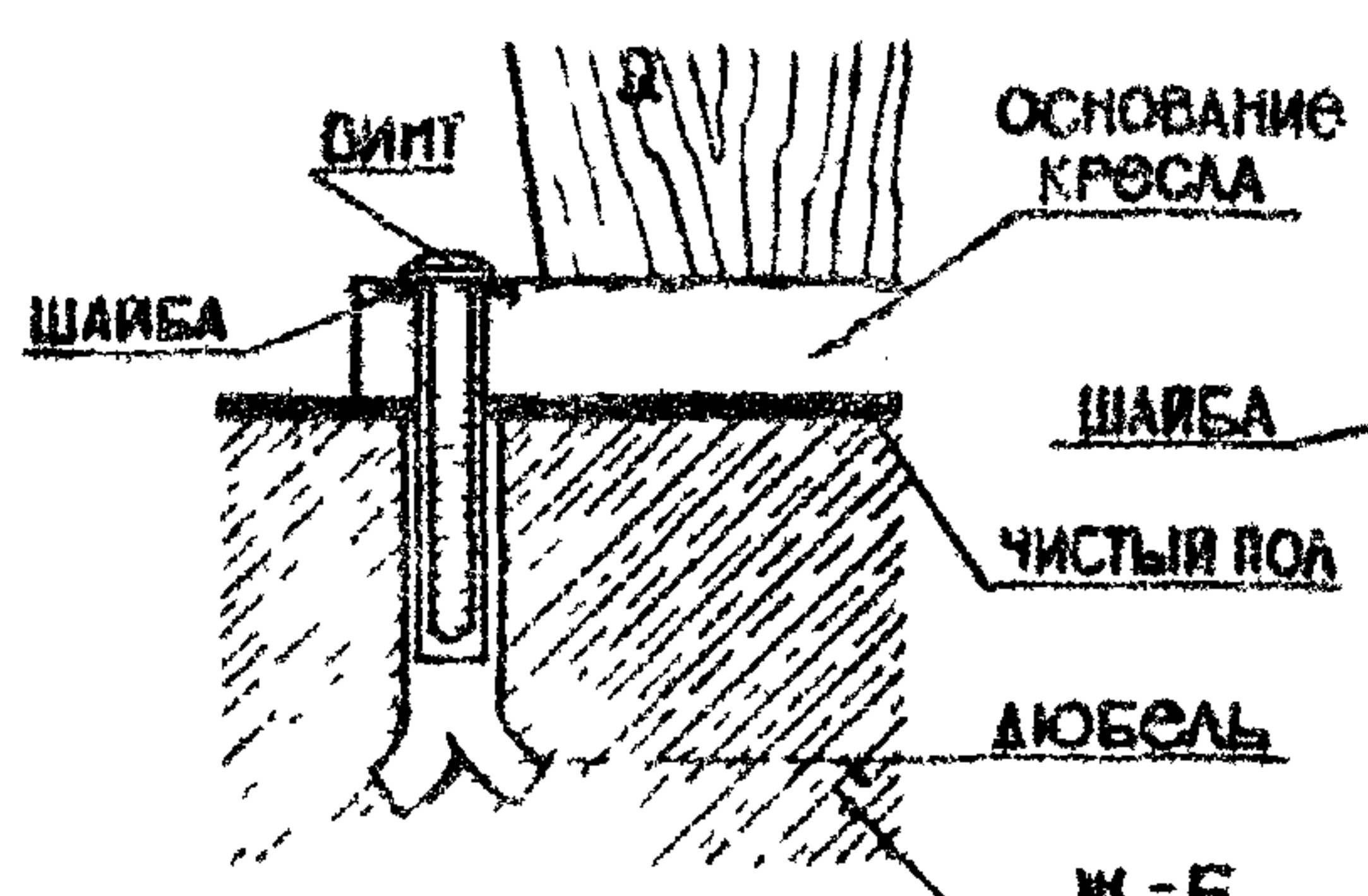
а КРЕПЛЕНИЕ КРЕСЛА К ПОЛУ ПРИ ПОМОЩИ ДЮБЕЛЕЙ.
