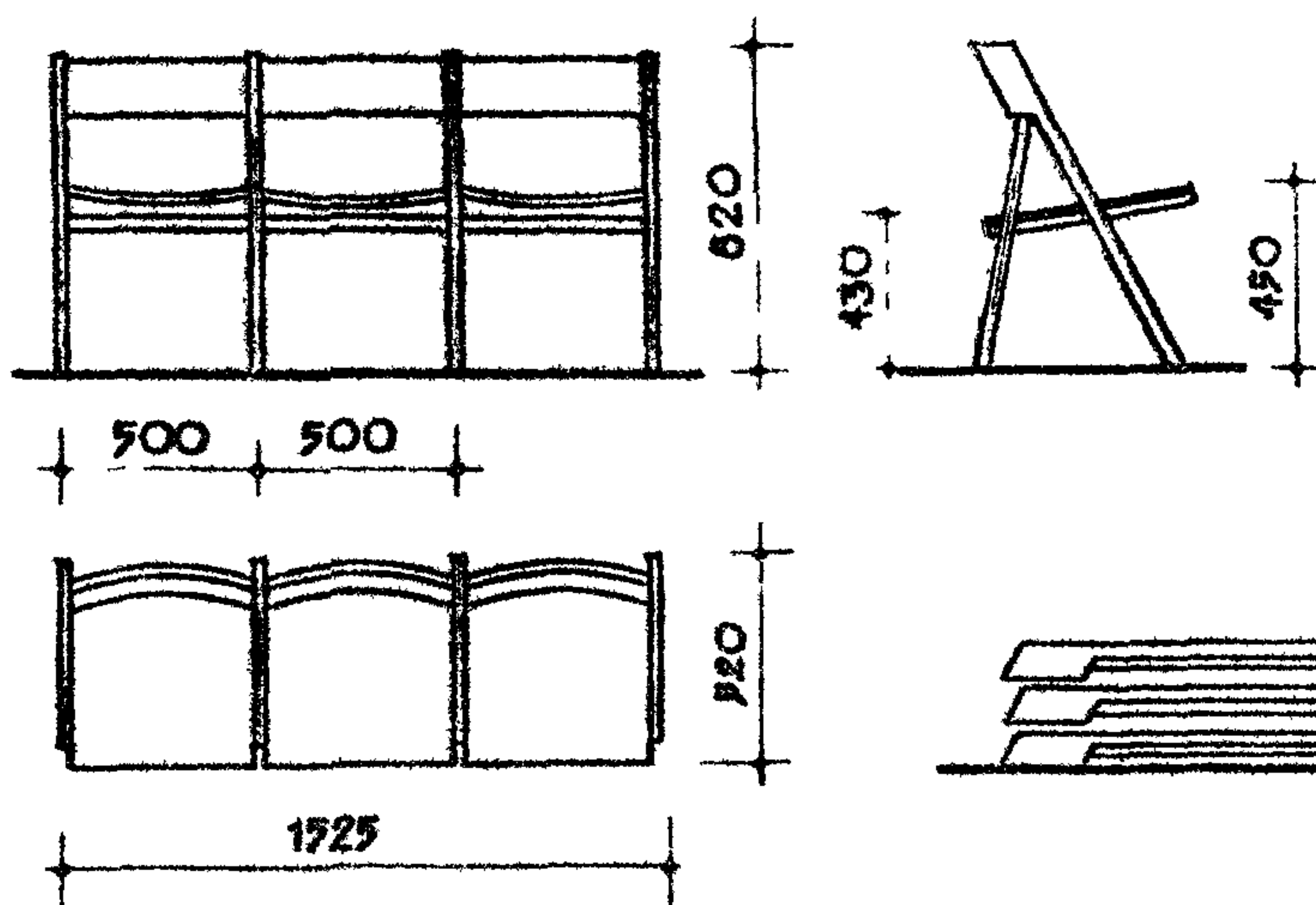
11) СЕКЦИЯ СКЛАДНЫХ СТУЛЬЕВ
