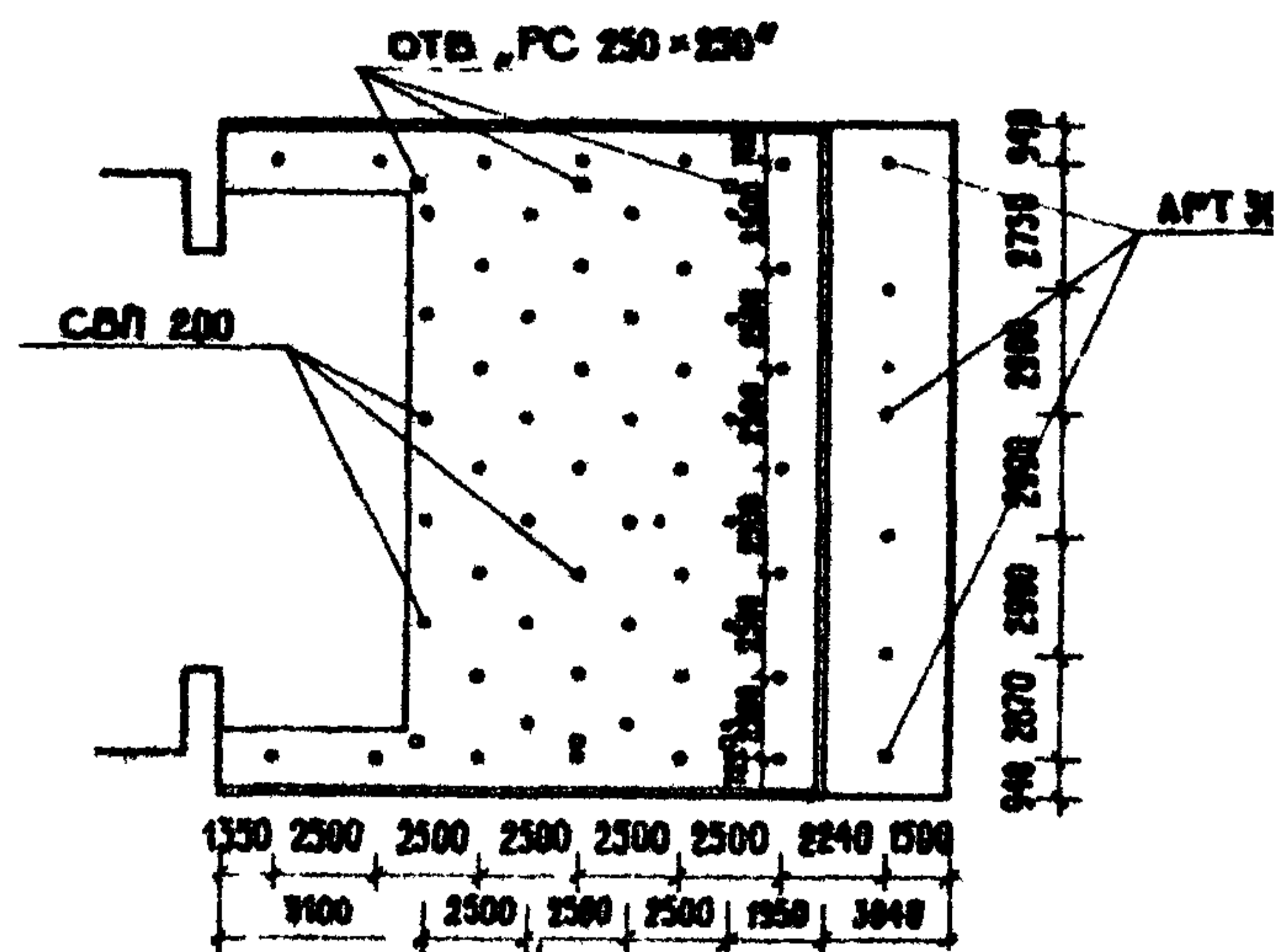
ПЛАН РАЗБИВКИ СВЕТИЛЬНИКОВ
