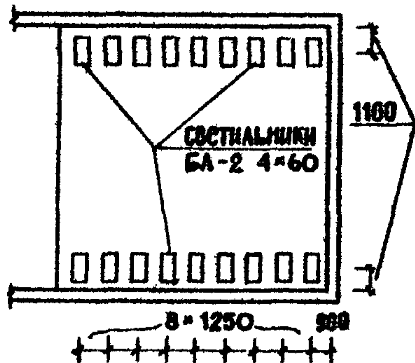
ПЛАН РАЗБИВКИ СВЕТИЛЬНИКОВ
