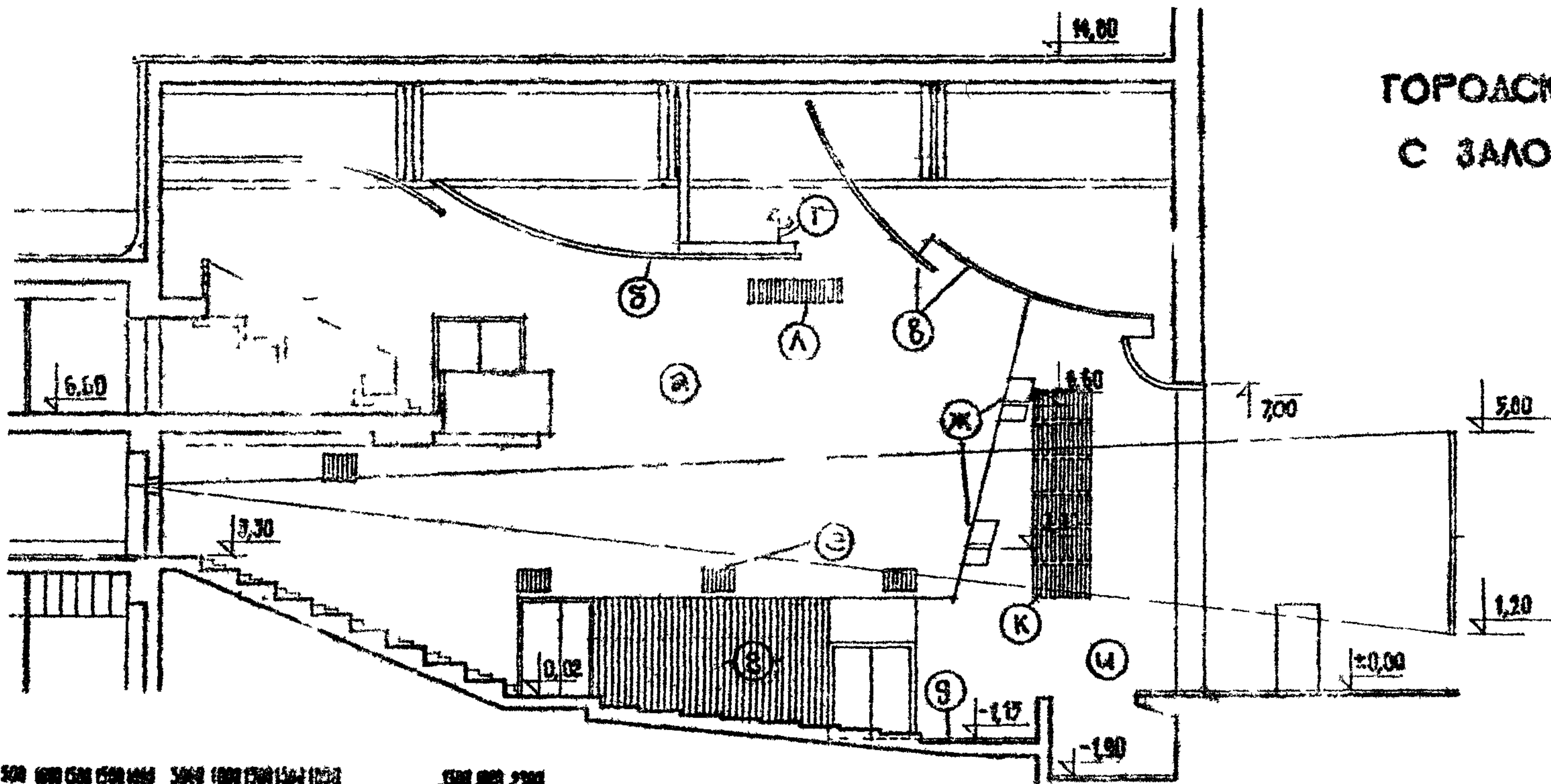
РАЗРЕЗ по А-А
