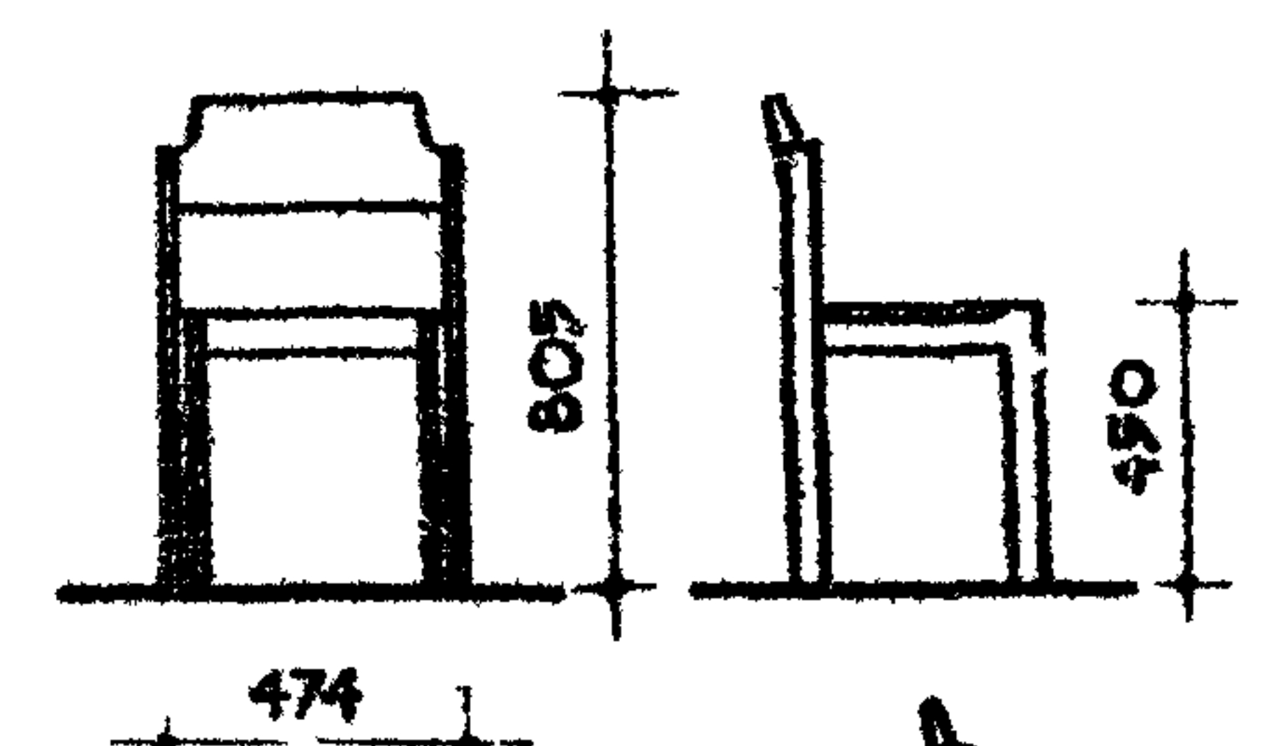
12) СЕКЦИЯ СКЛАДИРУЕМЫХ СТУЛЬЕВ С ОТКИДНЫМ СИДЕНЬЕМ
