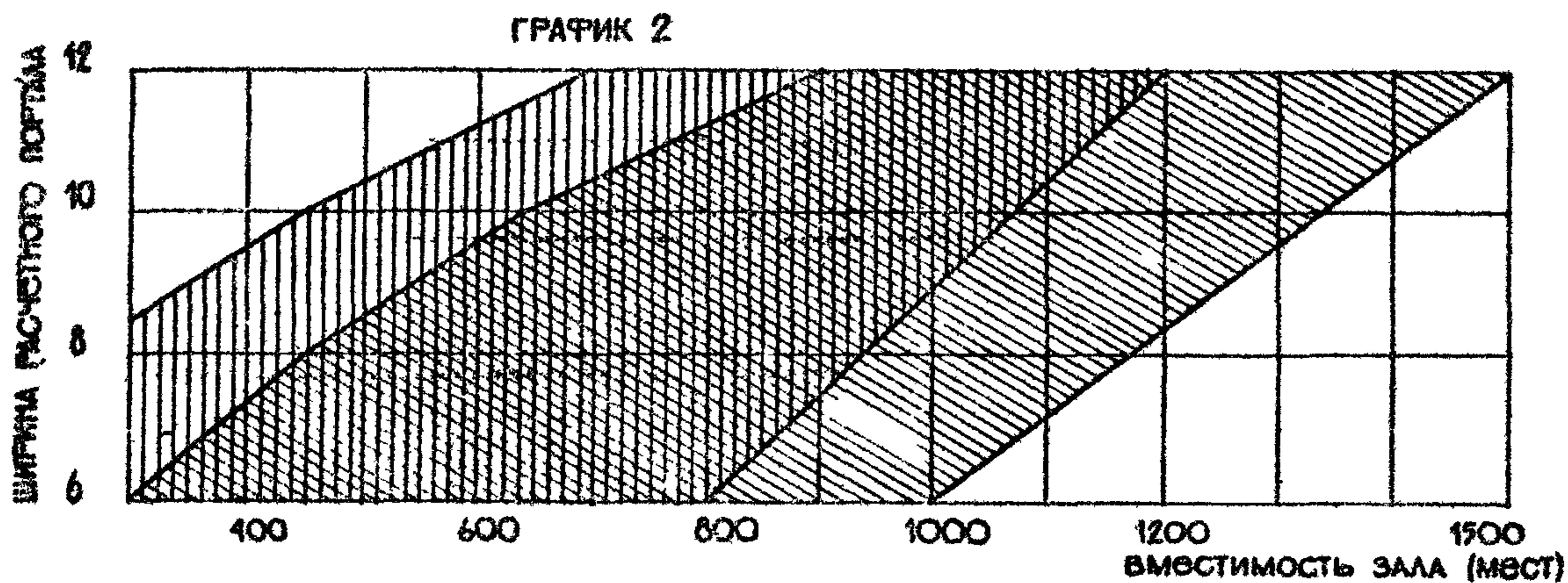
ГРАФИК 2 - ОБЩИЙ СЛУЧАЙ ДЛЯ ПРЯМОУГОЛЬНЫХ ЗАЛОВ.
