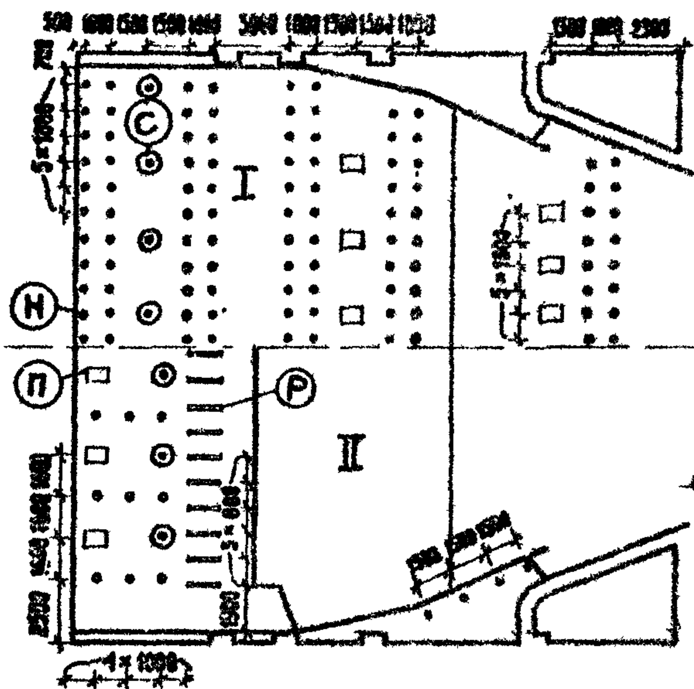
И - ПЛАН РАЗЕШКИ СВЕТИЛЬНИКОВ НАД ЗАЛОМ
