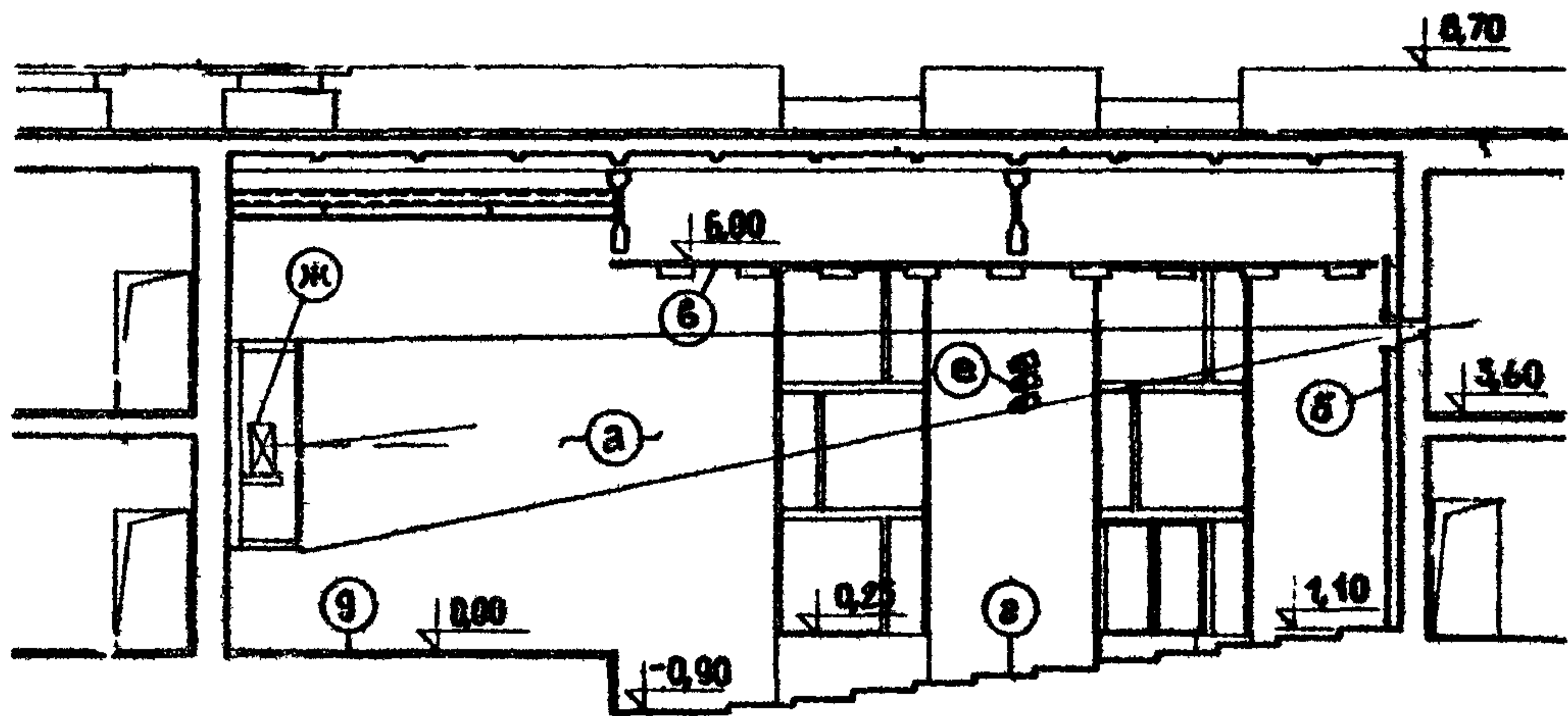
РАЗРЕЗ по А-А
